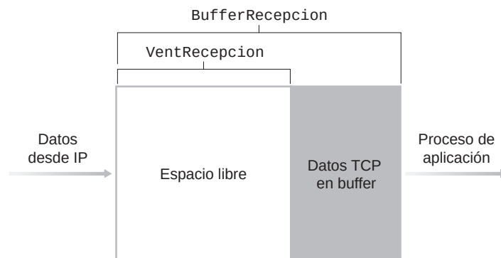
Figura 3.38 ♦ La ventana de recepción ( VentRecepcion ) y el buffer de recepción ( BufferRecepcion ).
