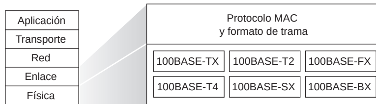
Figura 6.21 ♦ Estándares Ethernet a 100 Mbps: una capa de enlace común y diferentes capas físicas.
