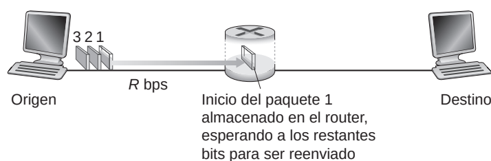
Figura 1.11 ♦ Conmutación de paquetes con almacenamiento y reenvío.
