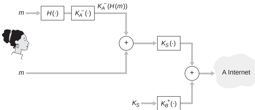
Figura 8.21 ♦ Alicia utiliza la criptografía de clave simétrica, la criptografía de clave pública, una función hash y una firma digital para obtener los servicios de confidencialidad, autenticación del emisor e integridad de los mensajes.
