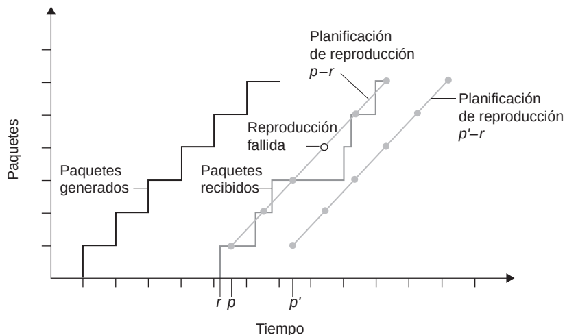
Figura 9.4 ♦ Pérdida de paquetes para diferentes retardos fijos de reproducción.
