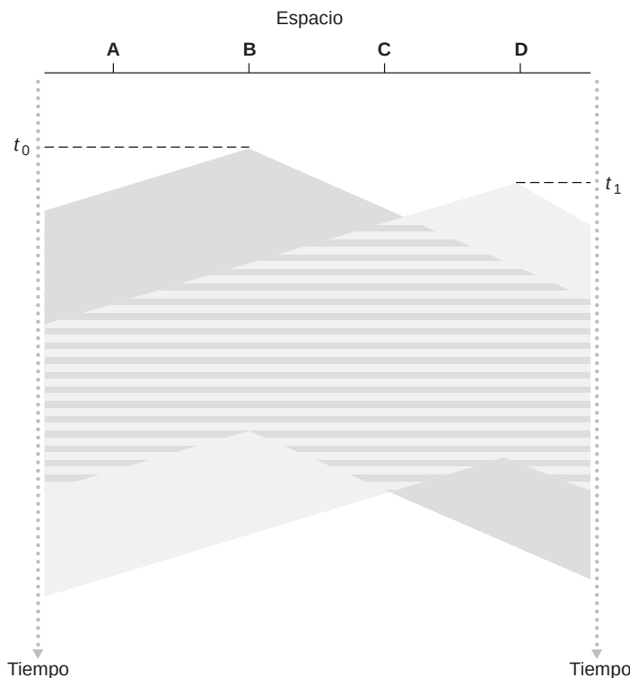
Figura 6.12 ♦ Diagrama espacio-tiempo para dos nodos CSMA con transmisiones que entran en colisión.
