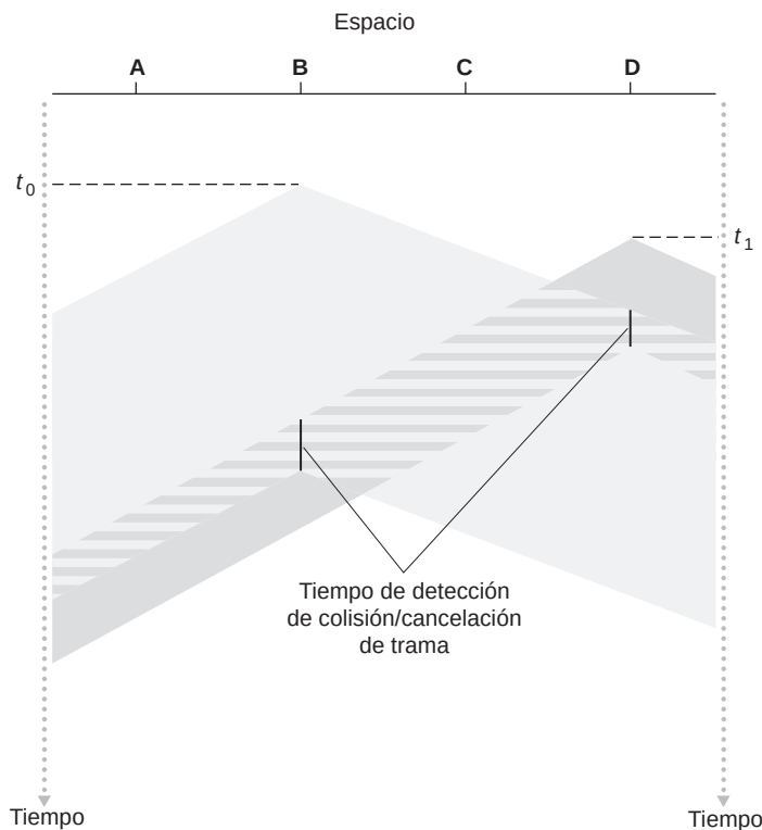
Figura 6.13 ♦ CSMA con detección de colisiones.
