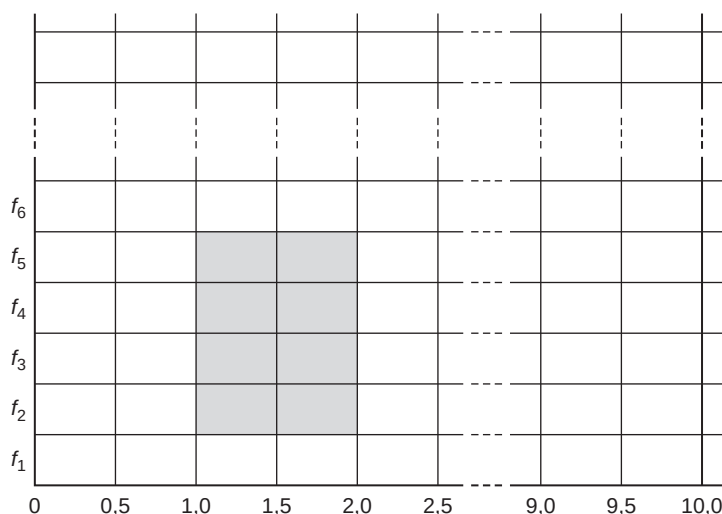
Figura 7.21 ♦ Veinte particiones de 0,5 ms organizadas en tramas de 10 ms en cada frecuencia. Se indica sombreada una asignación de ocho particiones.
