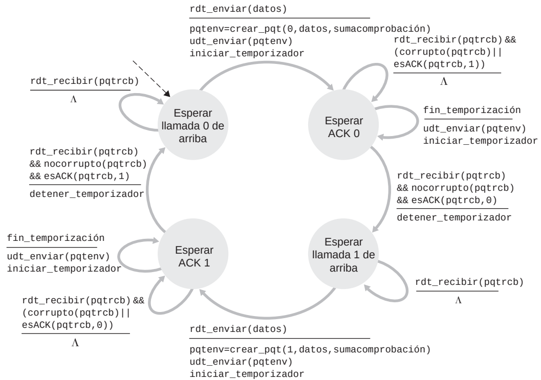
Figura 3.15 ♦ Lado emisor de rdt3.0
