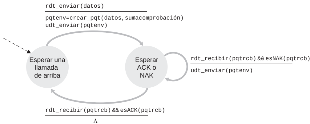
a. rdt2.0: lado emisor
