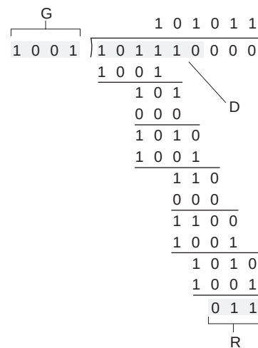
Figura 6.7 ♦ Un ejemplo de cálculo de CRC.
