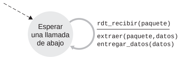
Figura 3.9 ♦ rdt1.0 – Protocolo para un canal totalmente fiable.
