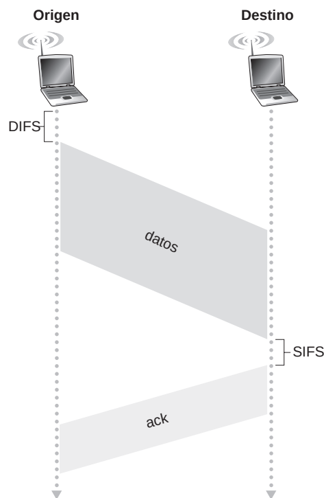
Figura 7.10 ♦ 802.11 utiliza reconocimientos (ACK) de la capa de enlace.
