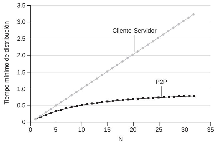
Figura 2.23 ♦ Tiempo de distribución para las arquitecturas P2P y cliente-servidor.
