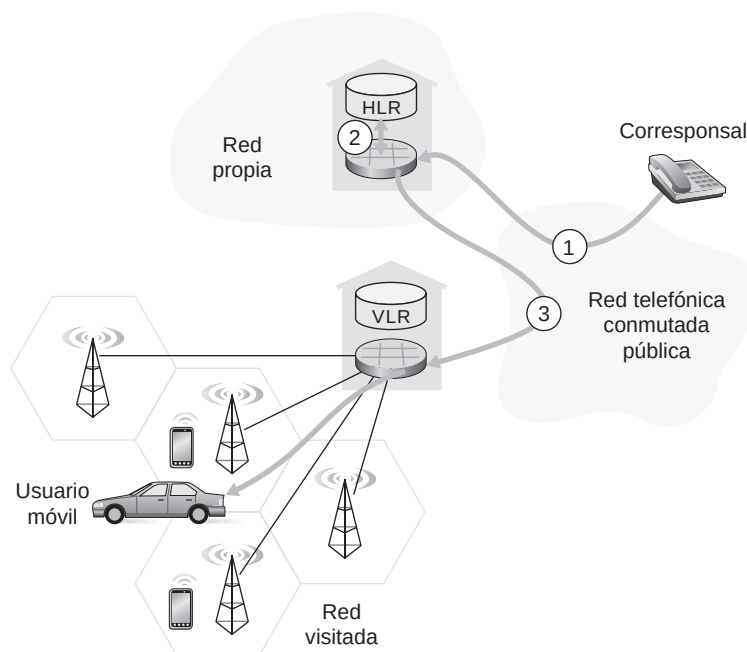
Figura 7.30 ♦ Establecimiento de una llamada hacia un usuario móvil: enrutamiento indirecto.
