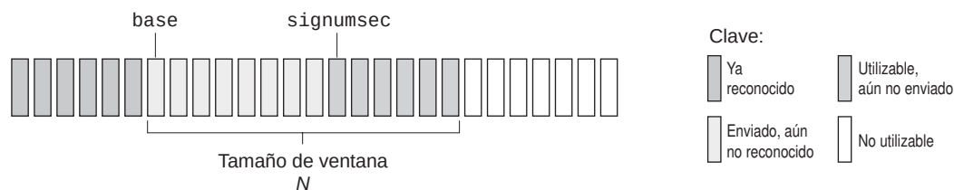
Figura 3.19 ♦ Números de secuencia en el emisor en el protocolo Retroceder N.
