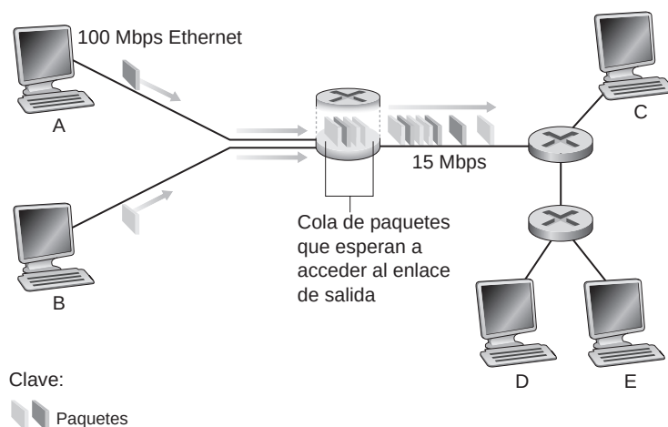
Figura 1.12 ♦ Conmutación de paquetes.
