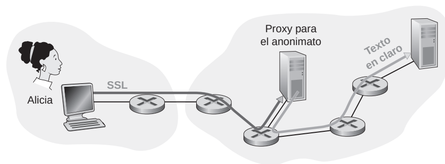
Figura 8.35 ♦ Cómo proporcionar anonimato y privacidad con un proxy.
