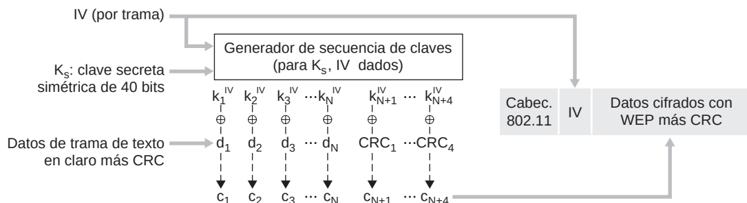
Figura 8.30 ♦ Protocolo WEP 802.11.
