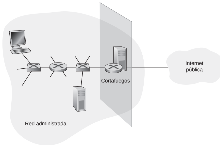
Figura 8.33 ♦ Colocación de un cortafuegos entre la red administrada y el mundo exterior.
