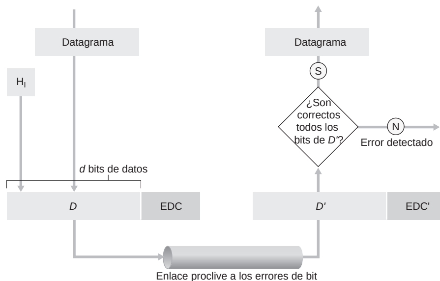
Figura 6.3 ♦ Escenario para la detección y corrección de errores.
