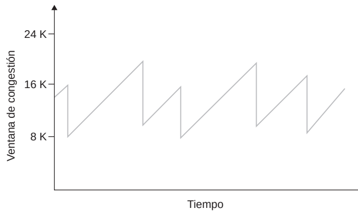
Figura 3.53 ♦ Control de congestión con crecimiento aditivo y decrecimiento multiplicativo.
