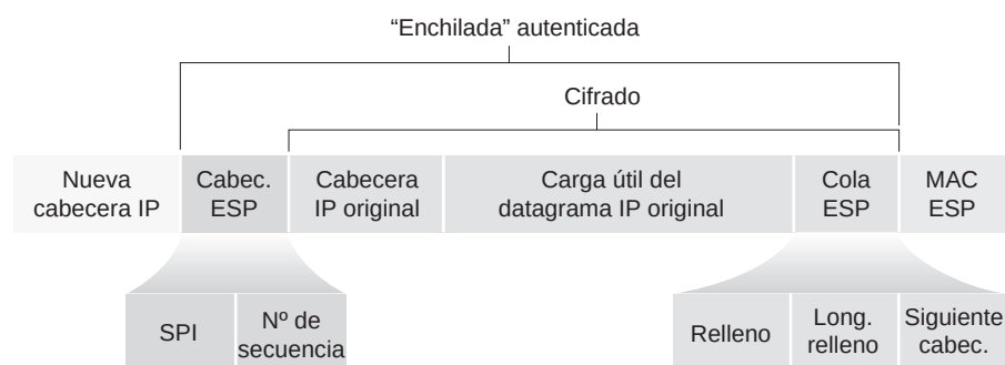
Figura 8.29 ♦ Formato del datagrama IPsec.
