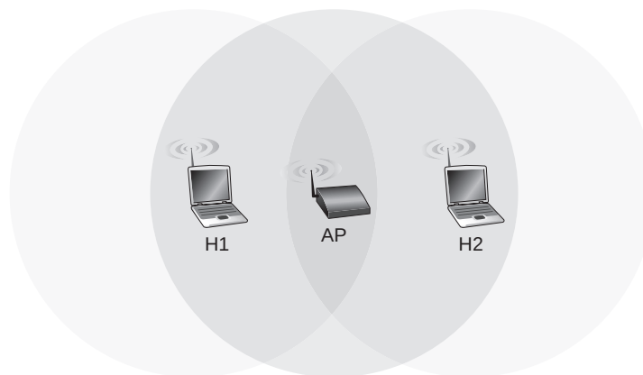
Figura 7.11 ♦ Ejemplo de terminales ocultos: H1 está oculto a ojos de H2 y viceversa.
