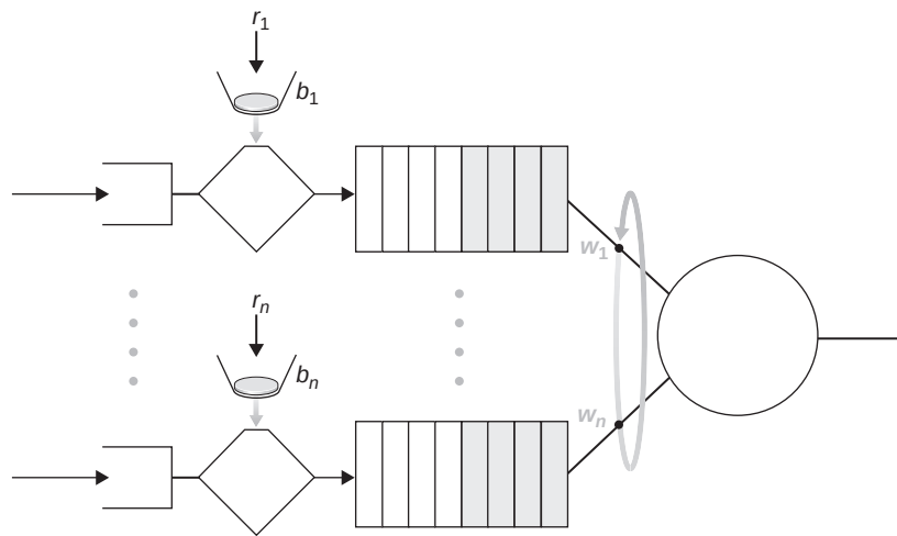
Figura 9.15 ♦ n flujos multiplexados con cubetas con pérdidas y planificación WFQ.
