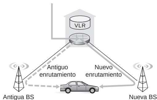
Figura 7.31 ♦ Escenario de transferencia de llamadas entre estaciones base con un MSC común.
