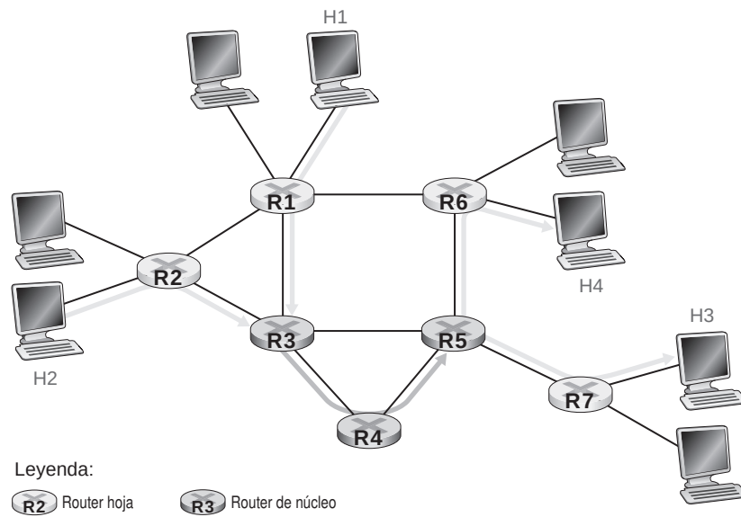
Figura 9.16 ♦ Un ejemplo de red Diffserv simple.
