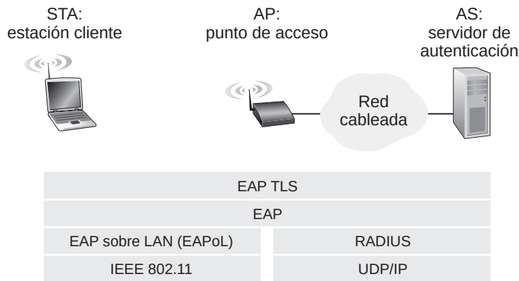
Figura 8.32 ♦ EAP es un protocolo extremo a extremo. Los mensajes EAP se encapsulan utilizando EAPoL sobre el enlace inalámbrico existente entre el cliente y el punto de acceso, y empleando RADIUS sobre UDP/IP entre el punto de acceso y el servidor de autenticación.
