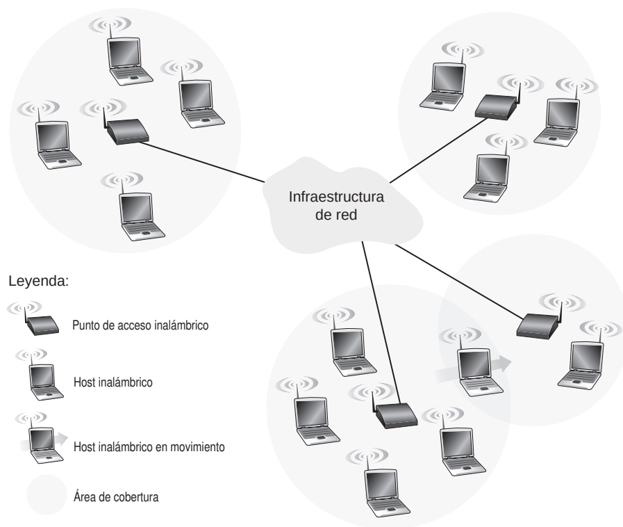
Figura 7.1 ♦ Elementos de una red inalámbrica.
