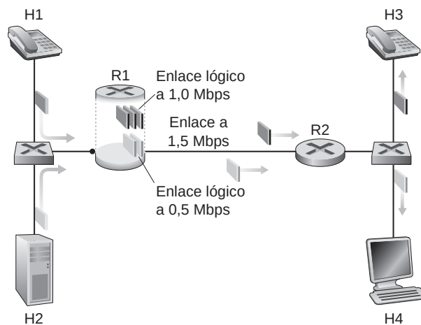
Figura 9.13 ♦ Aislamiento lógico de las clases de tráfico de audio y HTTP.
