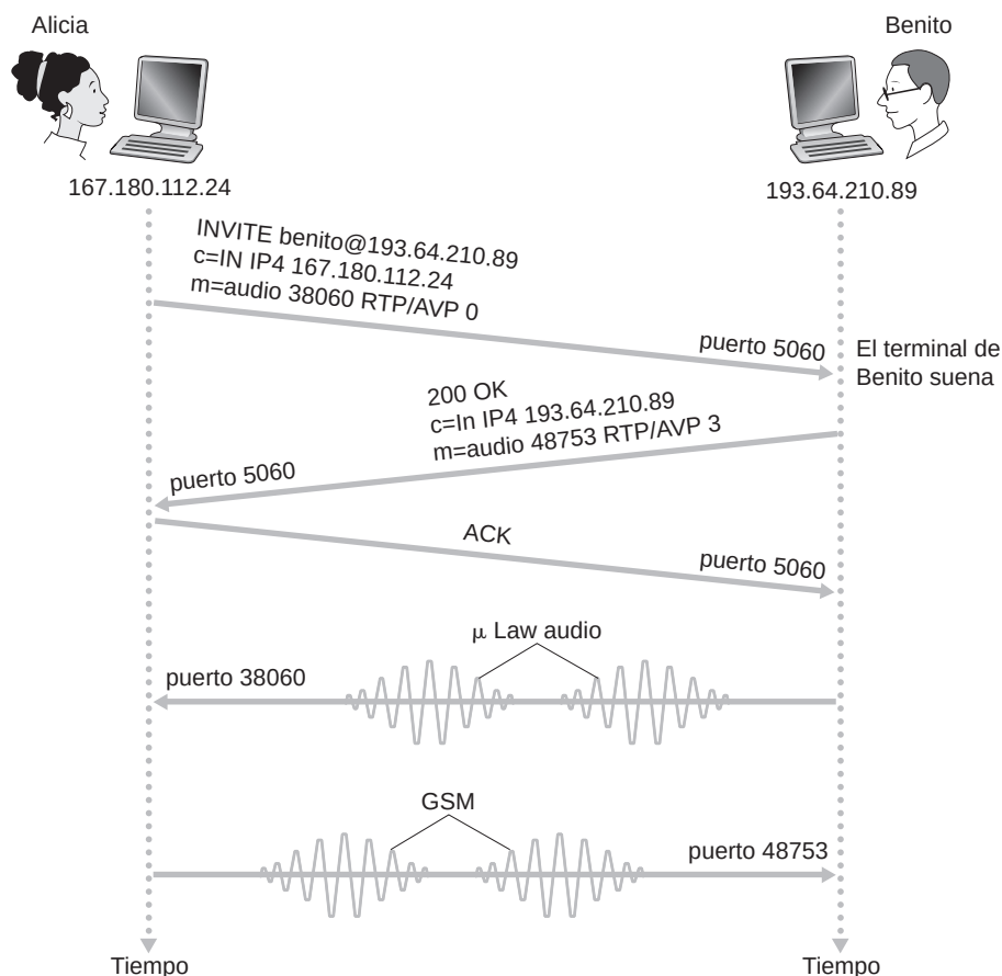
Figura 9.9 ♦ Establecimiento de una llamada SIP cuando Alicia conoce la dirección IP de Benito.
