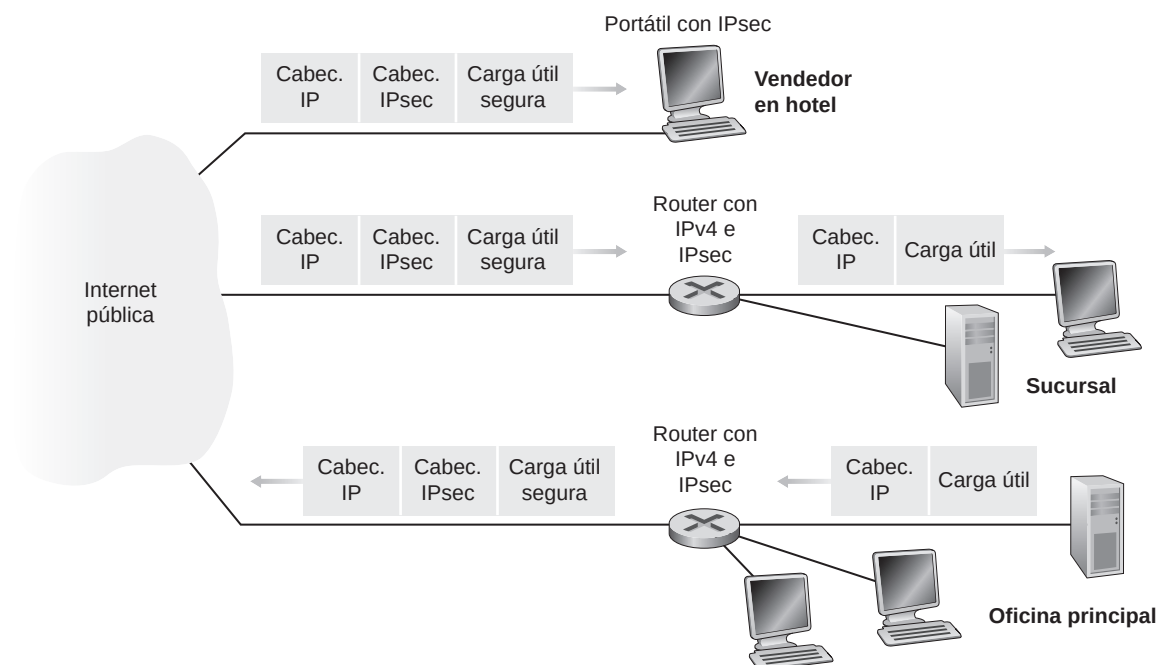
Figura 8.27 ♦ Red privada virtual (VPN).
