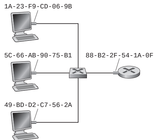
Figura 6.16 ♦ Cada interfaz conectada a una LAN dispone de una dirección MAC única.
