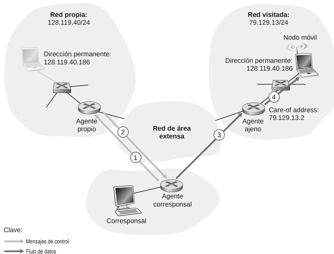
Figura 7.26 ♦ Enrutamiento directo hacia un usuario móvil.
