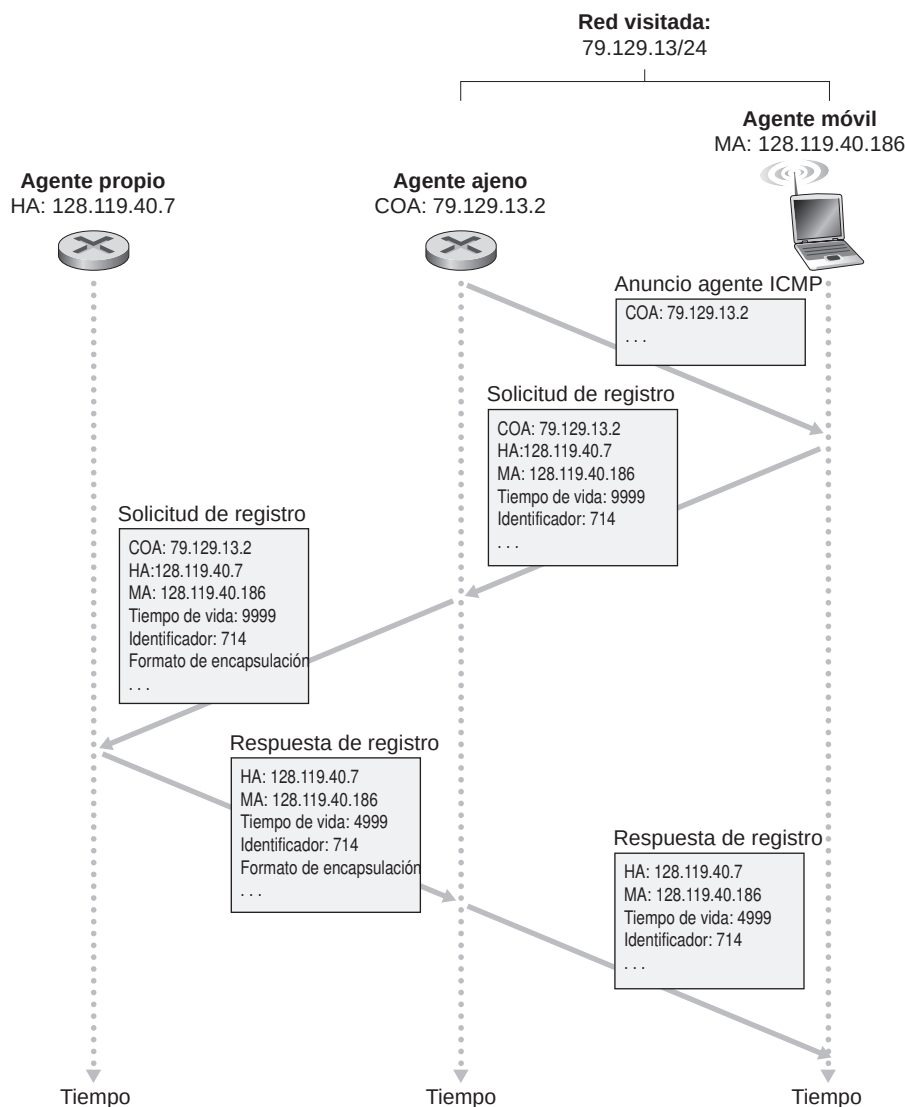
Figura 7.29 ♦ Anuncio de agente y registro de IP móvil.
