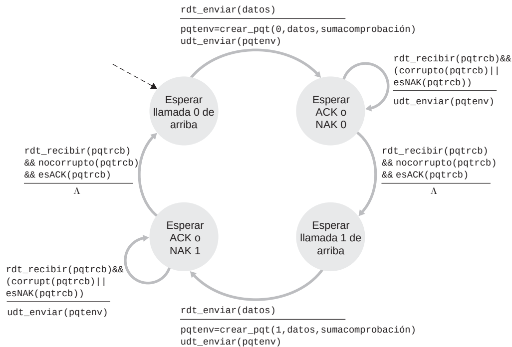
Figura 3.11 ♦ Lado emisor de rdt2.1
