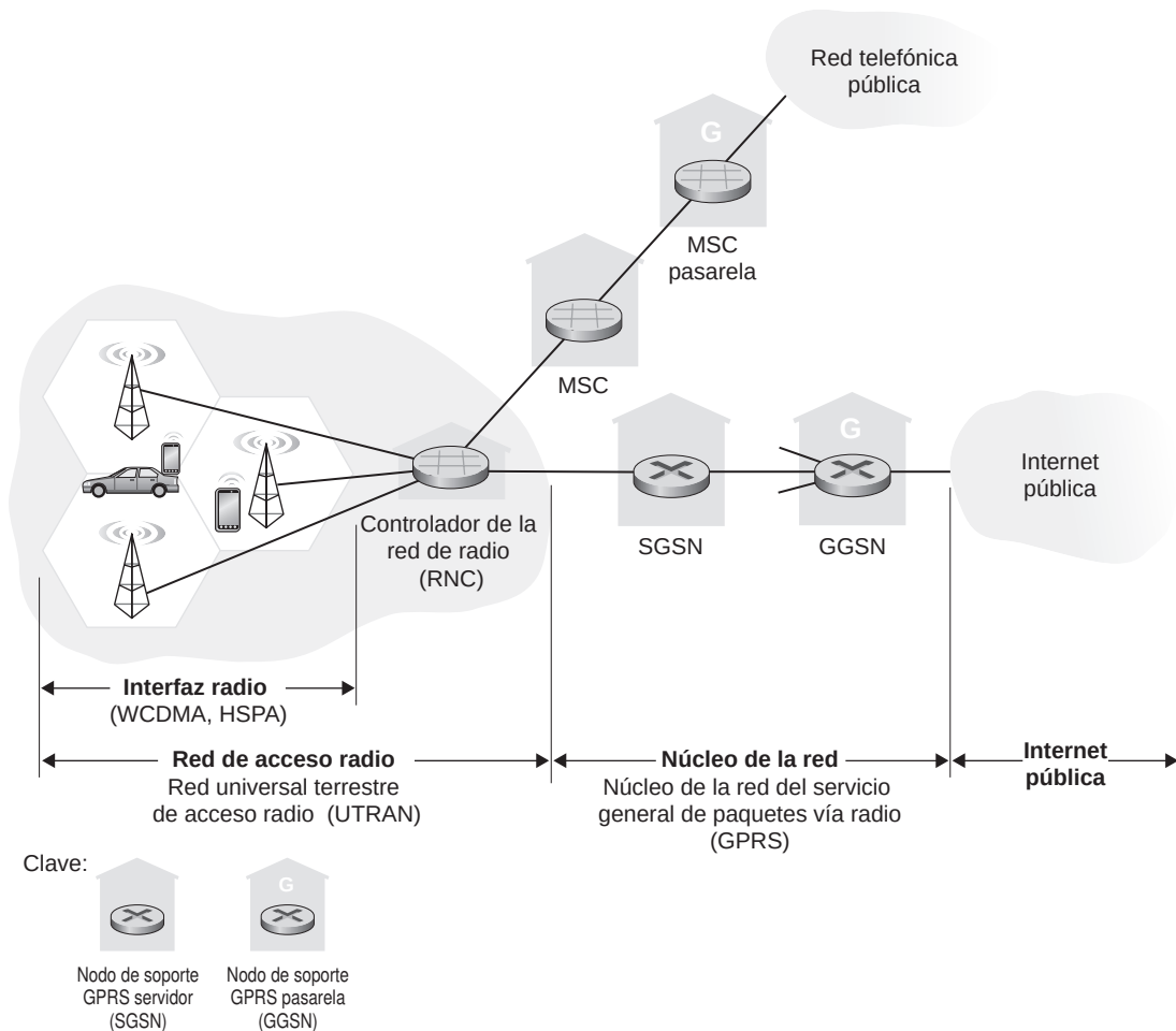
Figura 7.19 ♦ Arquitectura del sistema 3G.
