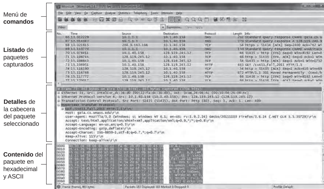
Figura 1.28 ♦ Una captura de pantalla de Wireshark (reimpresa con permiso de Wireshark Foundation).
