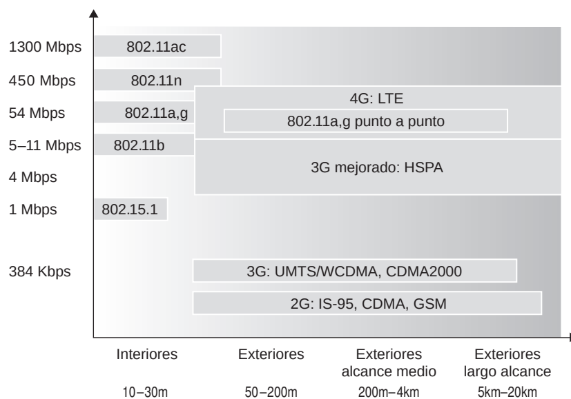
Figura 7.2 ♦ Características del enlace para una serie de estándares seleccionados de redes inalámbricas.
