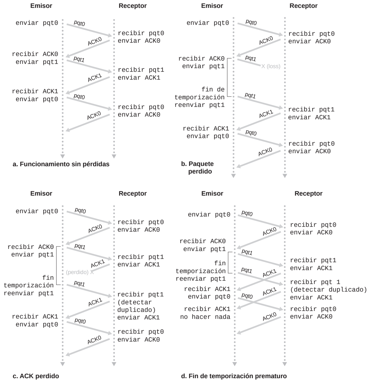
Figura 3.16 ♦ Funcionamiento de rdt3.0, el protocolo de bit alternante.
