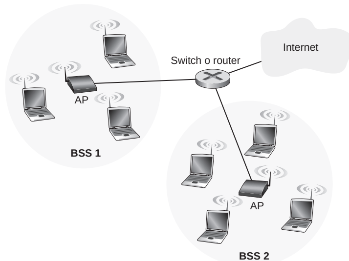
Figura 7.7 ♦ Arquitectura de una red LAN IEEE 802.11.
