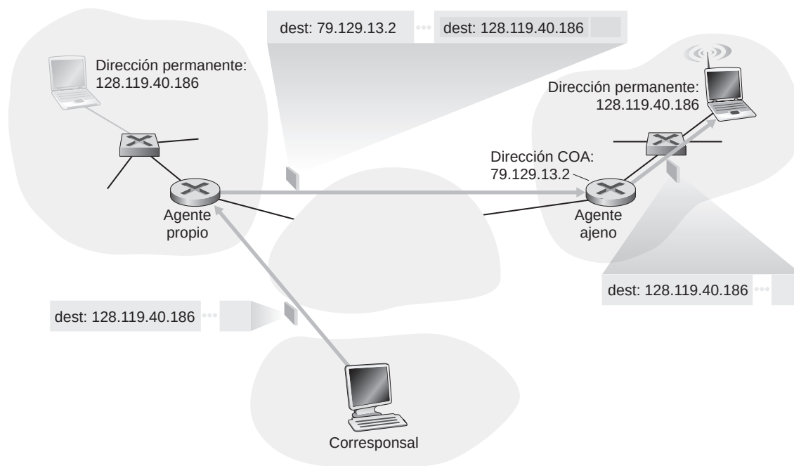
Figura 7.25 ♦ Encapsulación y desencapsulación.
