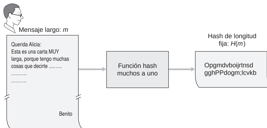
Figura 8.7 ♦ Funciones hash.
