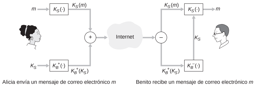
Figura 8.19 ♦ Alicia utiliza una clave de sesión simétrica, K_S , para enviar un mensaje secreto de correo electrónico a Benito.
