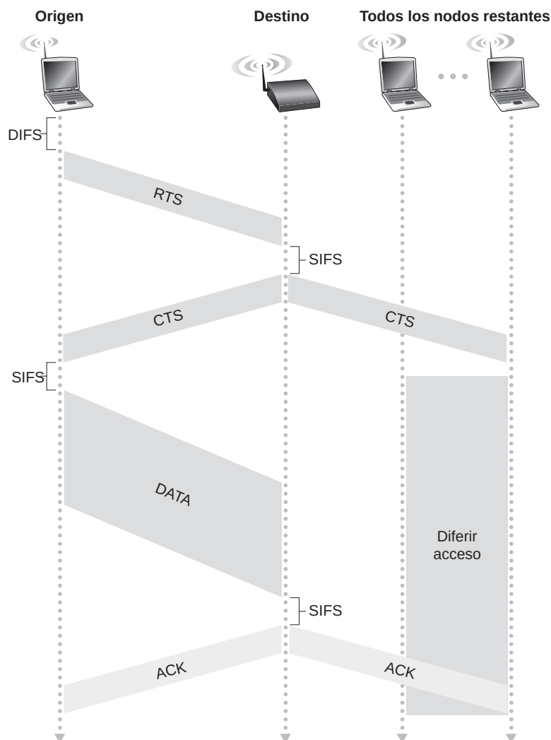
Figura 7.12 ♦ Evitación de colisiones utilizando las tramas RTS y CTS.
