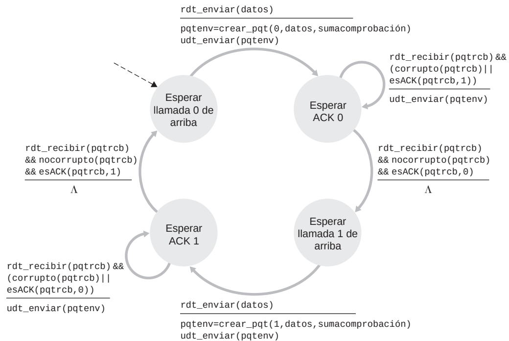
Figura 3.13 ♦ Lado emisor de rdt2.2.
