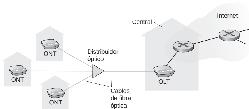
Figura 1.7 ♦ Acceso a Internet mediante FTTH.
