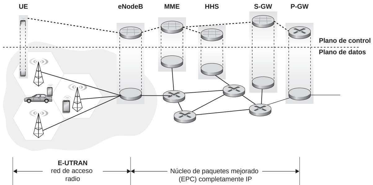
Figura 7.20 ♦ Arquitectura de red 4G.
