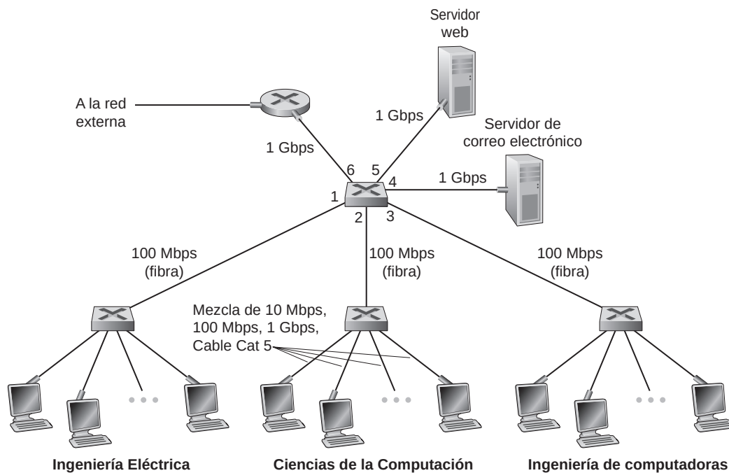
Figura 6.15 ♦ Red institucional conectada mediante cuatro switches.
