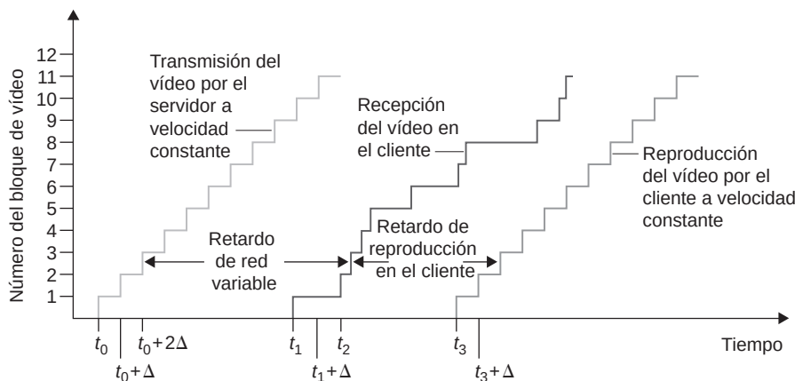
Figura 9.1 ♦ Retardo de reproducción de un flujo de vídeo en el cliente.
