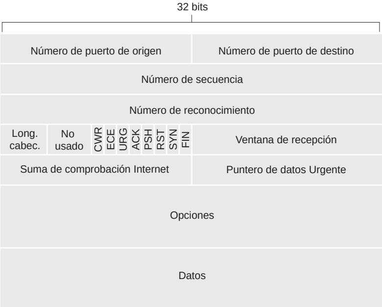
Figura 3.29 ♦ Estructura del segmento TCP.
