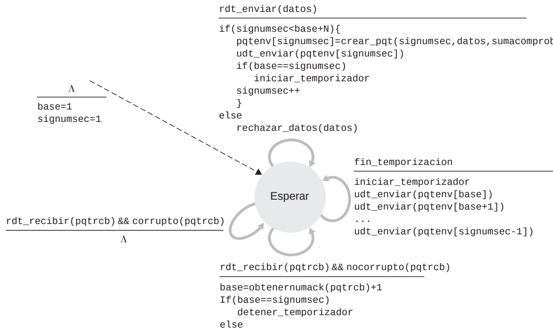
Figura 3.20 ♦ Descripción de la FSM ampliada del lado emisor de GBN.
