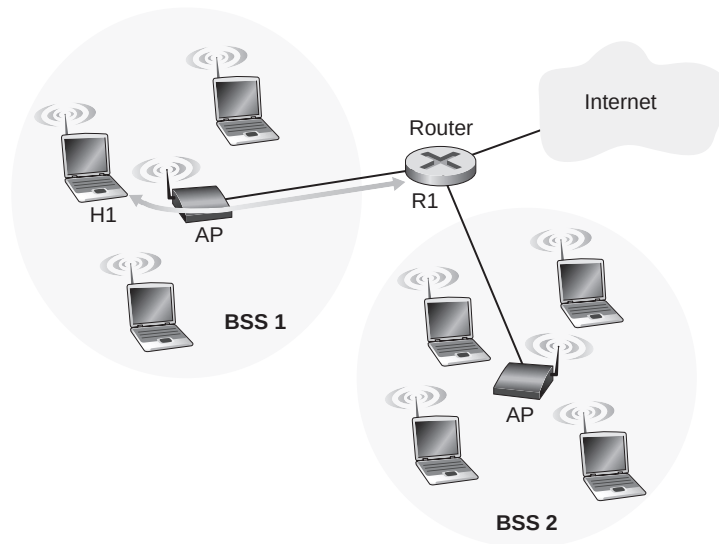
Figura 7.14 ♦ Uso de los campos de dirección en las tramas 802.11: envío de tramas entre H1 y R1.
