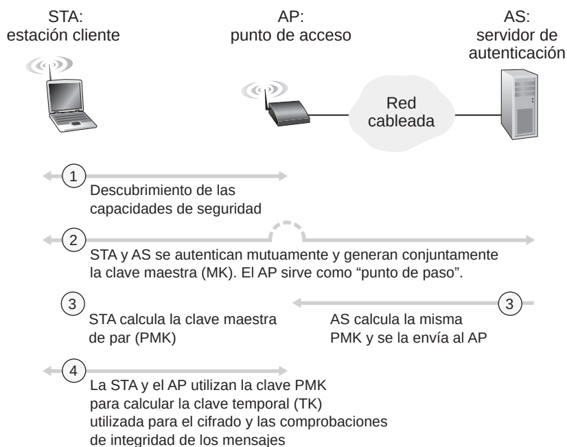
Figura 8.31 ♦ 802.11i: cuatro fases de operación.
