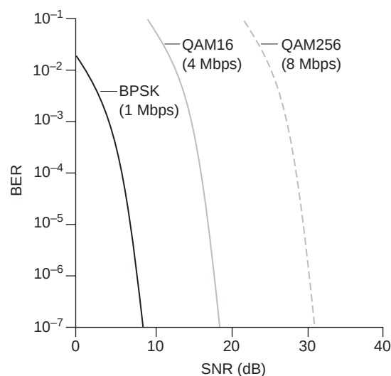
Figura 7.3 ♦ Tasa de errores de bit, velocidad de transmisión y SNR.
