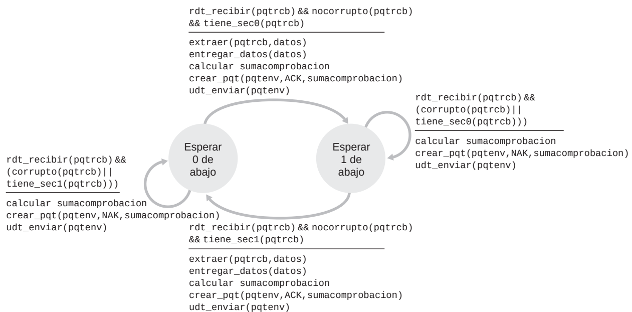
Figura 3.57 ♦ Un receptor incorrecto para el protocolo rdt 2.1.
