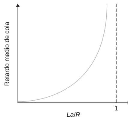
Figura 1.18 ♦ Dependencia del retardo medio de cola con respecto a la intensidad de tráfico.
