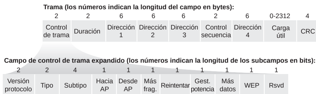
Figura 7.13 ♦ La trama 802.11.
