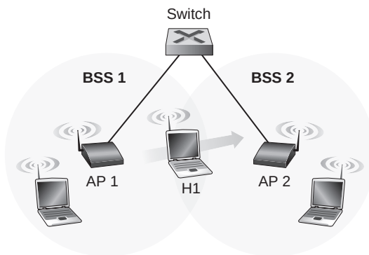
Figura 7.15 ♦ Movilidad dentro de la misma subred.
