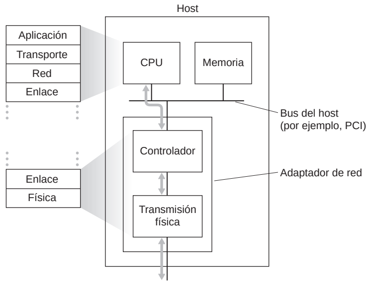
Figura 6.2 ♦ Adaptador de red: su relación con otros componentes del host y con la funcionalidad de la pila de protocolos.
