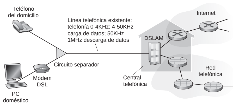
Figura 1.5 ♦ Acceso a Internet mediante DSL.
