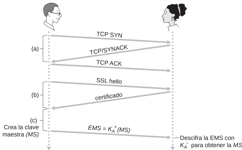
Figura 8.25 ♦ La fase de acuerdo de casi-SSL comienza con una conexión TCP.
