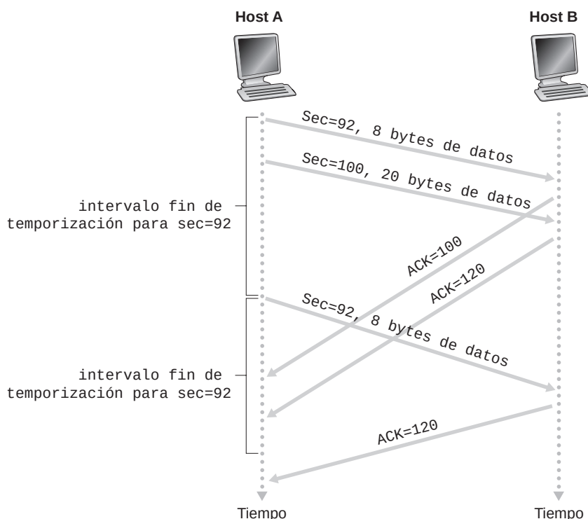
Figura 3.35 ♦ Segmento 100 no retransmitido.
