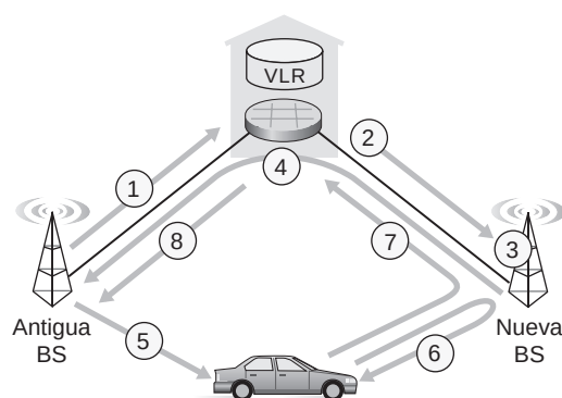
Figura 7.32 ♦ Pasos necesarios para realizar una transferencia entre estaciones base con un MSC común.
