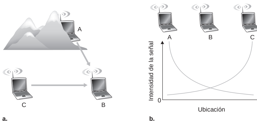
Figura 7.4 ♦ Problema del terminal oculto causado por la existencia de un obstáculo (a) y problema del desvanecimiento (b).
