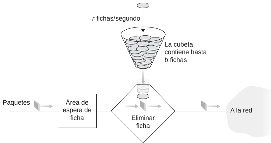
Figura 9.14 ♦ El controlador de la cubeta con pérdidas.
