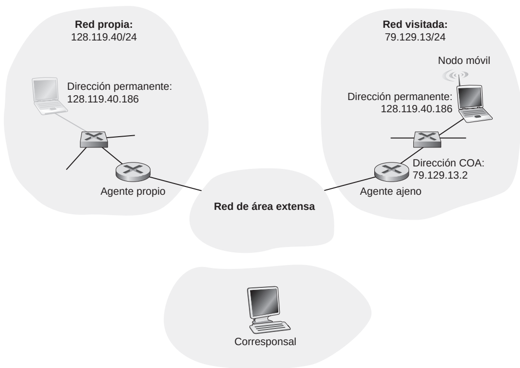
Figura 7.23 ♦ Elementos iniciales de una arquitectura de red móvil.
