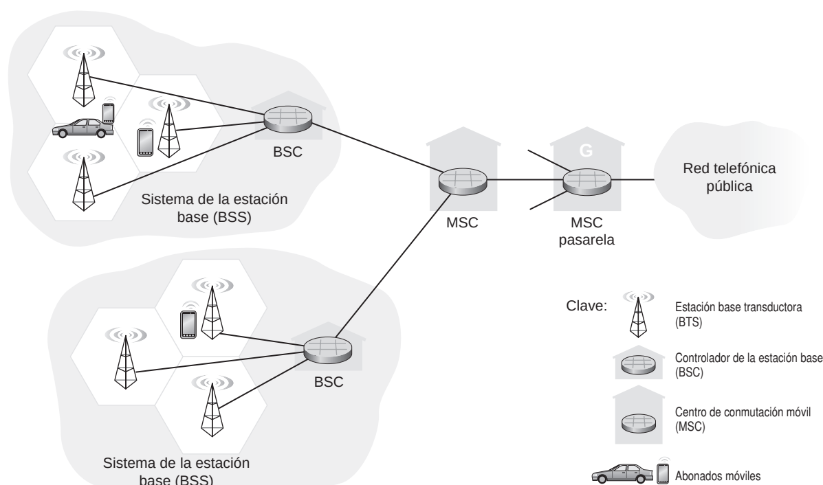
Figura 7.18 ♦ Componentes de una arquitectura de red celular GSM 2G.
