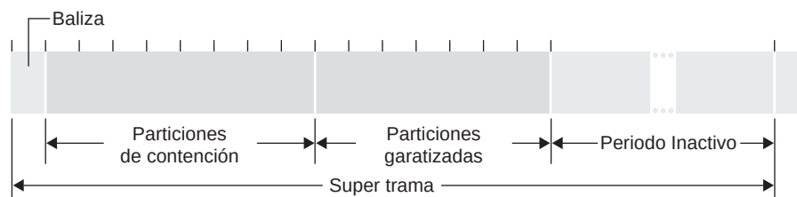
Figura 7.17 ♦ Estructura de la supertrama de Zigbee 802.15.4.
