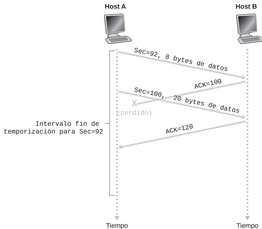
Figura 3.36 ♦ Un reconocimiento acumulativo evita la retransmisión del primer segmento.
