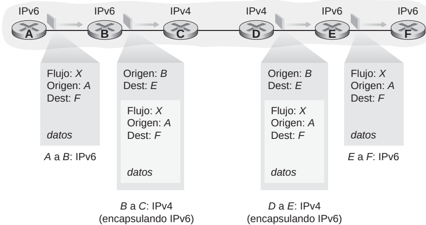
Figura 4.27 ♦ Tunelización.
