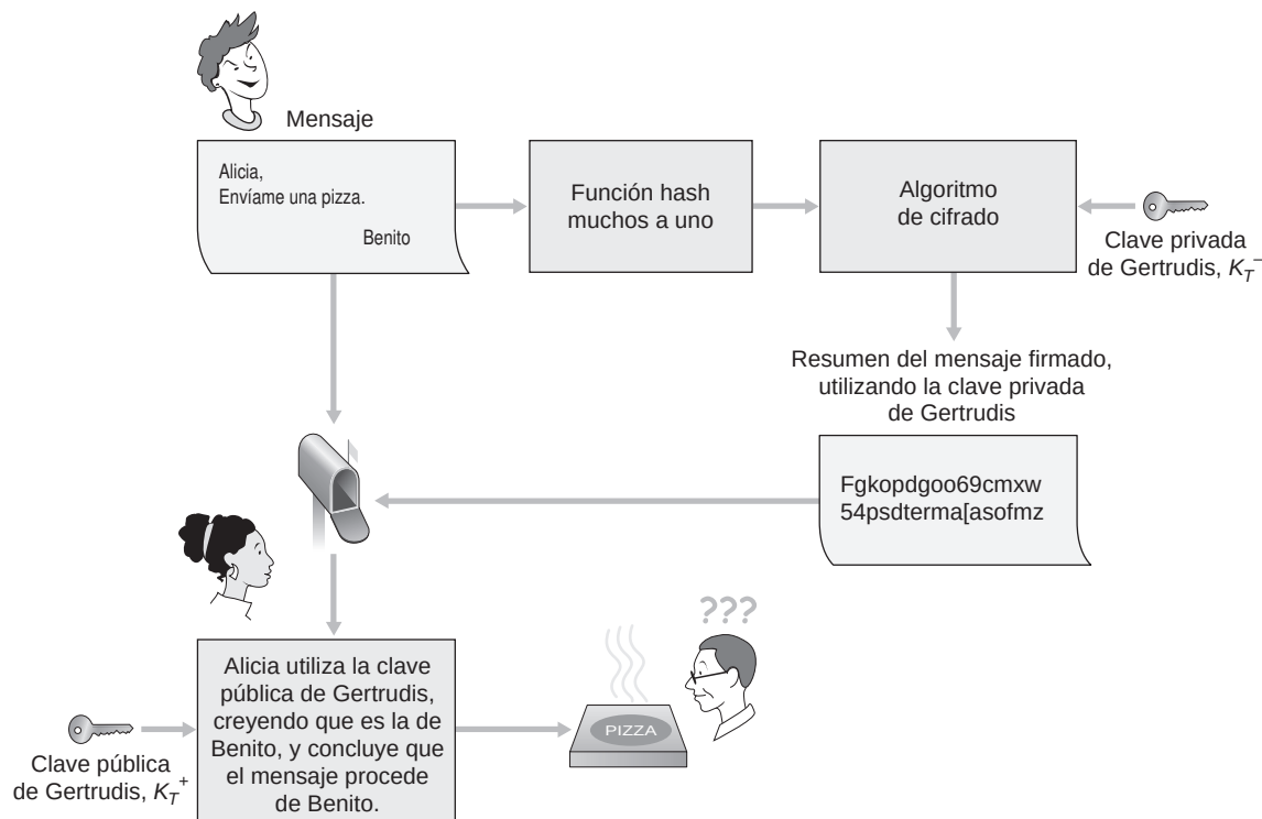
Figura 8.13 ♦ Gertrudis se hace pasar por Benito usando criptografía de clave pública.
