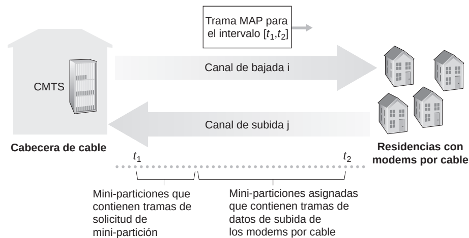
Figura 6.14 ♦ Canales de subida y de bajada entre el CMTS y los módems por cable.
