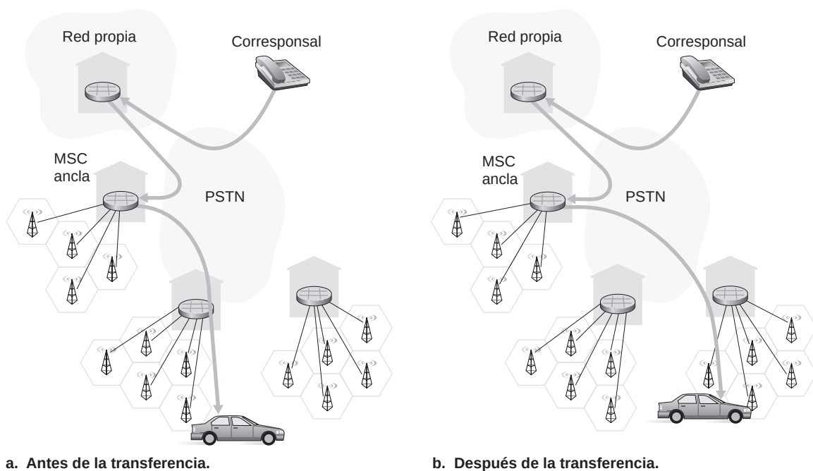
Figura 7.33 ♦ Re-enrutamiento a través de un MSC ancla.
