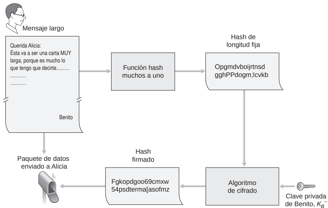
Figura 8.11 ♦ Transmisión de un mensaje firmado digitalmente.
