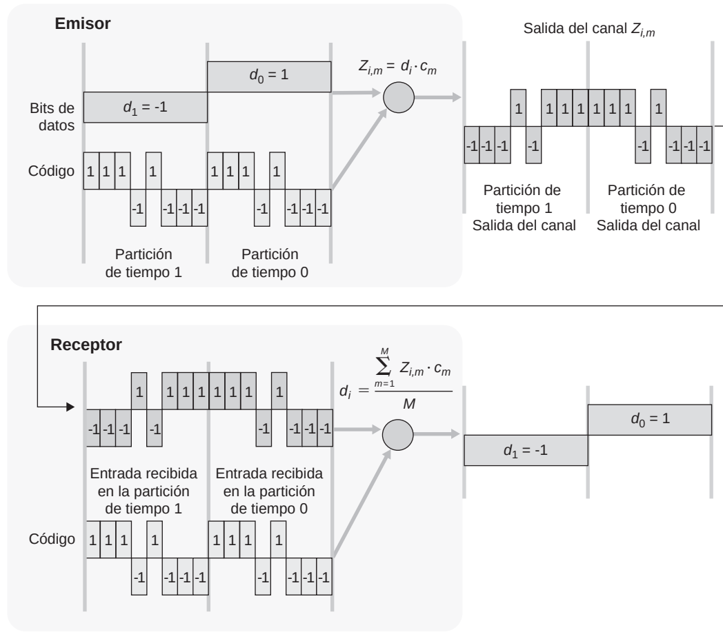
Figura 7.5 ♦ Un ejemplo simple de CDMA: codificación del emisor y decodificación del receptor.
