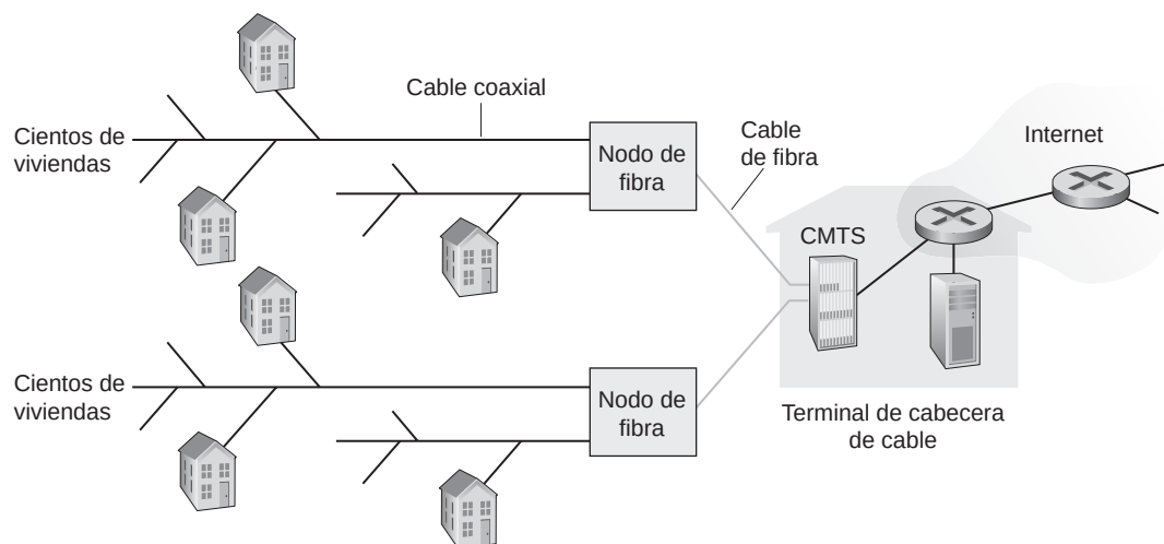
Figura 1.6 ♦ Red de acceso híbrida de fibra óptica y cable coaxial.
