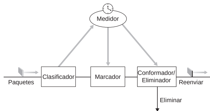
Figura 9.17 ♦ Visión lógica de las funciones de clasificación de paquetes y acondicionamiento de tráfico en el router terminal.
