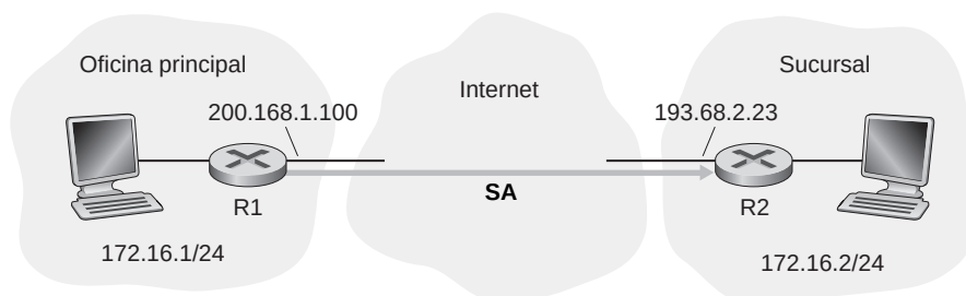
Figura 8.28 ♦ Asociación de seguridad (SA) de R1 a R2.
