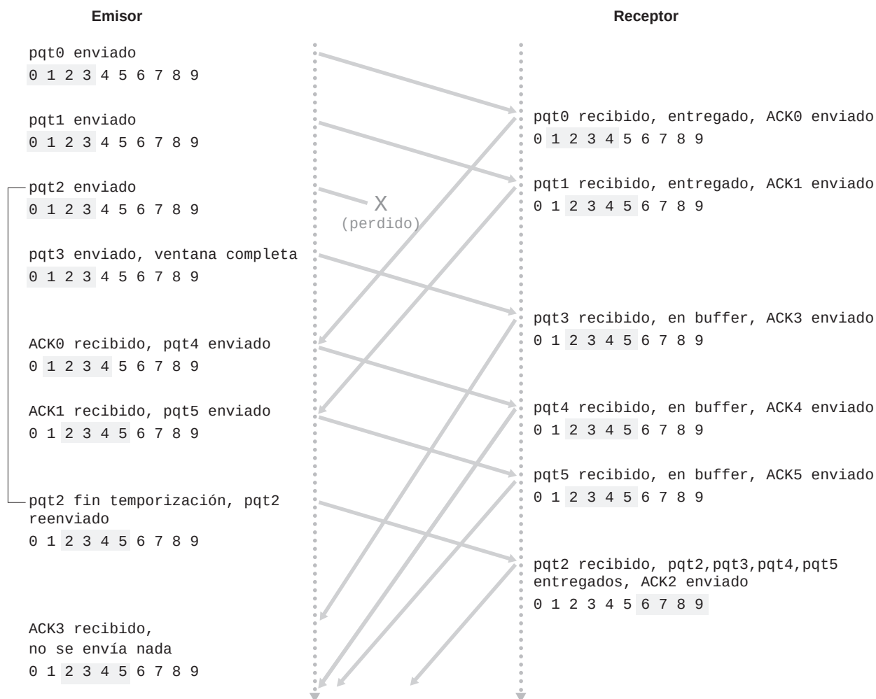
Figura 3.26 ♦ Funcionamiento del protocolo SR.
