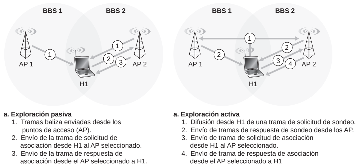
Figura 7.9 ♦ Exploración activa y pasiva de los puntos de acceso.
