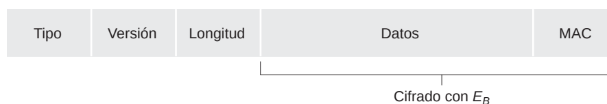
Figura 8.26 ♦ Formato de registro para SSL.
