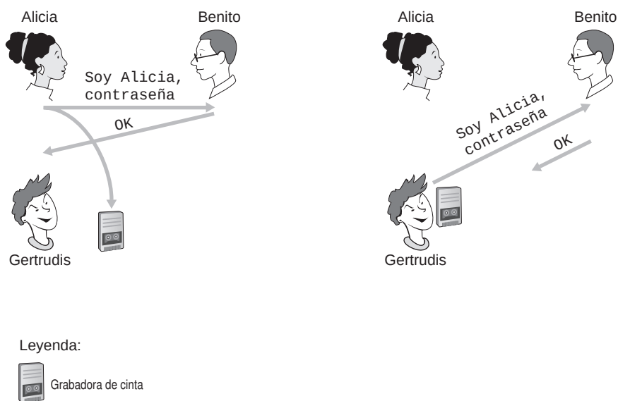
Figura 8.17 ♦ Protocolo ap3.0 y un posible escenario de fallo.
