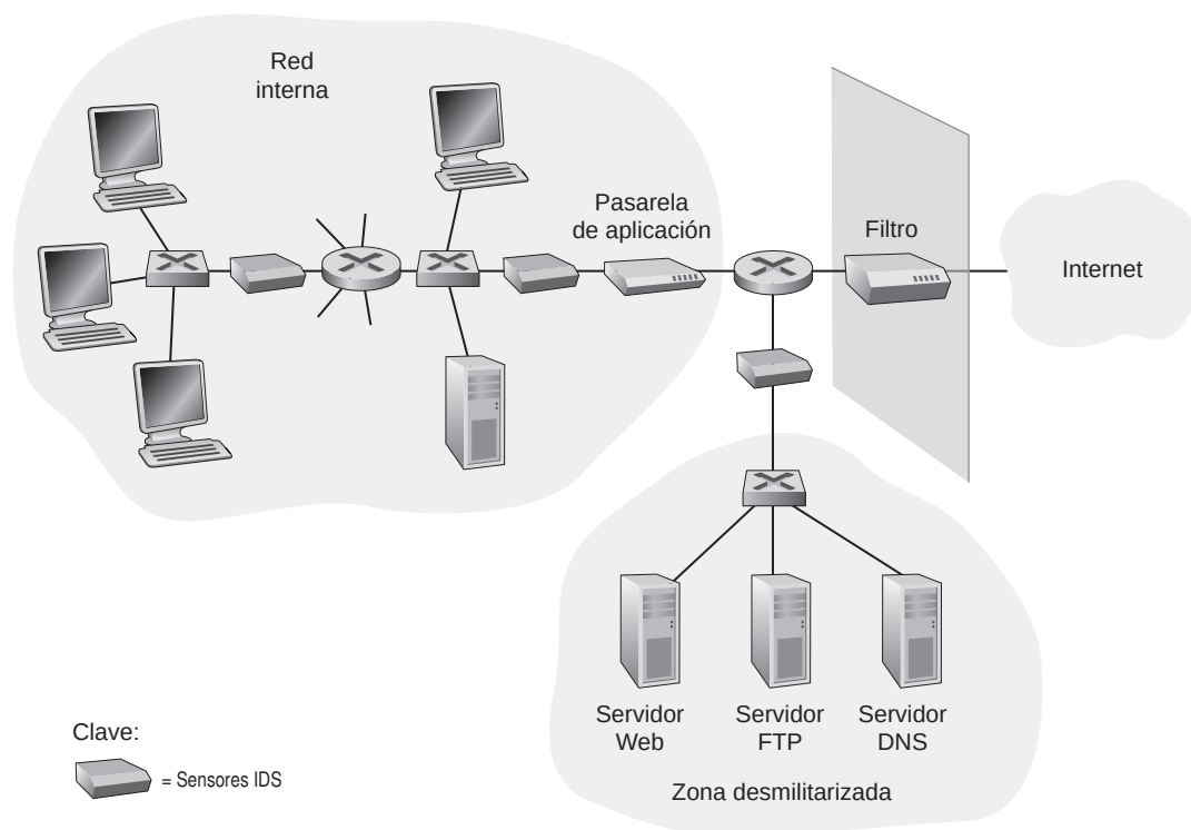
Figura 8.36 ♦ Una organización en la que se ha implantado un filtro, una pasarela de aplicación y sensores IDS.
