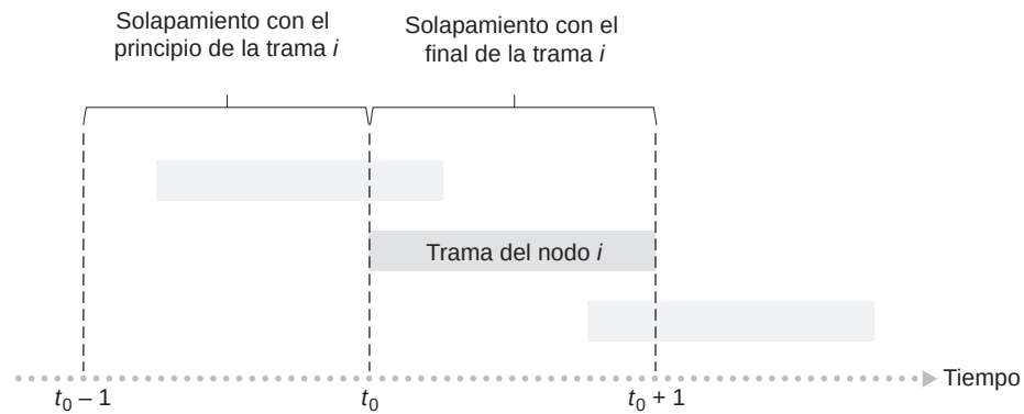
Figura 6.11 ♦ Transmisiones que interfieren en el protocolo ALOHA puro.
