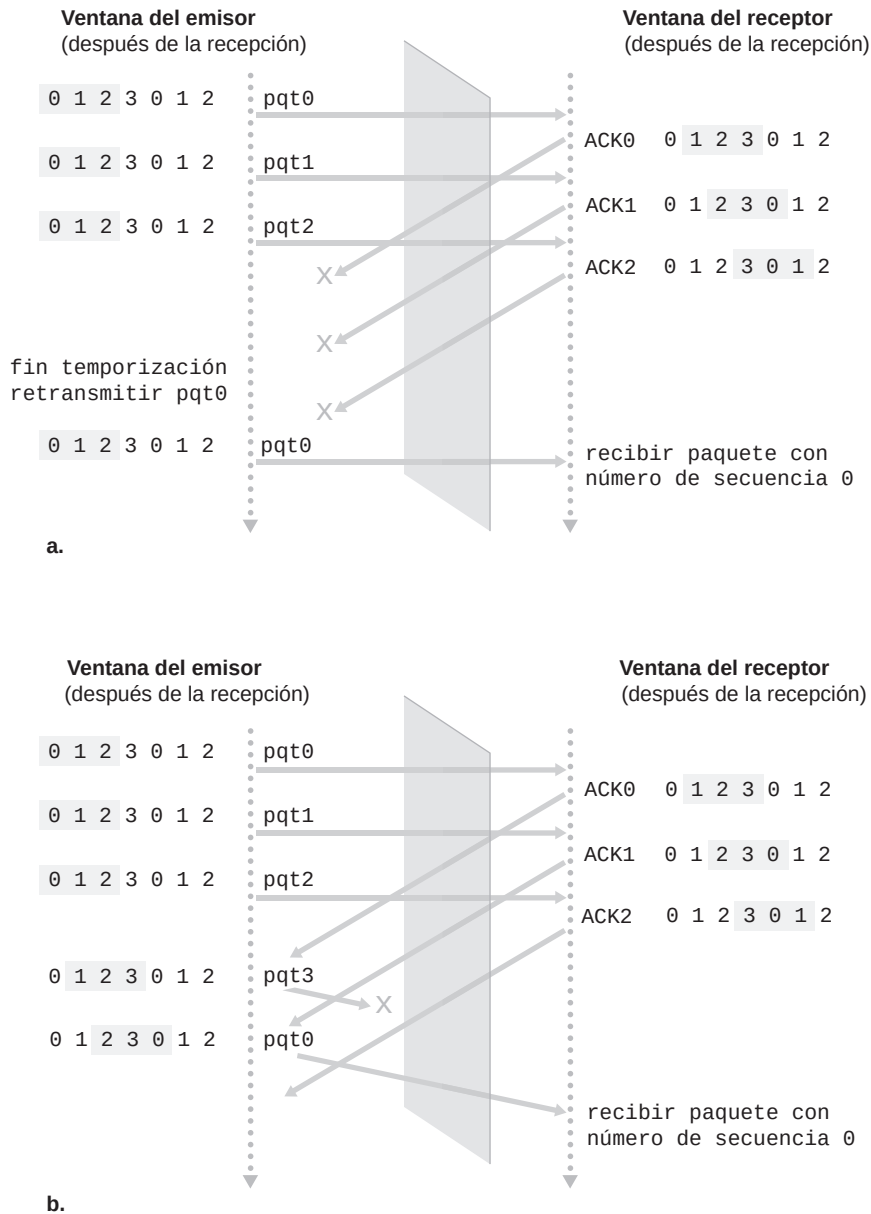
Figura 3.27 ♦ Dilema del receptor de los protocolos SR con ventanas demasiado grandes: ¿un nuevo paquete o una retransmisión?
