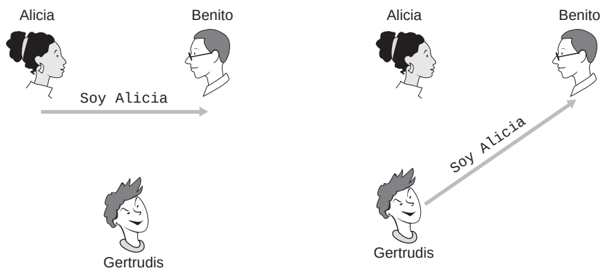
Figura 8.15 ♦ Protocolo ap1.0 y un posible escenario de fallo.
