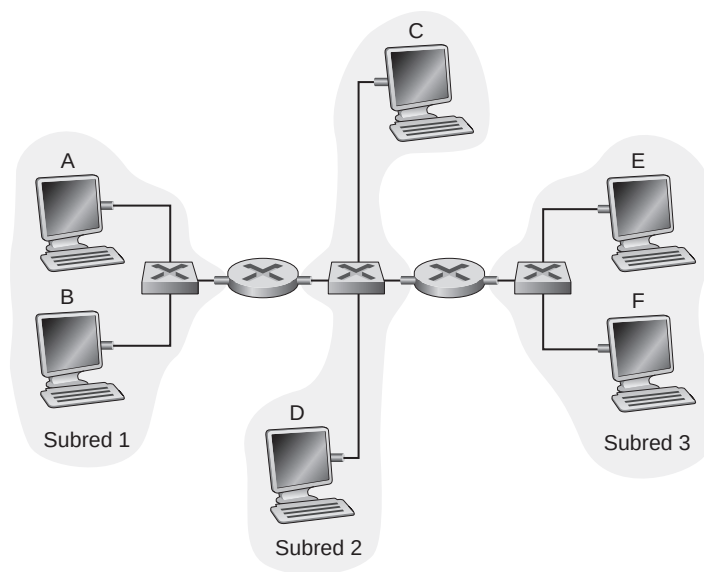
Figura 6.33 ♦ Tres subredes interconectadas mediante routers.
