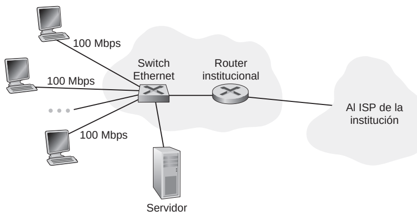
Figura 1.8 ♦ Acceso a Internet utilizando tecnología Ethernet.
