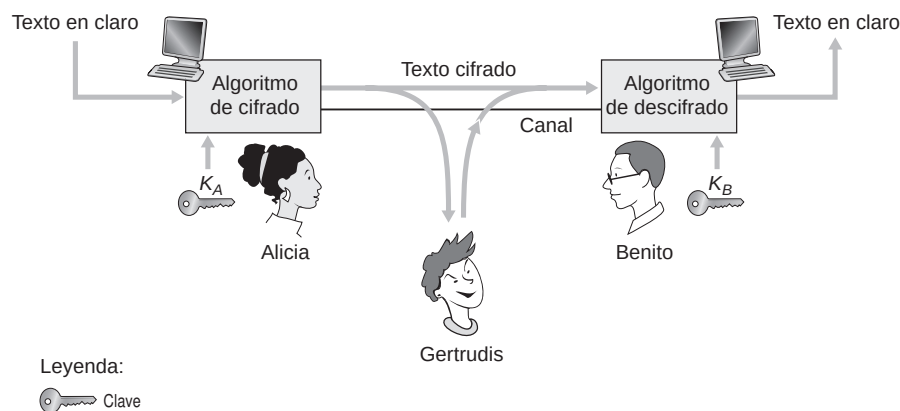
Figura 8.2 ♦ Componentes criptográficos.
