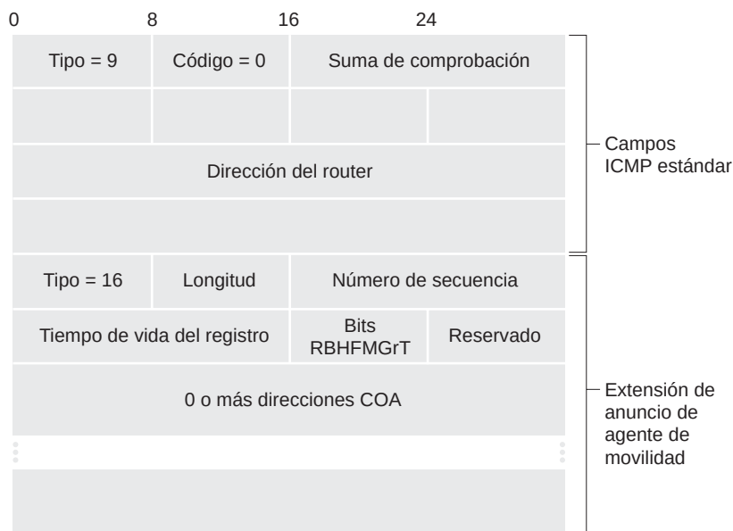
Figura 7.28 ♦ Mensaje de descubrimiento de router ICMP con la extensión de anuncio de agente de movilidad.
