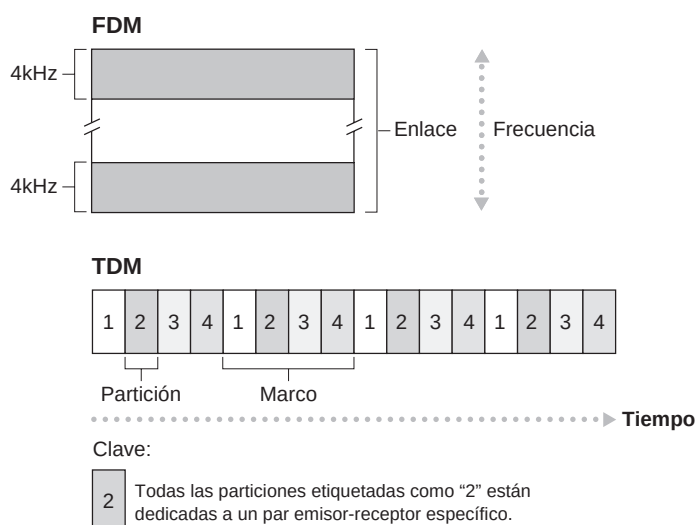
Figura 1.14 ♦ Con FDM, cada circuito obtiene de forma continua una fracción del ancho de banda. Con TDM, cada circuito dispone de todo el ancho de banda periódicamente durante breves intervalos de tiempo (es decir, durante las particiones).
