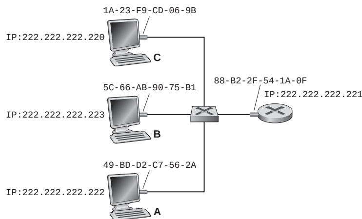
Figura 6.17 ♦ Cada interfaz de una LAN tiene una dirección IP y una dirección MAC.
