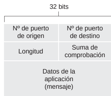
Figura 3.7 ♦ Estructura de un segmento UDP.
