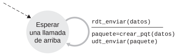
a. rdt1.0: lado emisor
