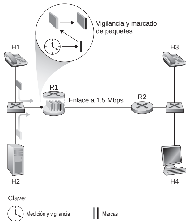
Figura 9.12 ♦ Vigilancia (y marcado) de las clases de tráfico de audio y HTTP.
