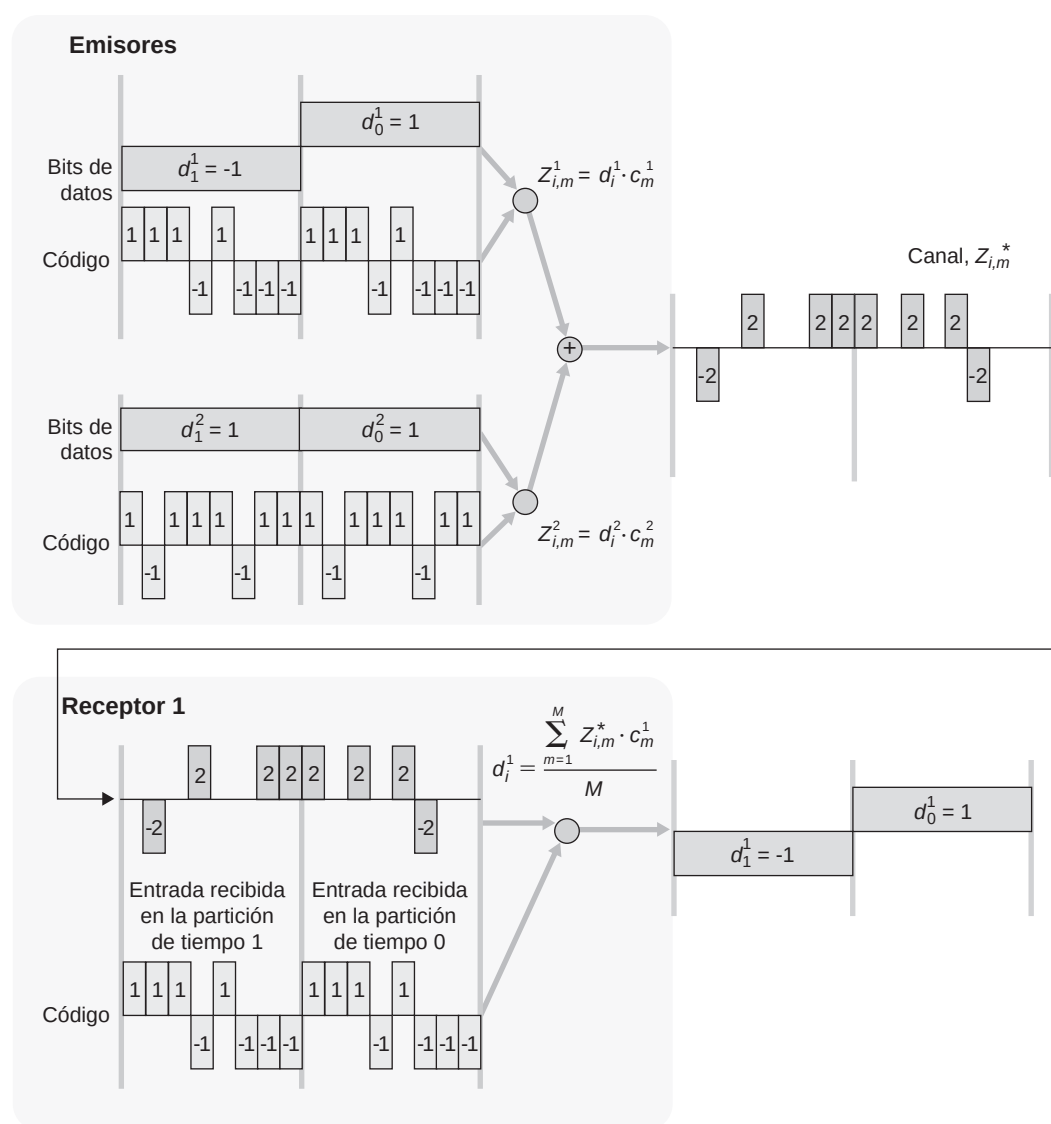
Figura 7.6 ♦ Un ejemplo de CDMA con dos emisores.
