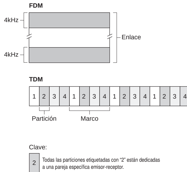
Figura 6.9 ♦ Un ejemplo de TDM y FDM para cuatro nodos.
