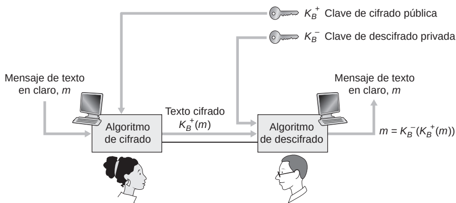
Figura 8.6 ♦ Criptografía de clave pública.
