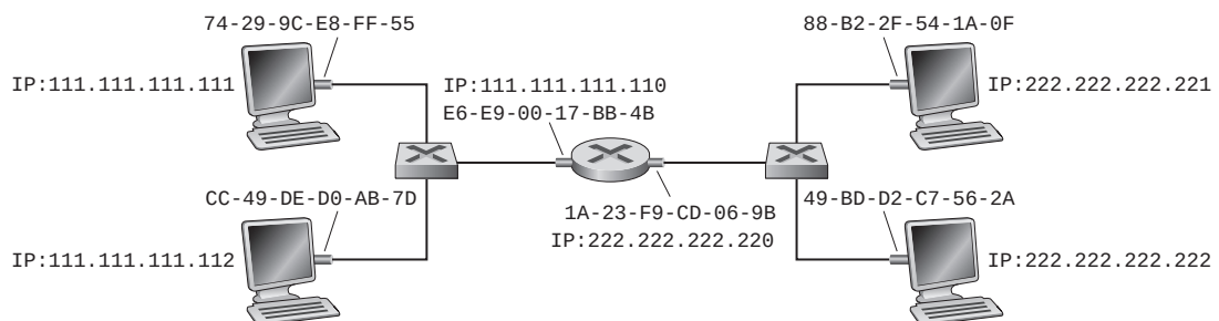
Figura 6.19 ♦ Dos subredes interconectadas mediante un router.
