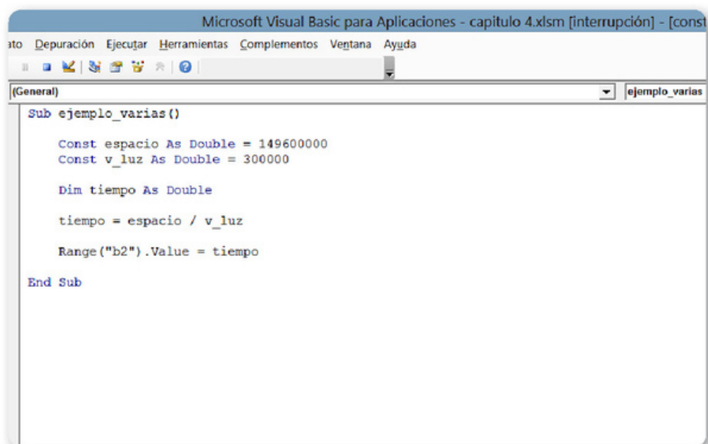
Figura 12. Los caracteres sufijos se pueden aplicar también a la declaración de variables, por ejemplo: espacio# .
