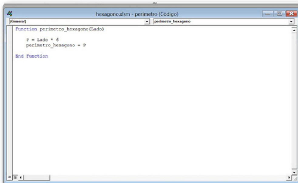
Figura 4. El código de esta función definida por el usuario devuelve el perímetro de un hexágono.
