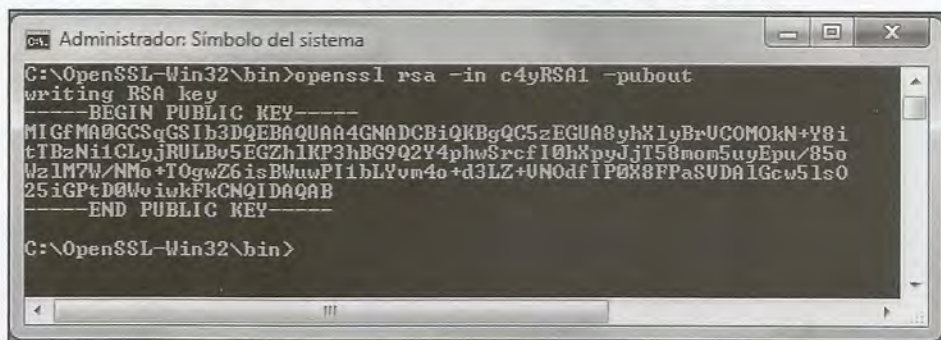
Figura 22. Exportación de la clave pública c4yRSA1 en formato base64.
