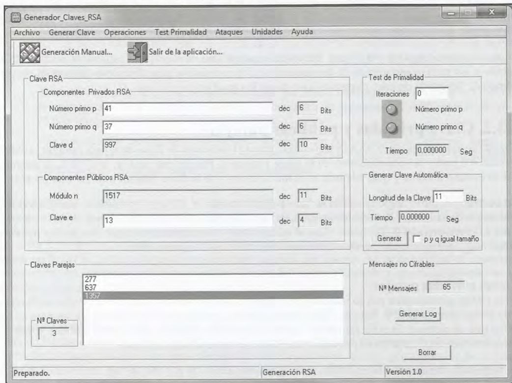
Figura 15. Las tres claves privadas parejas de la clave RSA.
