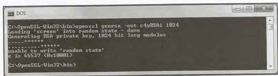
Figura 18. Generación de la clave c4yRSA1 de 1024 bits.
