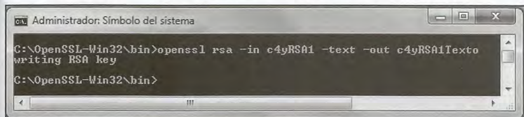
Figura 23. Conversión de la clave c4yRSA1 a formato hexadecimal.
