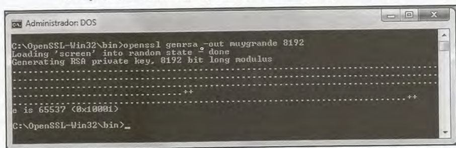
Figura 19. Generación de la clave muygrande de 8192 bits.
