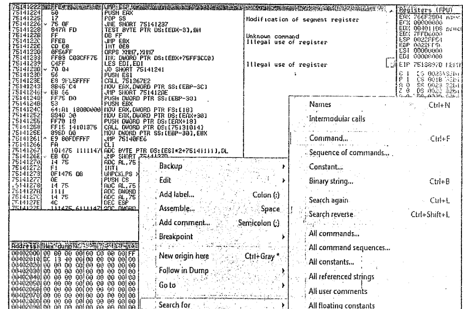
Fig 5.19: Localización de una instrucción de salto incondicional a la pila.
