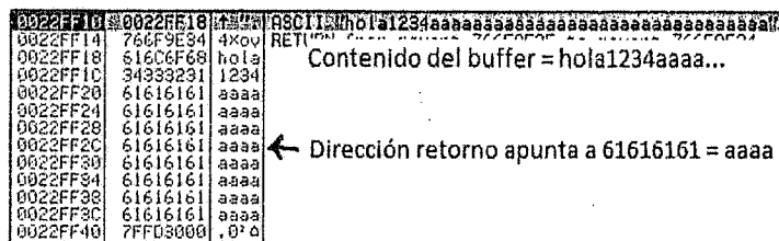
Fig 5.18: Estado de la pila en el instante previo a finalizar la ejecución de la función strcpy .
