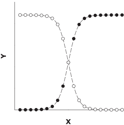
Figura XI.3. Curva logística con pendiente negativa (○) y positiva (●).
