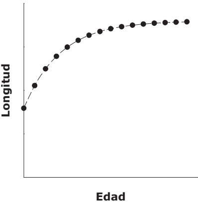
Figura XI.4. Curva de crecimiento de von Bertalanffy.
