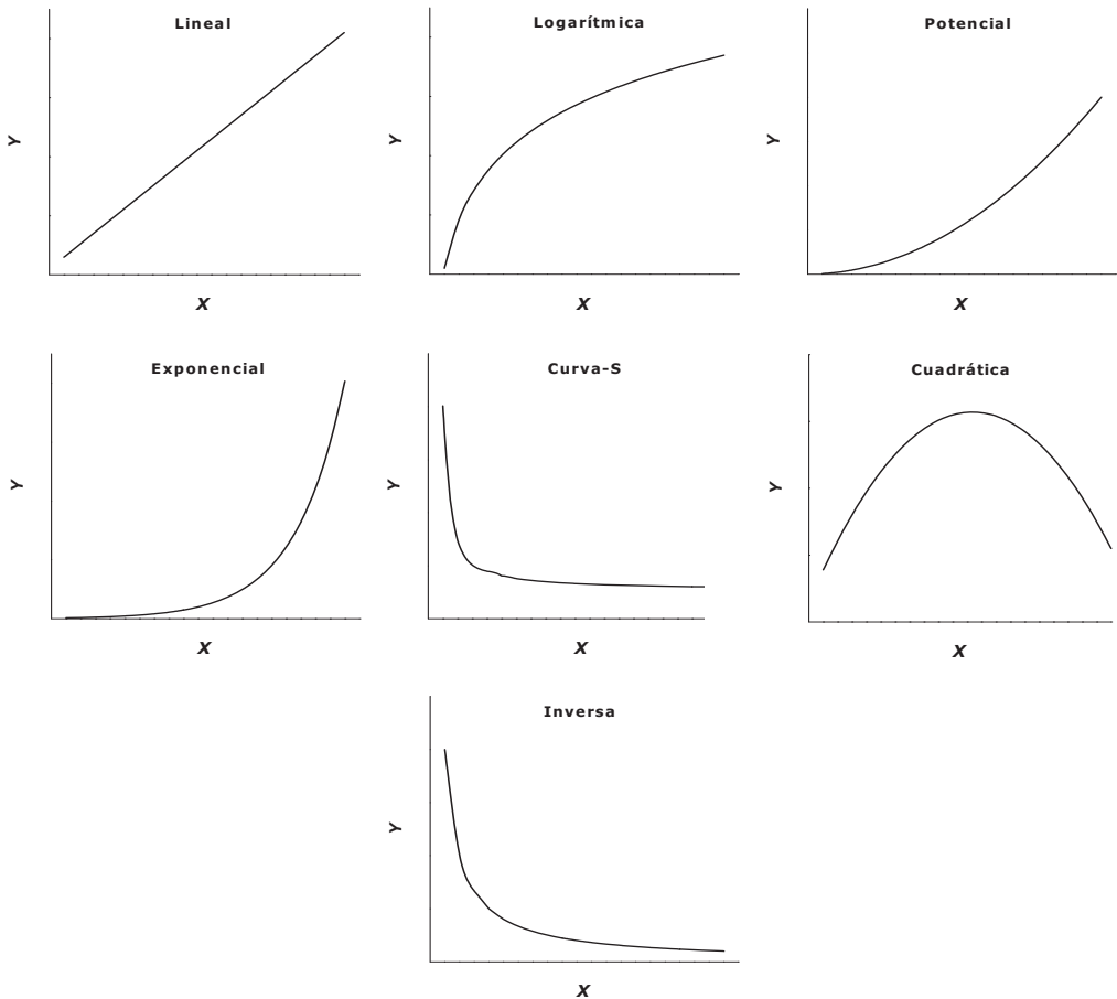
Figura XI.2. Representación gráfica de las funciones mostradas en el texto.
