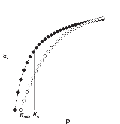
Figura XI.6. Ecuación de Monod (●) y ecuación que incluye K_{min} (○).
