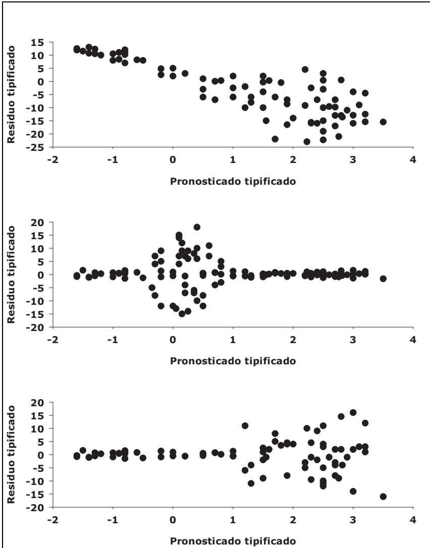
Figura XI.1. Ejemplos en los que no se cumple la homocedasticidad.
