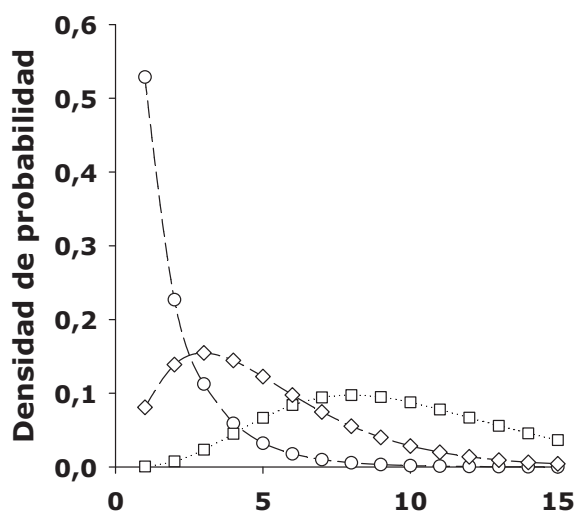
Figura III.5. Curvas de densidad de probabilidad de la distribución \chi^2 para 1 (○), 5 (◇) y 10 (□) grados de libertad.
