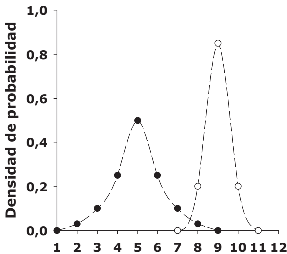
Figura III.1. Distribuciones normales con diferentes medias y desviaciones típicas.
