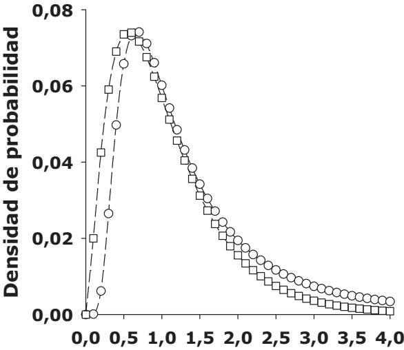
Figura III.6. Funciones de densidad de la distribución F Fisher-Snedecor para distintos grados de libertad F_{(30,5)} ( \circ ) y F_{(5,30)} ( \square ).
