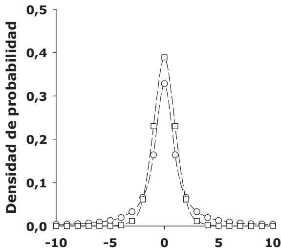
Figura III.4. Funciones de densidad de la distribución de Student para 1 (○) y 10 (□) grados de libertad.
