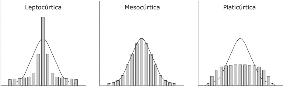
Figura III.3. Tipos de curtosis (barras) en comparación con la distribución Normal (línea continua).
