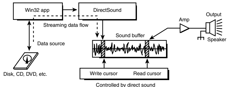
Figure 10.10 Streaming audio data.
