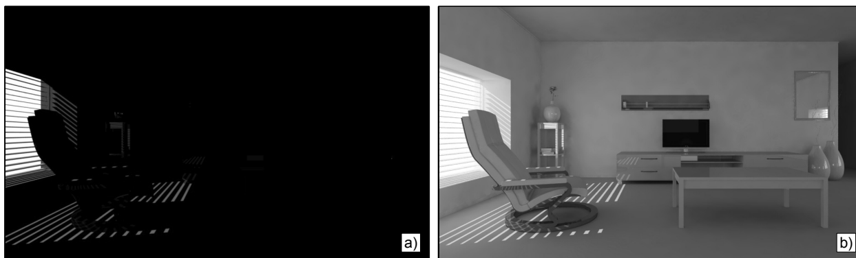
Figura 7.2: Ejemplo de resultado utilizando un modelo de iluminación local y un modelo de iluminación global con la misma configuración de fuentes de luz y propiedades de materiales. a) En el modelo de iluminación local, si no existen fuentes de luz en el interior de la habitación, los objetos aparecerán totalmente “a oscuras”, ya que no se calculan los rebotes de luz indirectos. b) Los modelos de iluminación global tienen en cuenta esas contribuciones relativas a los rebotes de luz indirectos.
