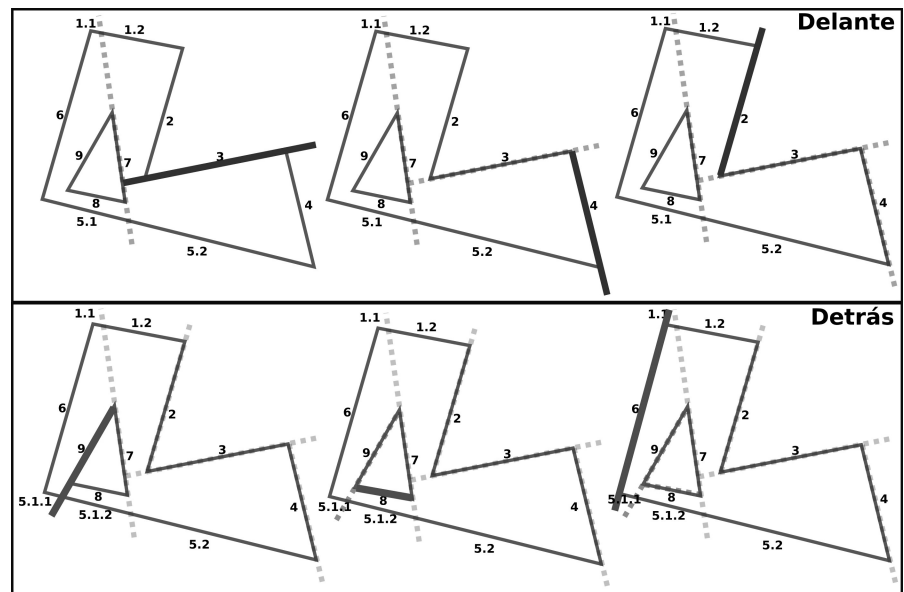
Figura 13.4: Sucesivas divisiones del nivel (BSP)
