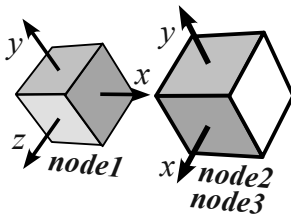
Figura 3.8: Tras aplicar la traslación de la línea 23, se aplica la rotación local al node3 . Ahora el objeto del node2 y node3 aparecen alineados exactamente en la misma posición del espacio.
