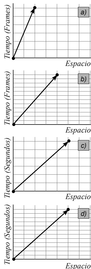
Figura 6.3: Comparación entre animación basada en frames y animación basada en tiempo. El eje de abscisas representa el espacio recorrido en una trayectoria, mientras que el eje de ordenadas representa el tiempo. En las gráficas a) y b) el tiempo se especifica en frames. En las gráficas c) y d) el tiempo se especifica en segundos. Las gráficas a) y c) se corresponden con los resultados obtenidos en un computador con bajo rendimiento gráfico (en el mismo tiempo presenta una baja tasa de frames por segundo). Las gráficas b) y d) se corresponden a un computador con el doble de frames por segundo.
