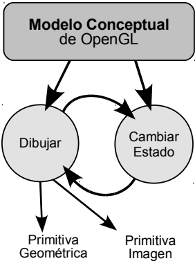
Figura 5.3: Modelo conceptual general de OpenGL.
