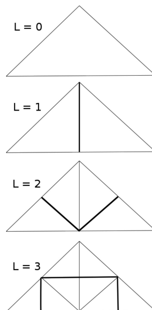
Figura 14.12: Distintos niveles de división en un BTT.
