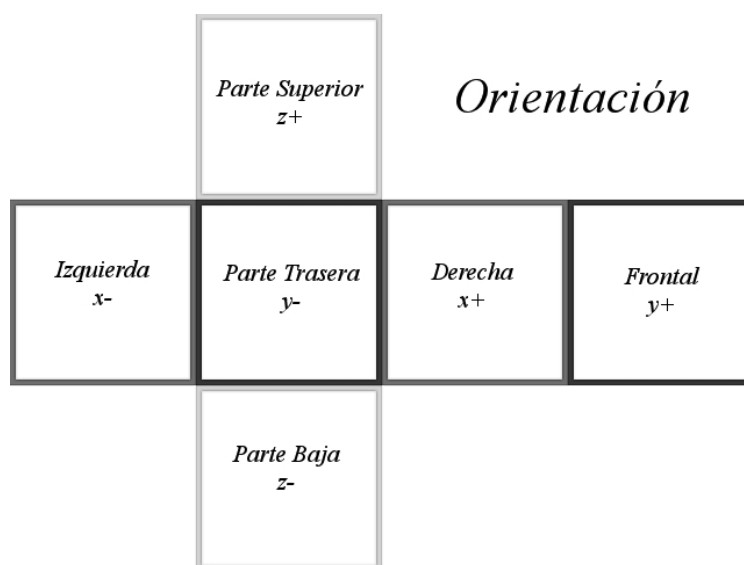
Figura 4.10: Orientación de las texturas aplicadas a un cubo
