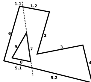
Figura 13.3: Primera división (BSP).
