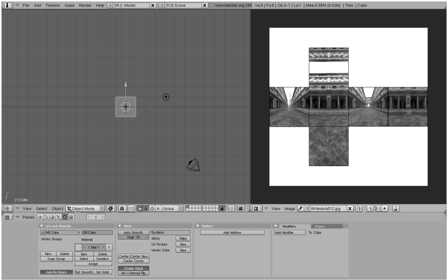
Figura 4.12: Editor de Blender con una división en dos marcos. En la parte izquierda aparece la figura geométrica a texturizar y en la parte derecha las texturas que serán aplicadas mediante la técnica de UV/Mapping
