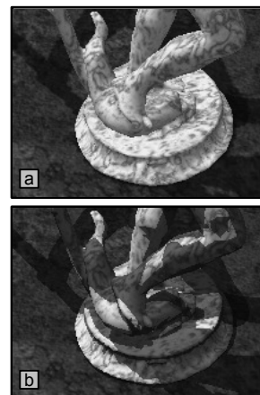
Figura 9.6: En el cálculo de sombras mediante Mapas de Textura (en a )), el objeto emisor de sombras no recibe su propia sombra proyectada. Empleando el Stencil Buffer ( b )) es posible recibir la sombra proyectada.
