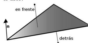
Figura 13.1: Posición con respecto a un plano de normal n .
