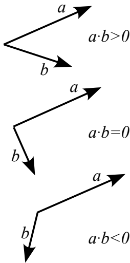
Figura 2.6: Algunos ejemplos de uso del producto escalar.
