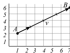
Figura 2.21: Ejemplo de interpolación lineal entre dos puntos. Se han marcado sobre el vector \vec{v} los puntos correspondientes a t = 0,25 , t = 0,5 y t = 0,75 .
