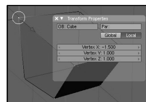
Figura 4.19: Ventana emergente al pulsar la tecla N para indicar los valores numéricos de coordenadas de los vértices del modelo.
