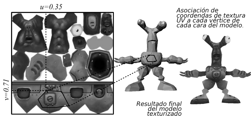
Figura 7.7: Asignación de coordenadas UV a un modelo poligonal. Esta operación suele realizarse con el soporte de alguna herramienta de edición 3D.
