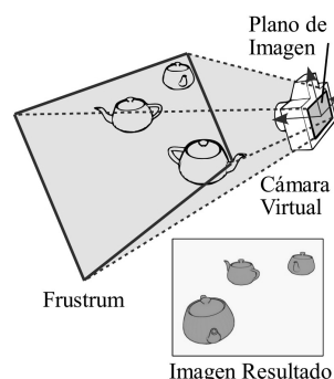
Figura 1.1: Descripción general del proceso de rendering .
