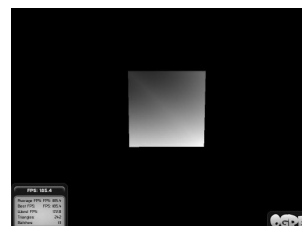
Figura 12.9: El cuadrado aparece con el color de sus cuatro vértices interpolado.
