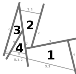
Figura 13.9: Nivel dividido en celdas (l-BSP).
