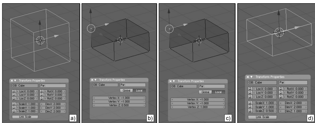
Figura 4.20: Aplicación de transformaciones geométricas en modo Edición. a) Situación inicial del modelo al que le aplicaremos un escalado de 0.5 respecto del eje Z. b) El escalado se aplica en modo Edición. El campo Vertex Z muestra el valor correcto. c) Si el escalado se aplicó en modo objeto, el campo Vertex Z no refleja la geometría real del objeto. Esto puede comprobarse fácilmente si alguno de los campos Scale no son igual a uno, como en d) .
