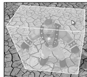
Figura 4.35: En el caso de objetos móviles, Ogre emplea una caja límite (definida por las coordenadas mayor y menor de los vértices del modelo) para calcular la intersección rayo-objeto y optimizar así los cálculos. Esto implica que, en el caso del test de intersección de la figura daría que hay colisión entre el rayo y el objeto. No obstante, es posible realizar manualmente un test de colisión con precisión (a nivel de polígono) si el juego lo requiere.
