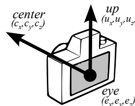
Figura 5.7: Parámetros de la función gluLookat .
