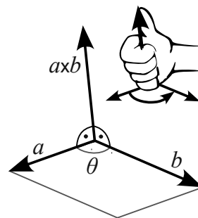
Figura 2.7: Representación del producto vectorial. El módulo del producto vectorial a \times b es igual al área del paralelogramo representado en la figura.
