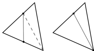
Figura 13.6: División de un triángulo por un plano.
