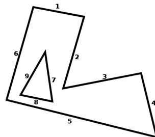
Figura 13.2: Mapa de una escena visto desde arriba.
