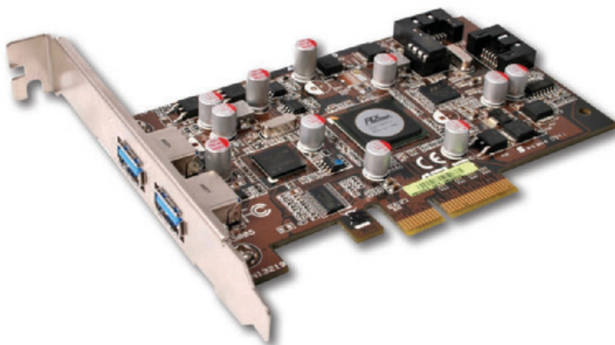
Figura 9. Placa controladora PCI-Express x4, de cuatro puertos USB 3.0 (dos internos y dos externos).
