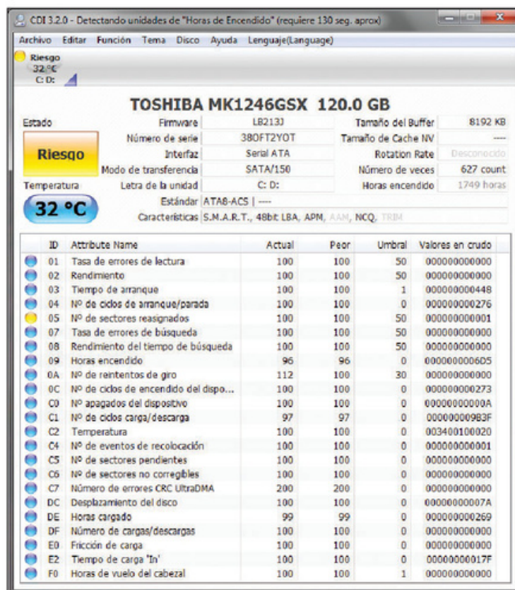
Figura 24. El software CrystaDiskInfo para diagnósticos S.M.A.R.T. indica que la unidad de disco está en riesgo debido a la cantidad de sectores reubicados.
