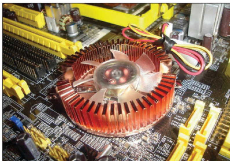
Figura 5. Los motherboards de gama alta instalan un ventilador en el northbridge de su chipset para refrigerarlo de mejor forma.
