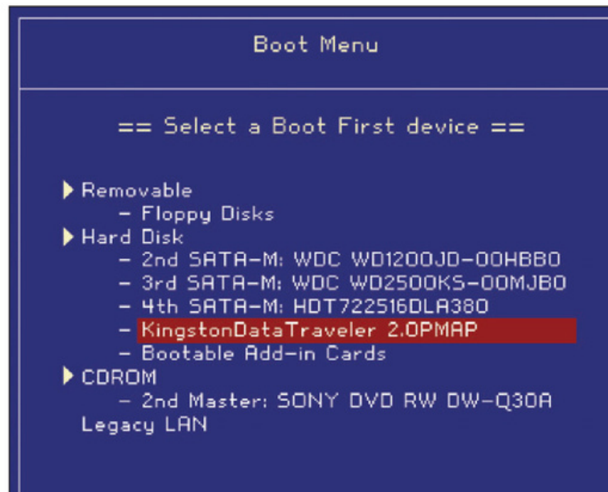
Figura 21. Menú BBS en un BIOS marca Phoenix-Award, donde despliega la lista de posibles soportes de booteo.
