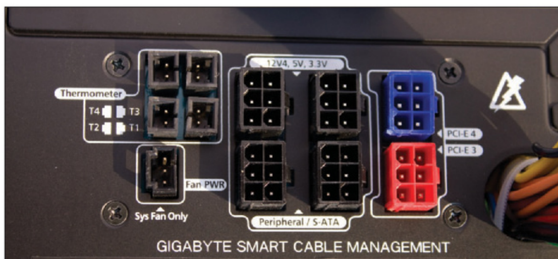
Figura 13. Conectores libres en una fuente semimodular.
