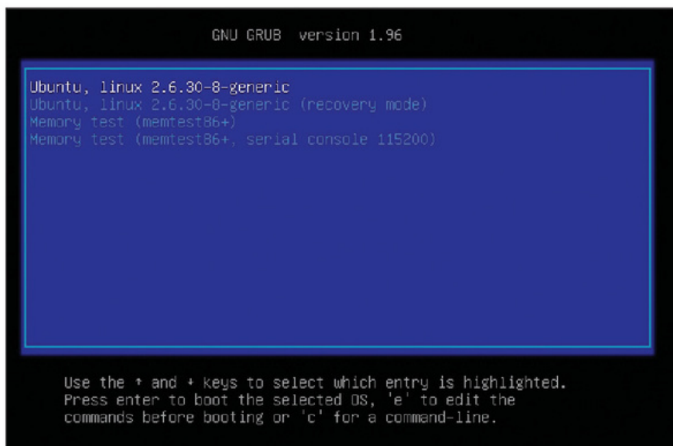
Figura 31. GRUB en modo texto es compatible con cualquier interfaz de video obsoleta, pero su apariencia es algo anticuada.
