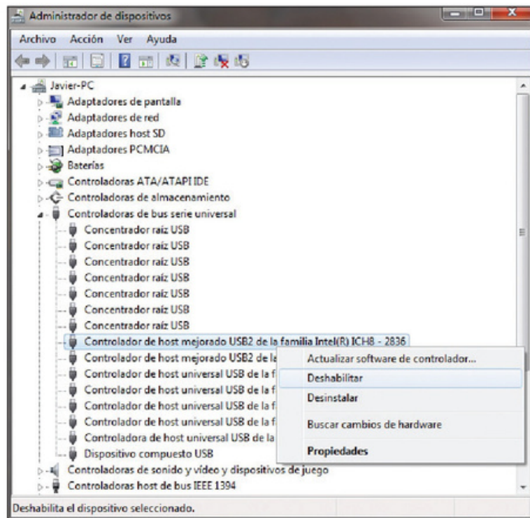
Figura 12. Desde el menú contextual de la controladora de host mejorada, en el Administrador de dispositivos , podemos habilitar la operación con USB 1.1.
