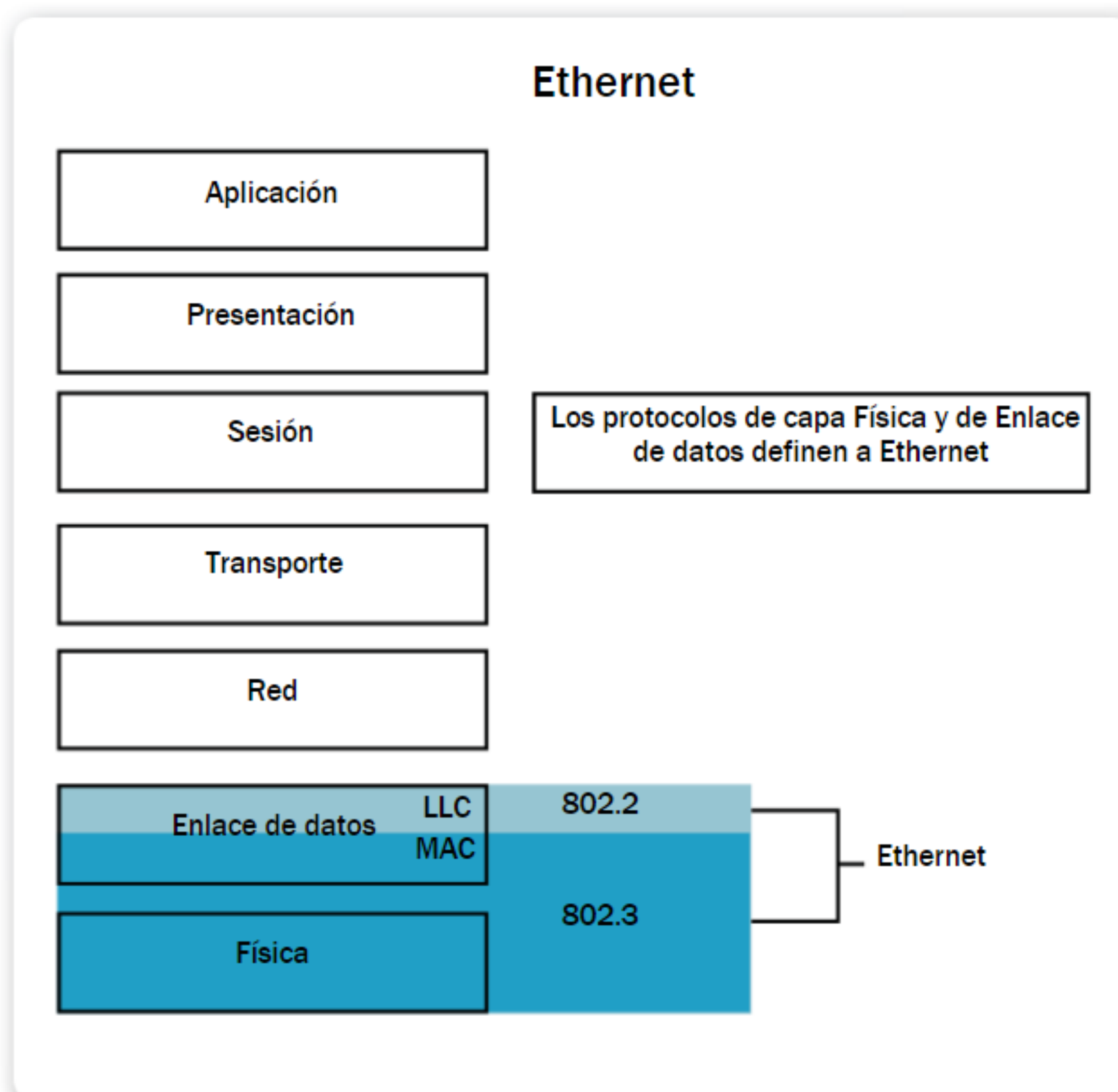
Figura 12. Esquema que abarca la norma 802.3 y la capa física de Ethernet.
