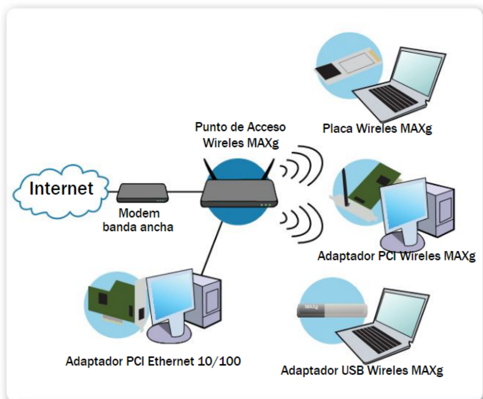
Figura 8. Infraestructura que combina conexiones Ethernet e inalámbricas.
