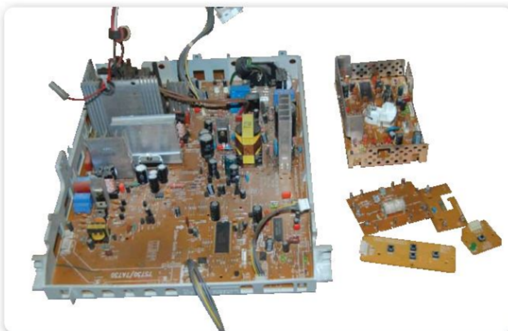
Figura 13. A la derecha, la placa base del monitor. A la izquierda vemos la placa del cañón.
