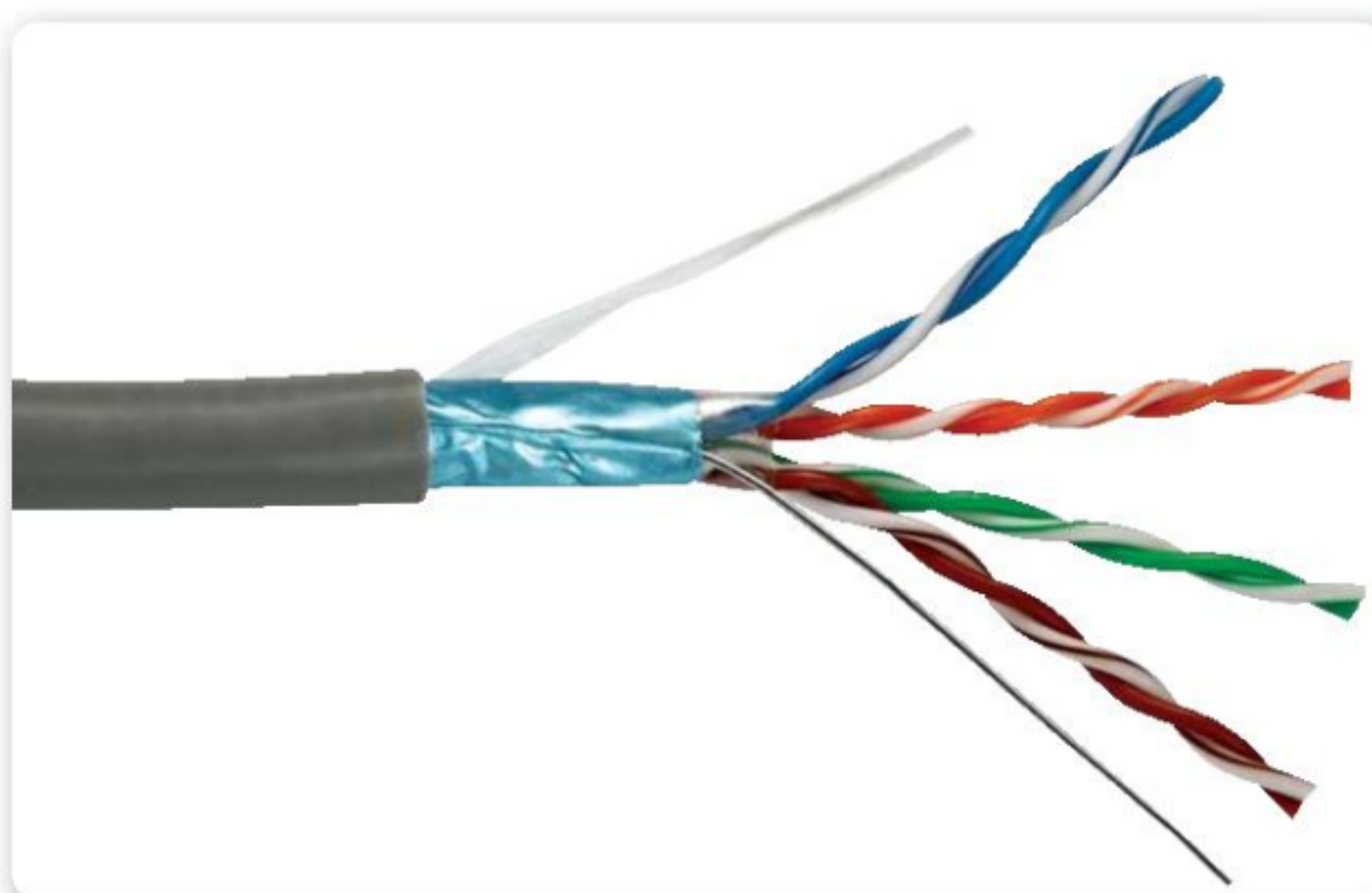
Figura 18. La elección de cable blindado o de UTP está determinada por el presupuesto y la seguridad.
