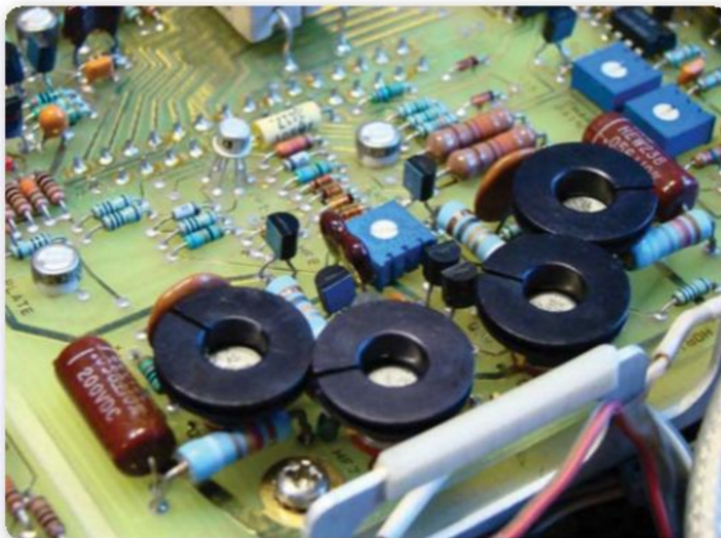
Figura 14. Los cuadrados azules son los presets que encontramos sobre la placa del monitor.
