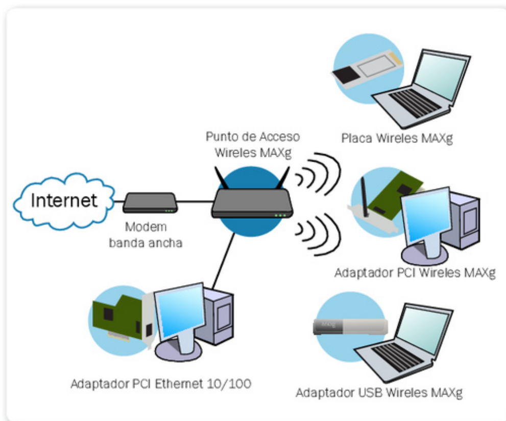
Figura 8. Infraestructura que combina conexiones Ethernet e inalámbricas.
