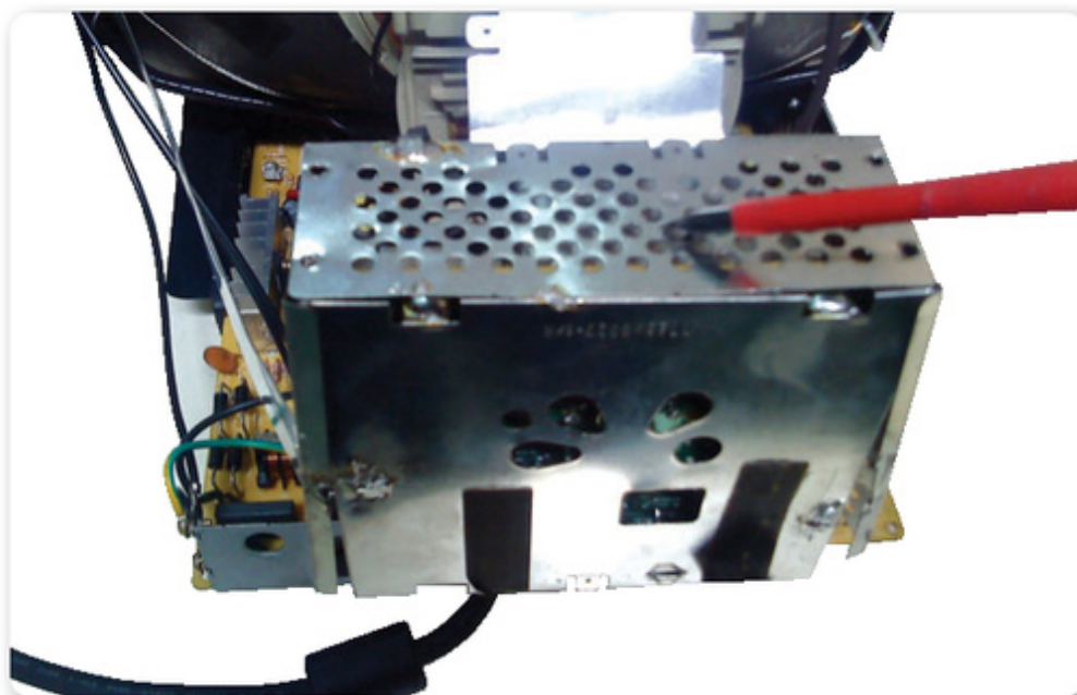
Figura 9. Acercamiento al interior de un monitor CRT.
