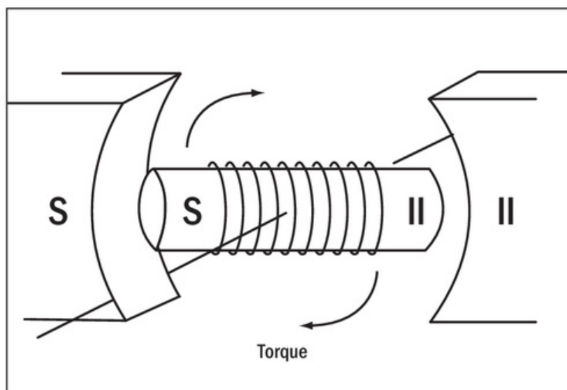
Figura 3. Efecto de giro del motor gracias a la atracción/el rechazo del núcleo de la bobina y los imanes de la carcasa.
