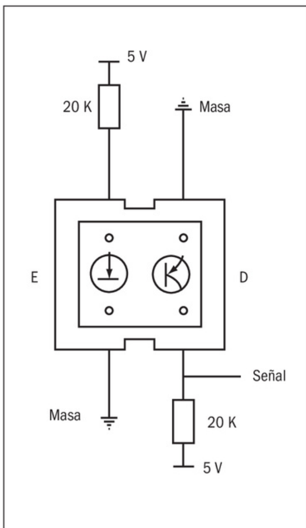
Figura 13. Conexión del CNY70 para usarlo como sensor analógico.
