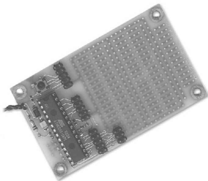
Figura 15. ATmega8 en una placa de prototipado rápido.
