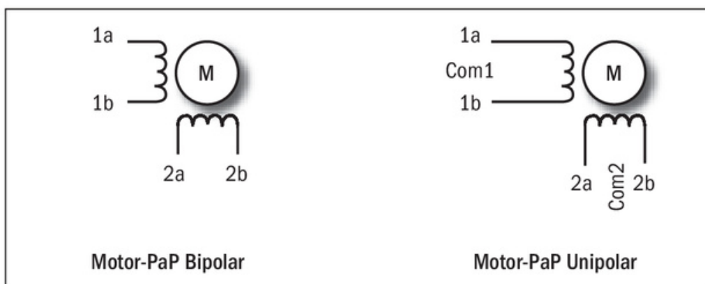
Figura 10. Esquemas de las bobinas de los motores bipolares y unipolares.
