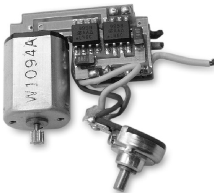
Figura 14. Un servo visto por dentro.
