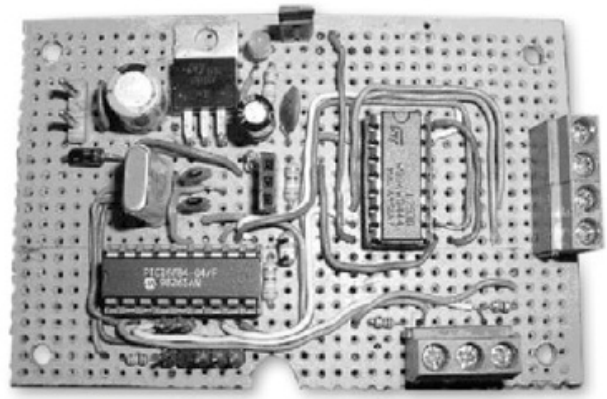
Figura 9. Visión final del controlador desarrollado sobre una placa experimental.
