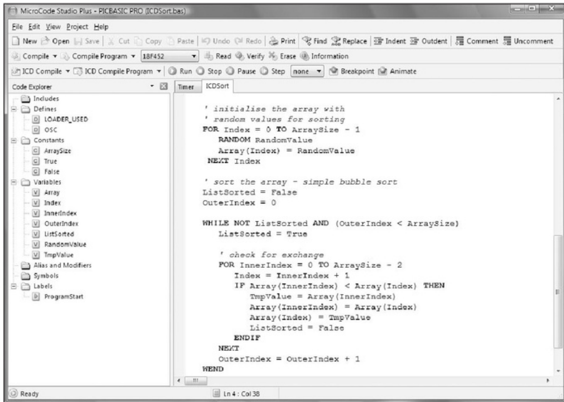
Figura 2. Vista del MicroCode Studio Plus , IDE para el PicBasic Pro .
