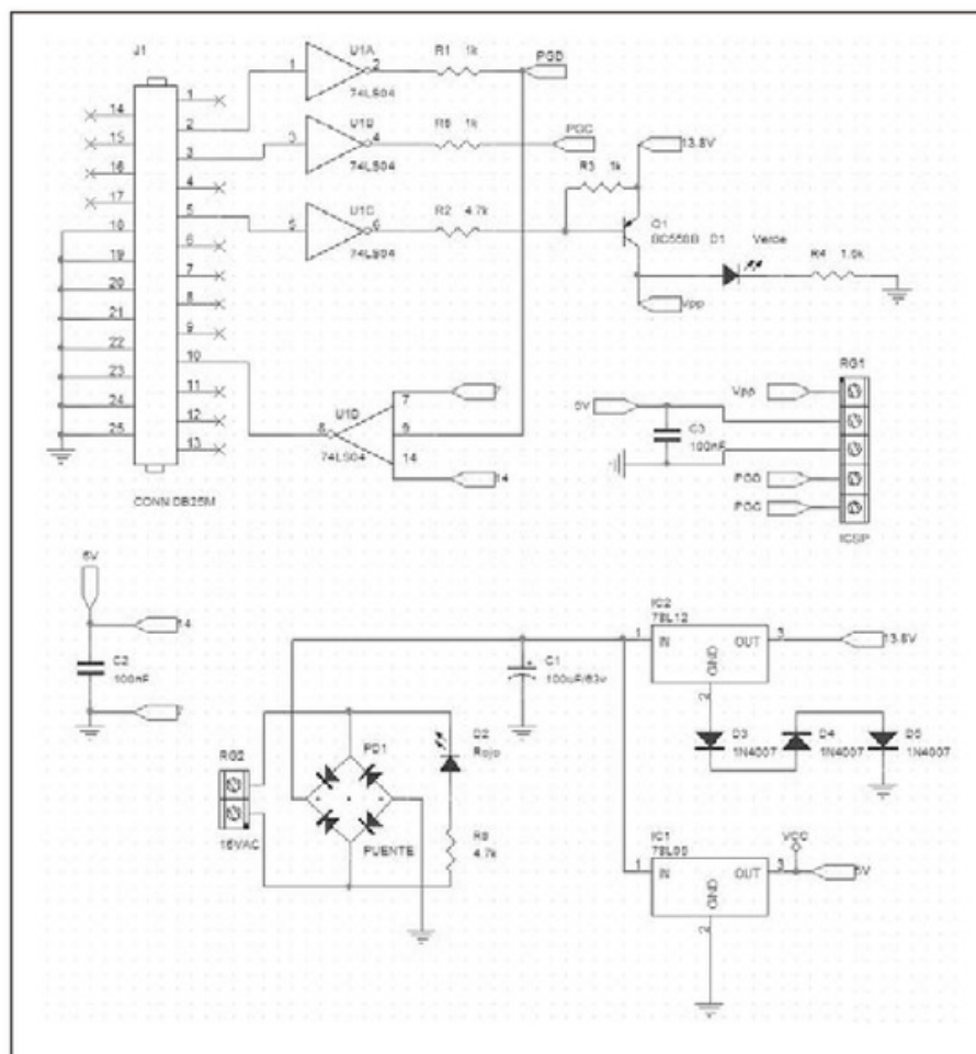
Figura 12. Esquema del programador GTP LITE.
