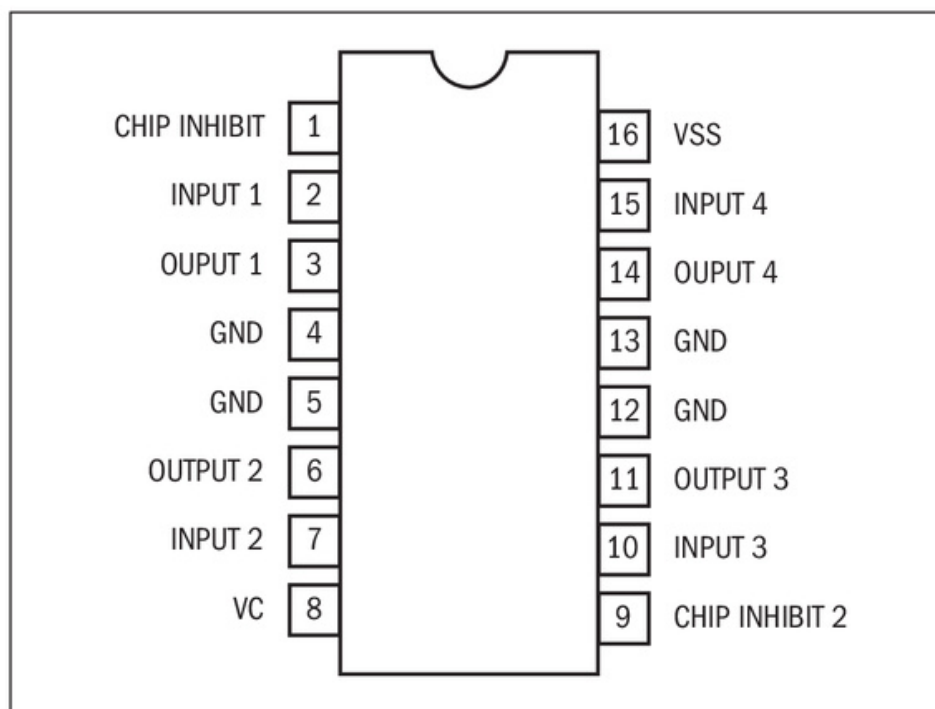
Figura 5. Esquema del integrado controlador de los motores L293D.
