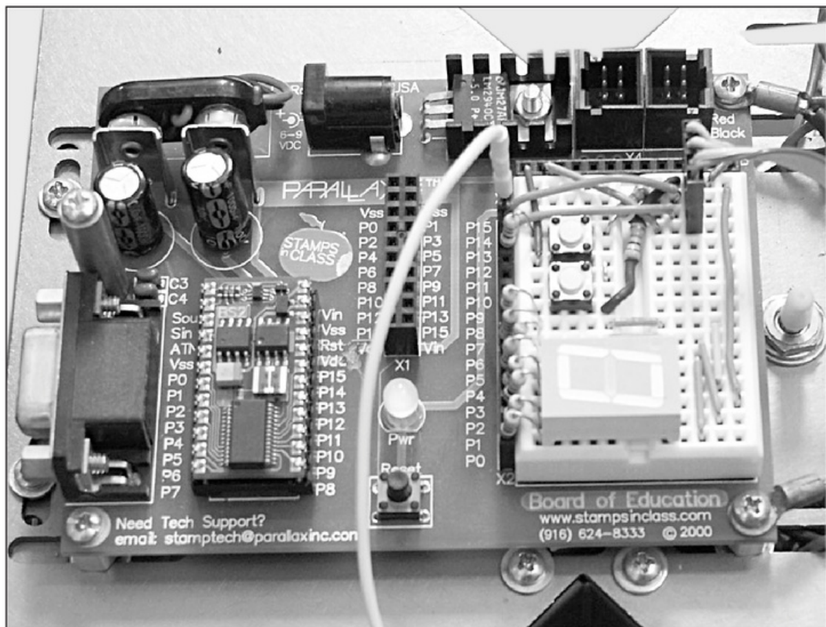
Figura 11. Placa educativa del Basic Stamp de Parallax.
