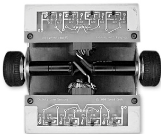
Figura 10. Sensores en un robot seguidor de línea creado por David Cook.
