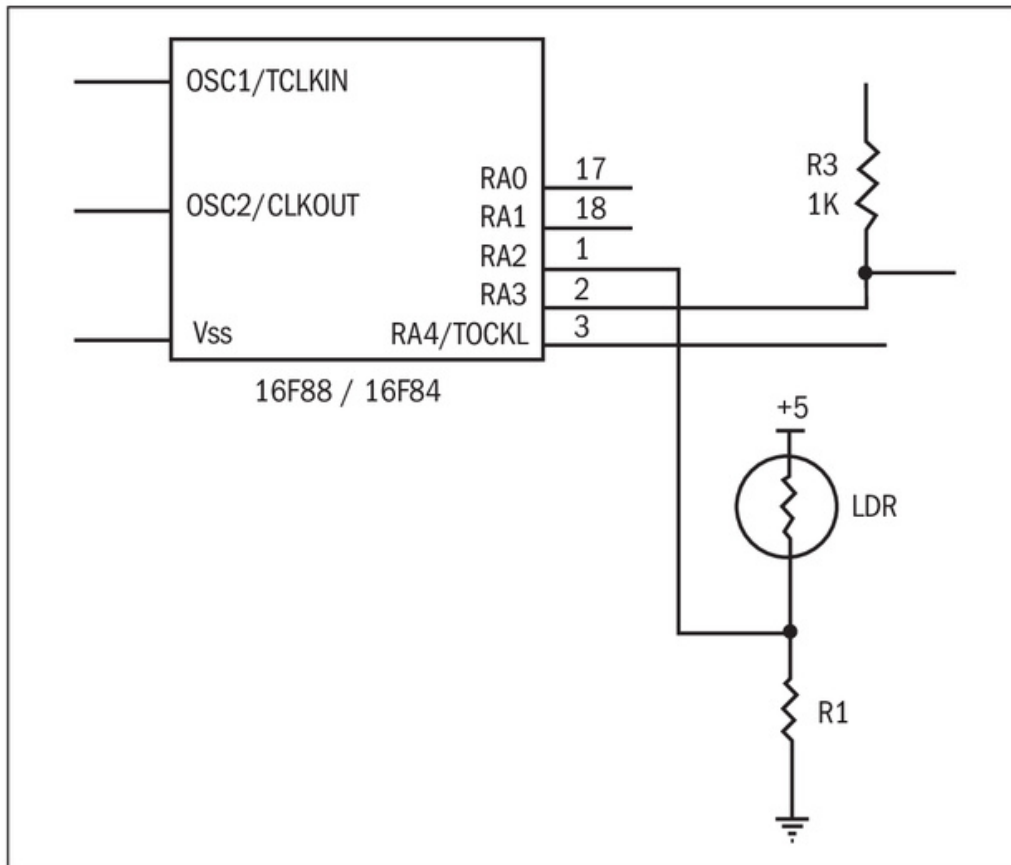
Figura 14. Conexión del LDR a nuestro controlador.
