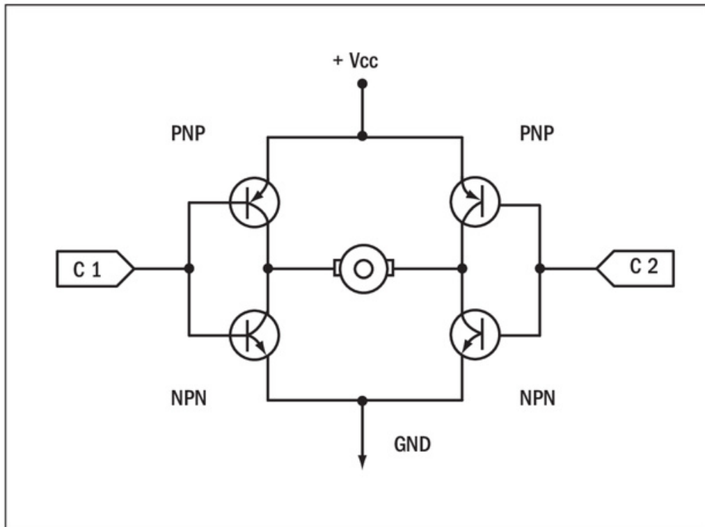
Figura 4. Esquema básico de un puente H.
