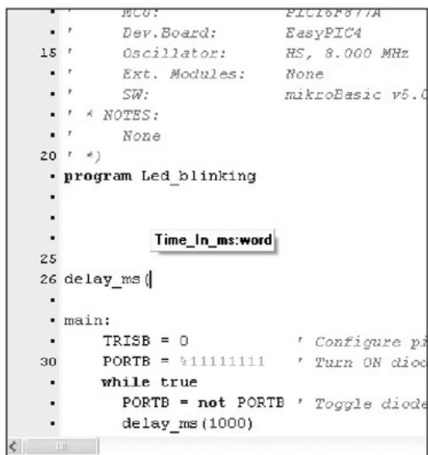
Figura 8. Asistente que informa los parámetros de las funciones.
