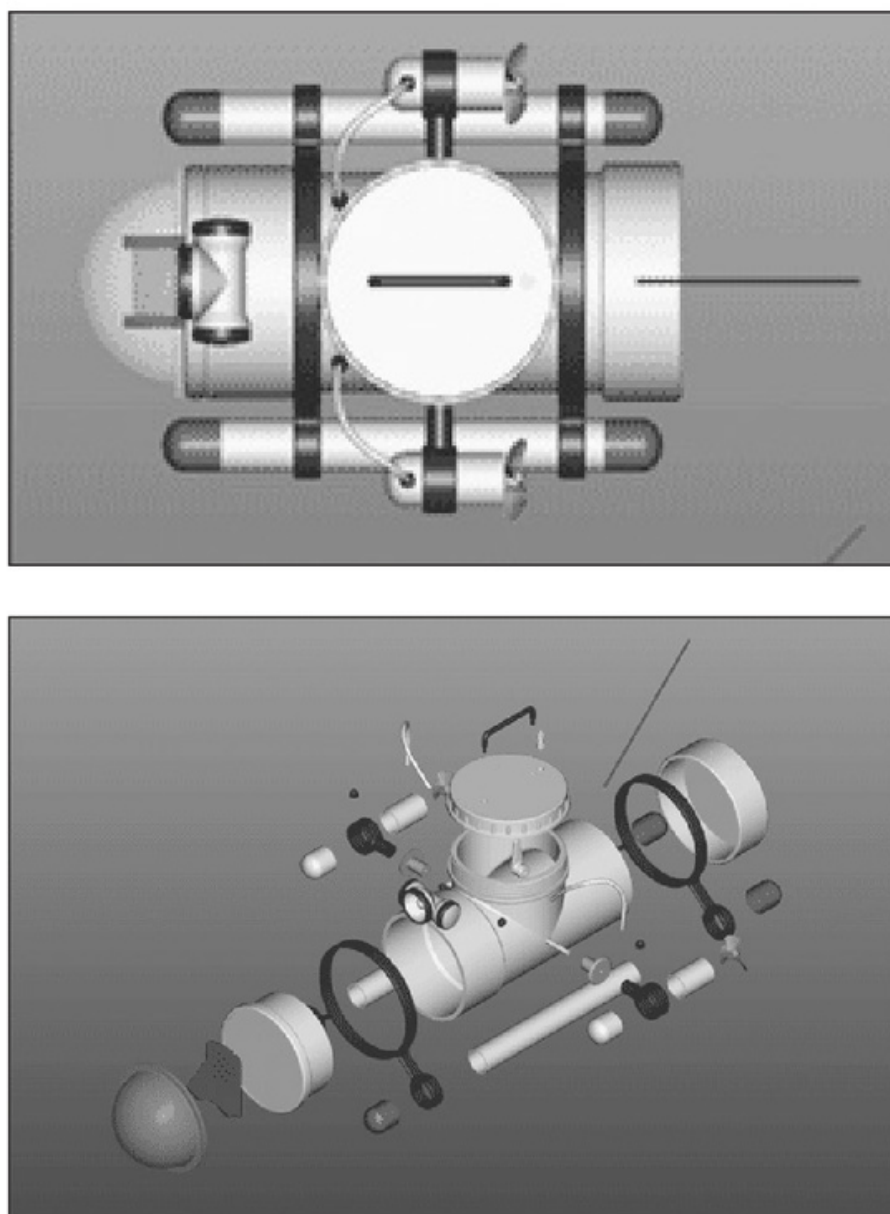
Figura 6. Explorador subacuático realizado por alumnos de una escuela media de Argentina. No es autónomo, pero resuelve todas las dificultades mecánicas de un robot submarino.
