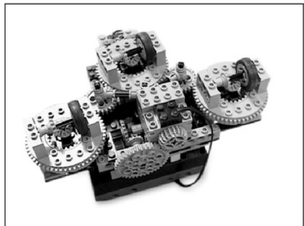
Figura 13. Un robot de configuración síncrona hecho con Lego. Se puede observar el engranaje que alimenta el giro de la rueda y el que alimenta la rotación del soporte de ésta.
