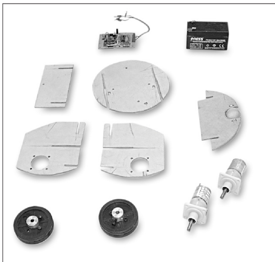
Figura 19. Conjunto total con las 14 piezas que componen nuestro robot.
