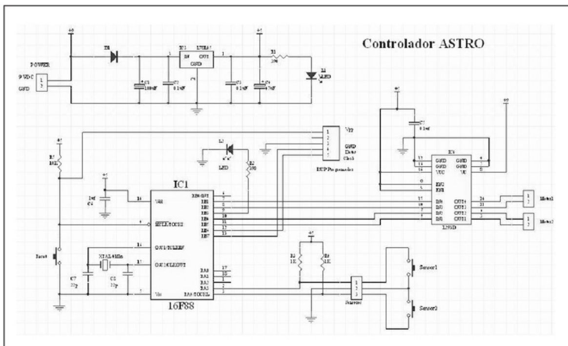
Figura 7. Esquema del circuito del controlador de nuestro robot.
