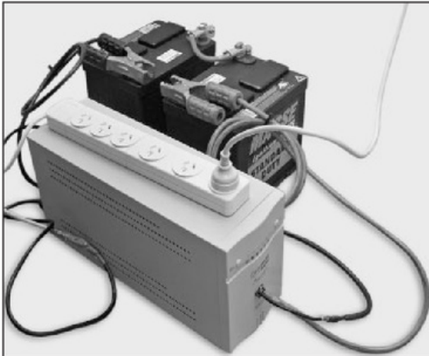
Figura 7. Una UPS alimentada por una batería de plomo-ácido .
