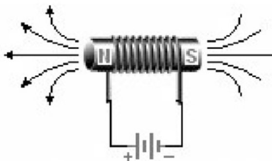
Figura 2. Si invertimos la polaridad de la bobina, cambiamos los polos del núcleo.
