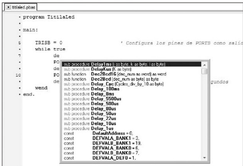
Figura 7. Ejemplo de la lista presentada por el asistente de código cuando escribimos de y luego CTRL + ESPACIO .
