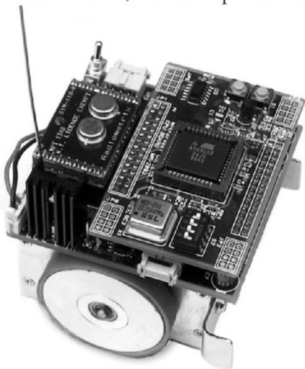
Figura 3. Ejemplo de robot de fútbol con ruedas diferenciales.
