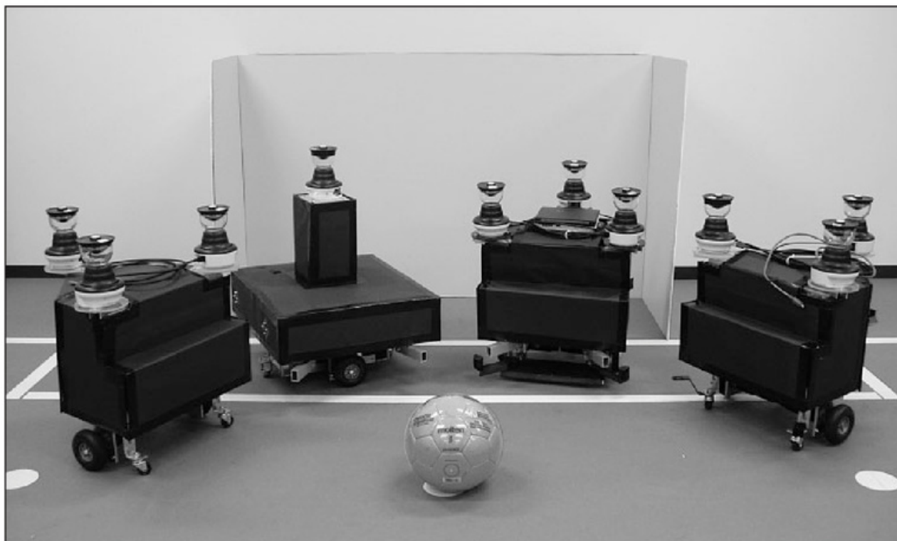
Figura 5. Ejemplos de robots seguidores de una pelota infrarroja.
