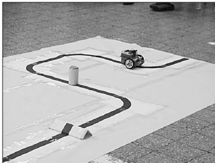
Figura 2. Seguimiento de línea con obstáculos.
