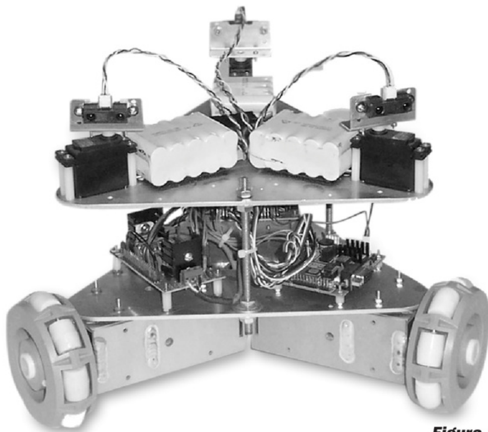
Figura 17. Arquitectura de un robot con tres ruedas omnidireccionales.
