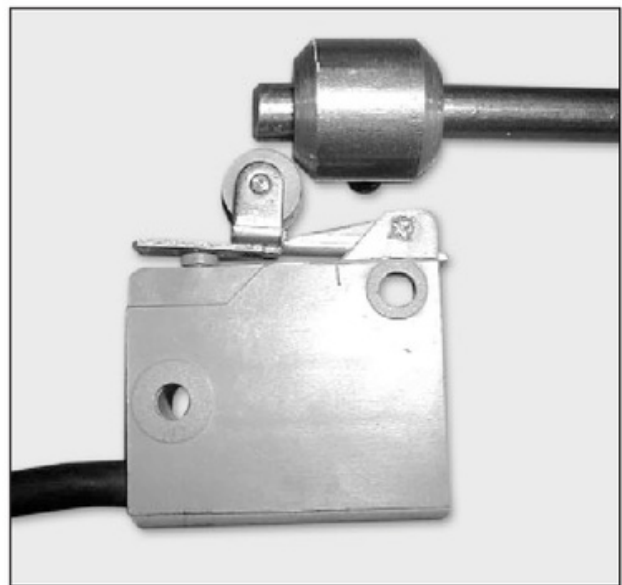
Figura 9. Un ejemplo de sensor de final de carrera.
