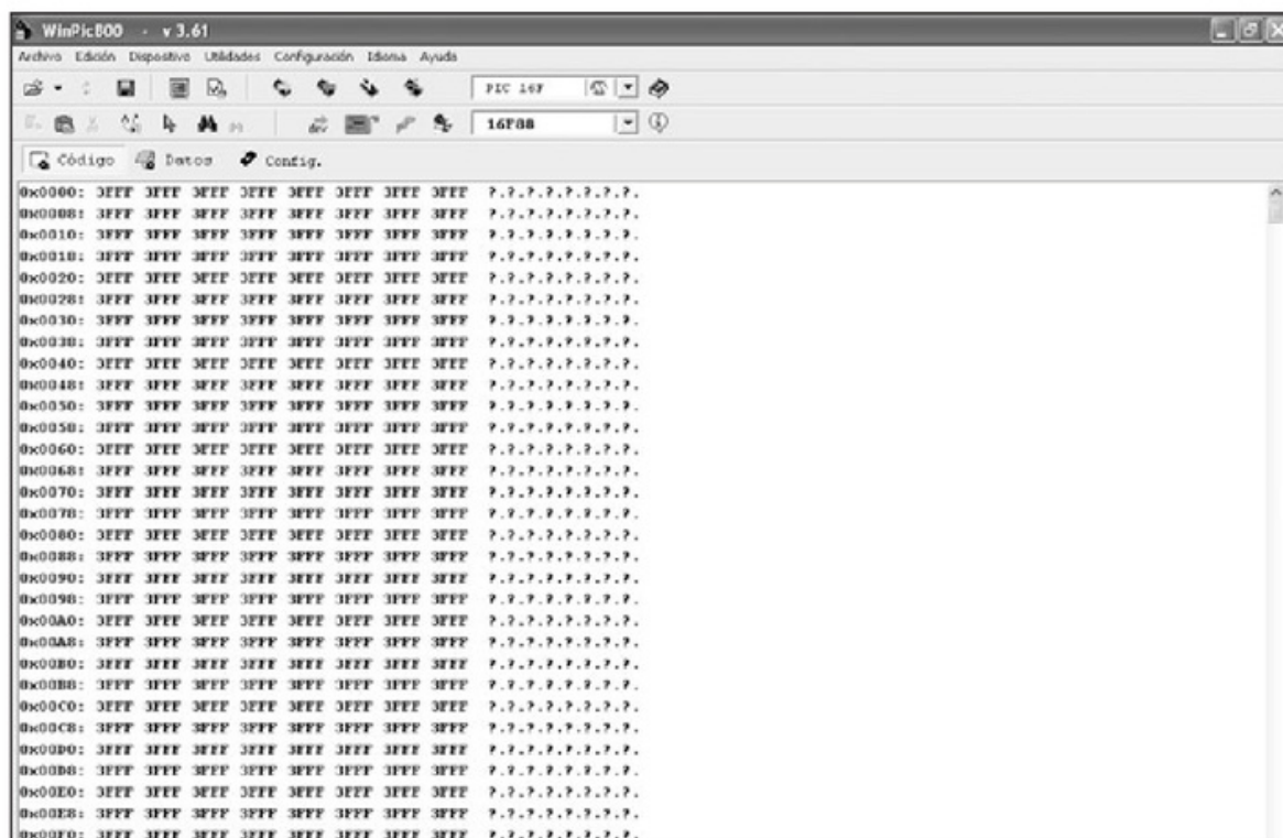
Figura 11. Pantalla principal del WinPic800 , configurada para el 16F88.
