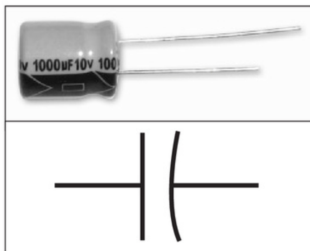
Figura 4. Capacitor electrolítico y símbolo electrónico del capacitor. Podemos ver la marca de la patita que debe ir a tierra.
