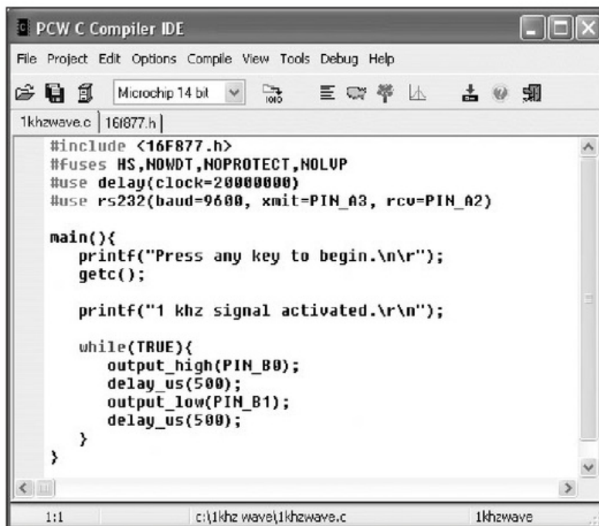
Figura 3. Vista del editor C Aware de CCS .
