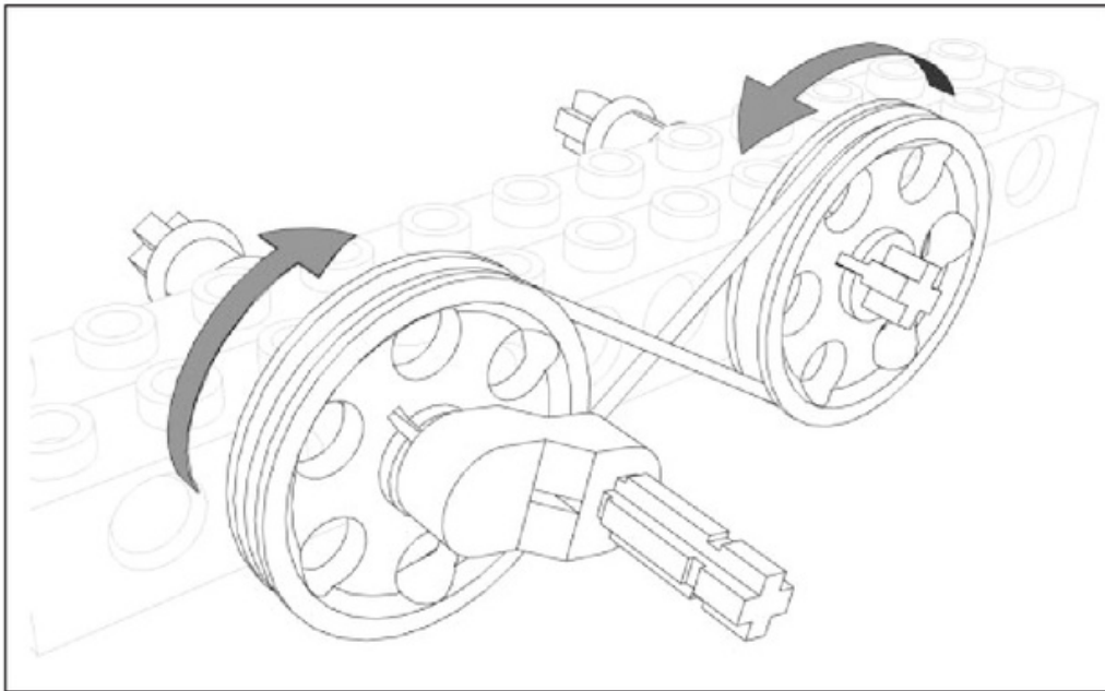
Figura 29. En esta imagen podemos observar cómo funciona la inversión del sentido de rotación de la polea de salida.
