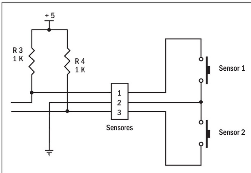
Figura 5. Conexión de los dos interruptores en nuestro controlador.
