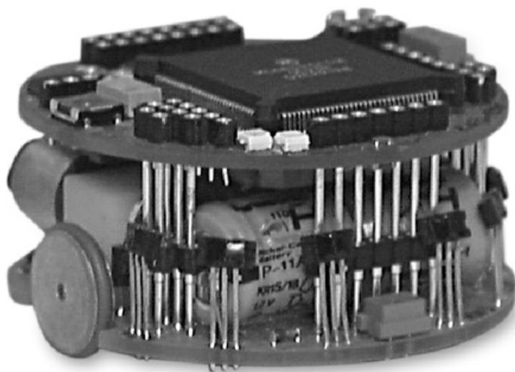
Figura 1. Kepera es un robot con ocho sensores infrarrojos y una cámara de visión lineal.
