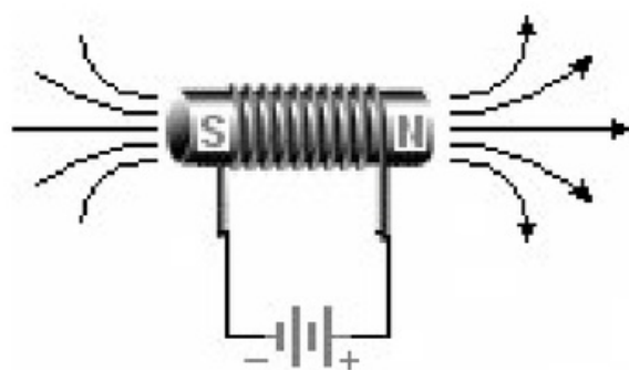
Figura 1. Determinación de los polos por el pasaje de corriente en la bobina.
