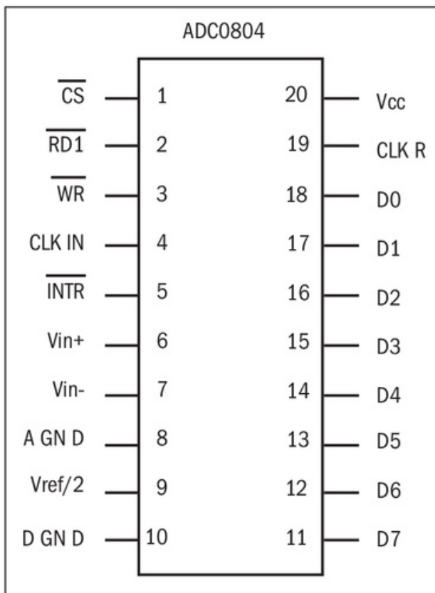
Figura 12. Esquema del conversor A/D ADC0804.
