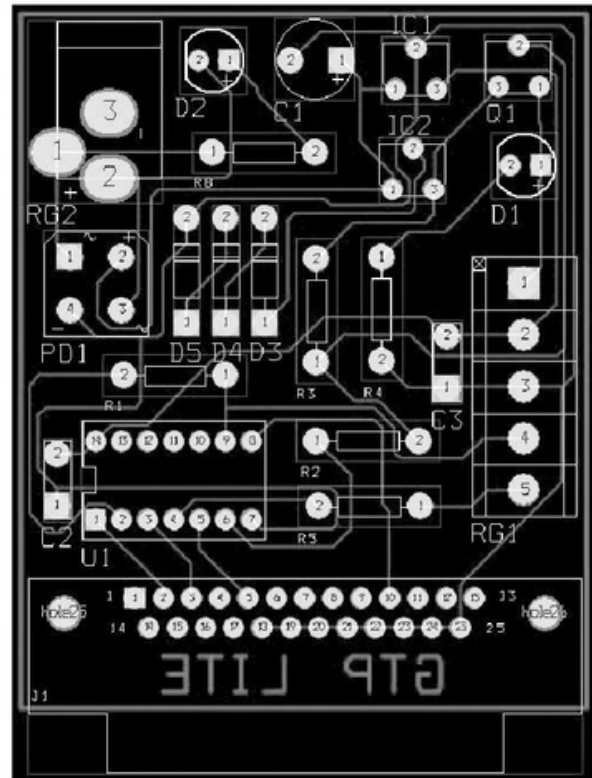
Figura 13. En esta imagen podemos ver el board del GTP LITE.
