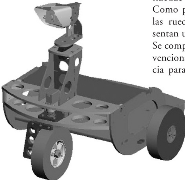
Figura 14. Esquema de un robot con arquitectura de triciclo.
