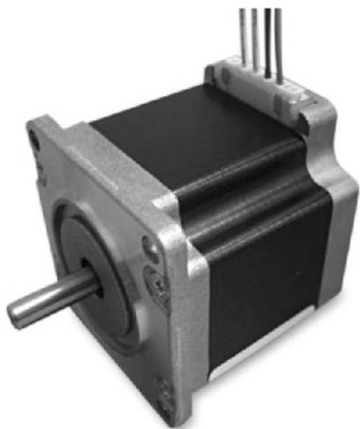
Figura 11. Un ejemplo de motor bipolar, con 4 cables.
