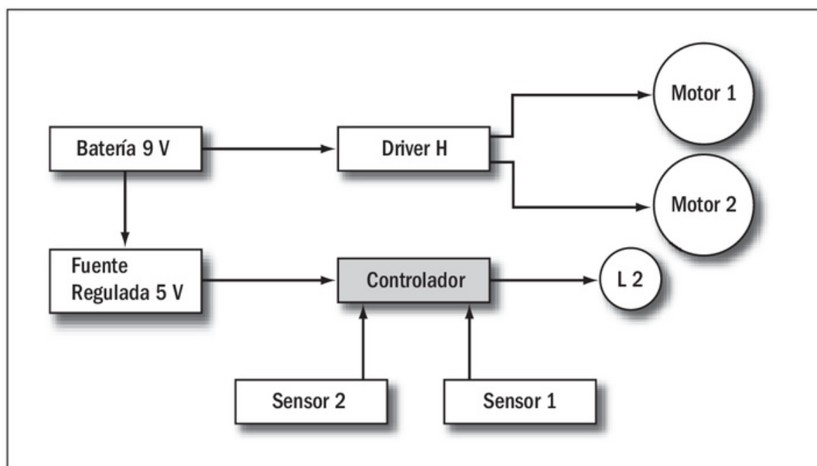
Figura 8. En esta figura podemos observar los bloques lógicos que componen nuestro controlador.
