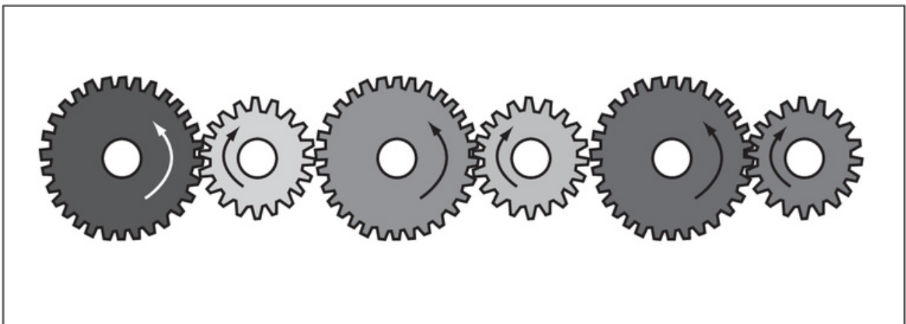
Figura 27. Sentido de rotación de cada engranaje en un conjunto de engranajes solidarios.
