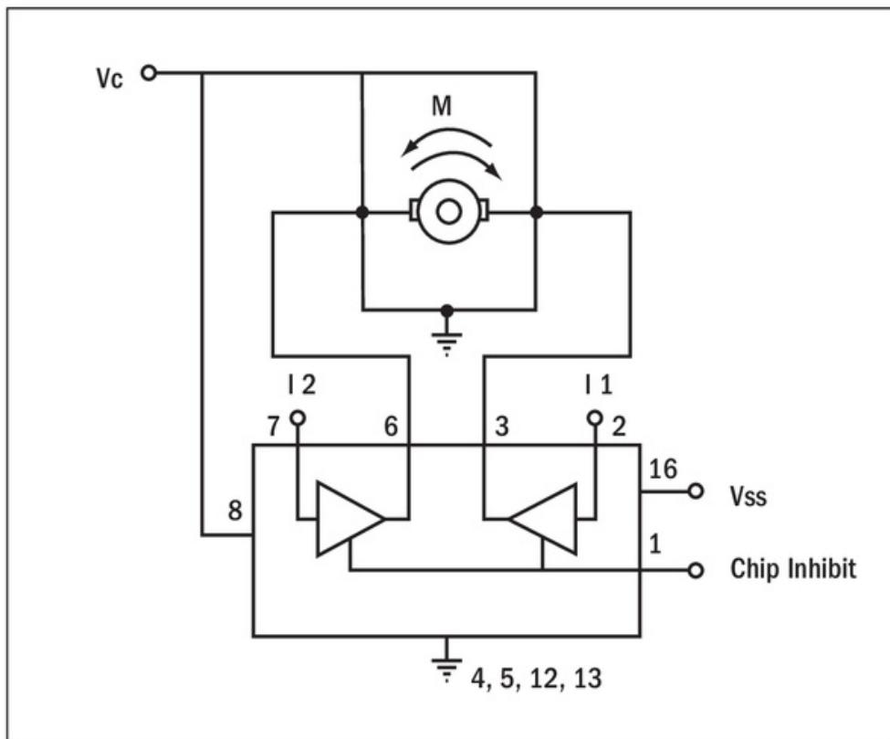
Figura 5. Diseño de conexiones para controlar un motor con inversión de giro mediante el uso del L293D .
