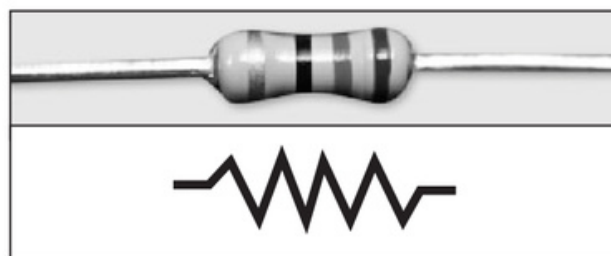
Figura 3. Resistencia de 62\Omega \pm 5\% y símbolo electrónico de la resistencia.
