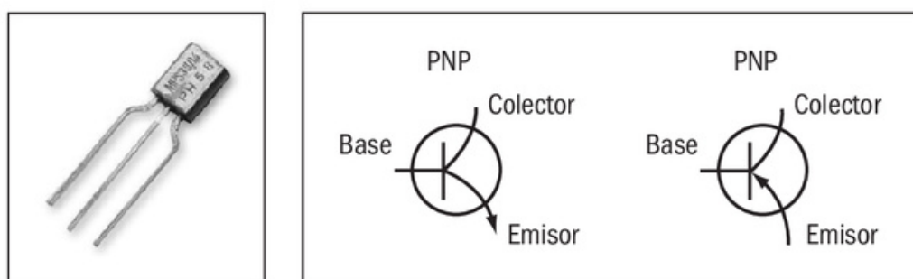
Figura 7. Un transistor y los símbolos para NPN (en el que la flecha va hacia fuera) y PNP
