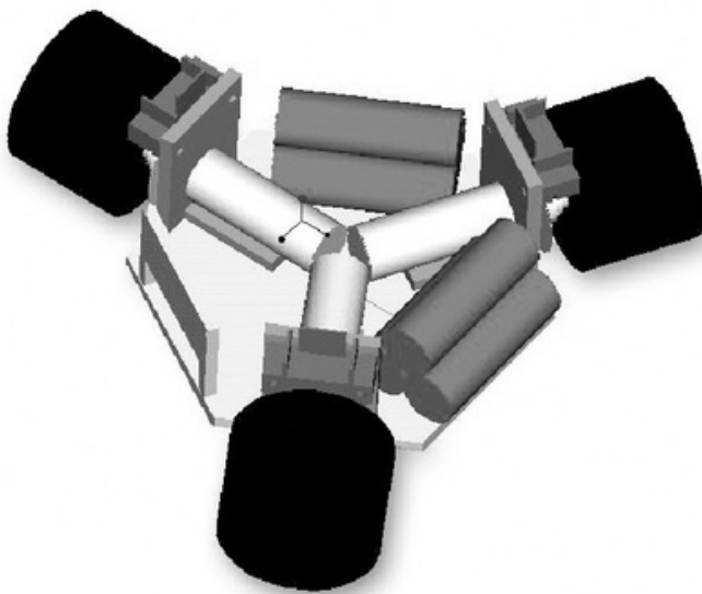
Figura 7. Arquitectura de un robot con ruedas omnidireccionales.
