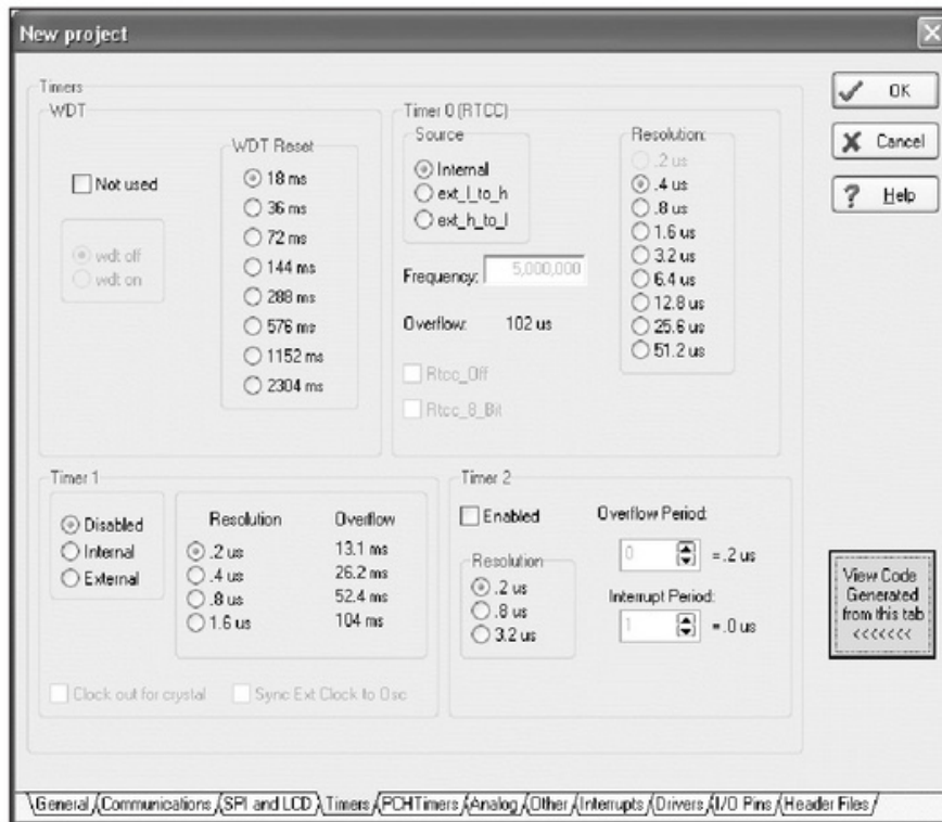
Figura 4. Asistente de proyectos del PCW.
