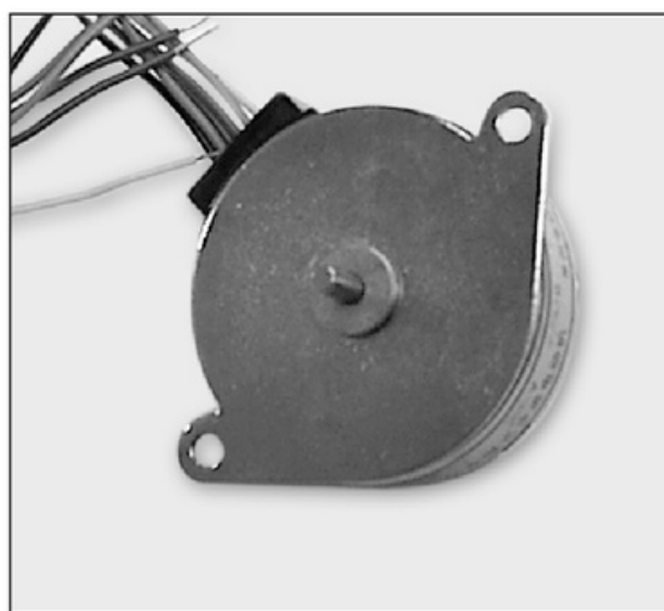
Figura 12. Ejemplo de motor unipolar con 5 cables, que tiene los dos rojos comunes.
