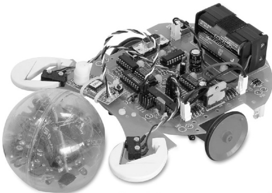
Figura 6. Un equipo con sistema de visión local. La cámara apunta hacia una semiesfera en la parte superior.
