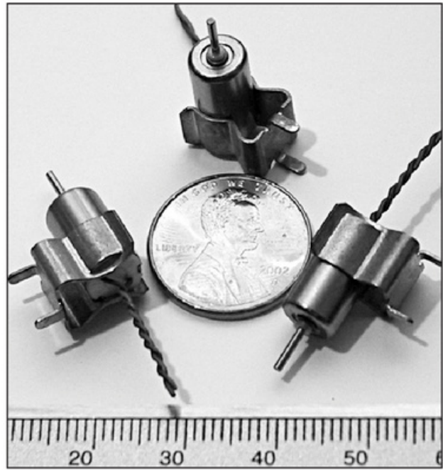
Figura 5. Motores de corriente continua de tamaño reducido.
