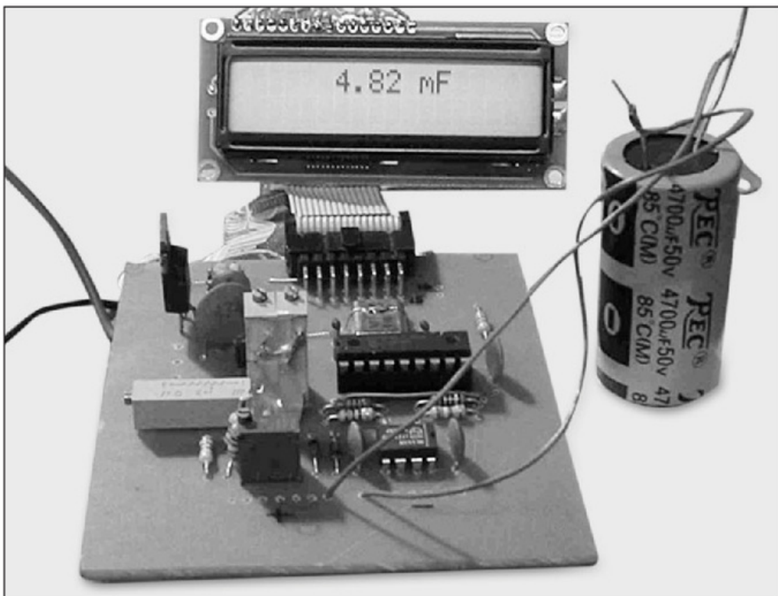
Figura 5. Capacímetro digital basado en un 16F84 con display de LCD, desarrollado por Sonytel Argentina.
