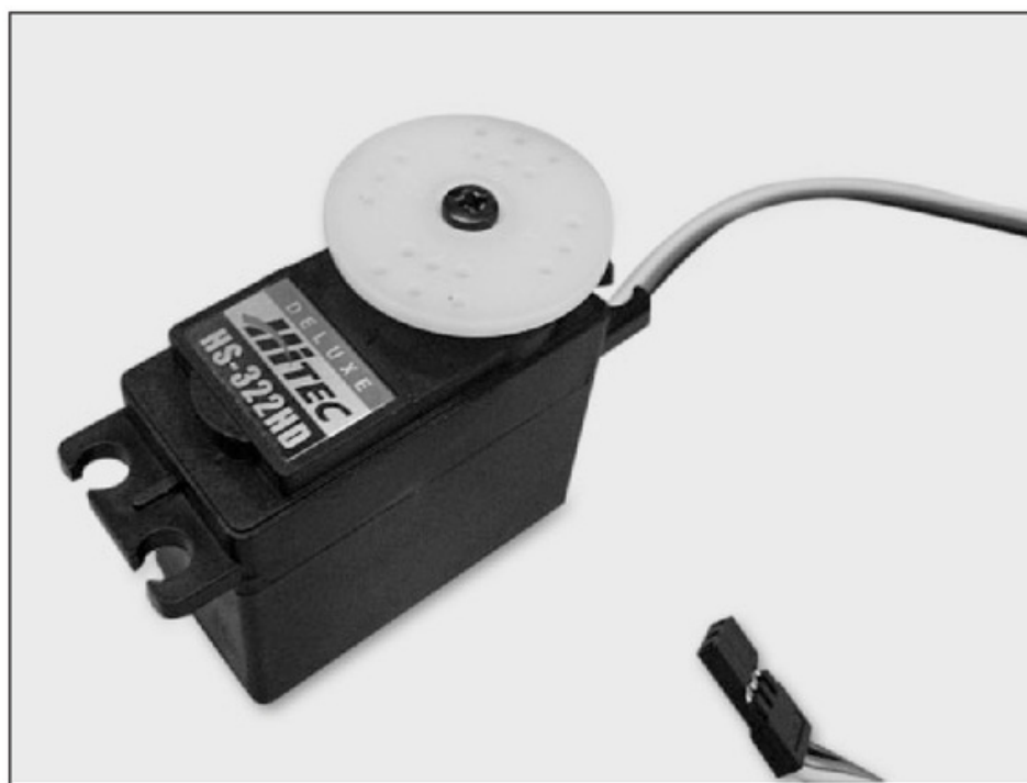
Figura 13. Servomotor Hitec, muy utilizado en robótica.
