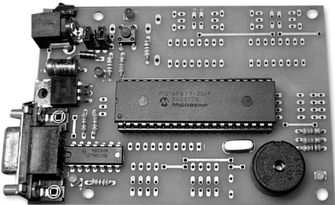
Figura 4. Un microcontrolador PIC montado en una placa controladora GoGo .
