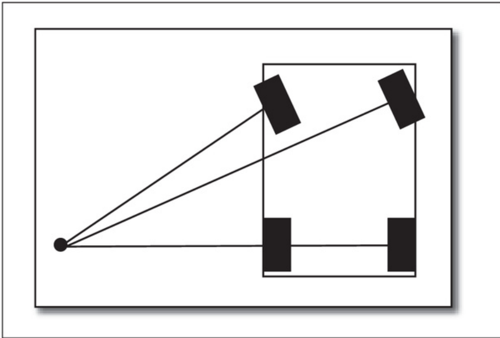
Figura 15. Arquitectura de un robot con control de ruedas Ackerman.
