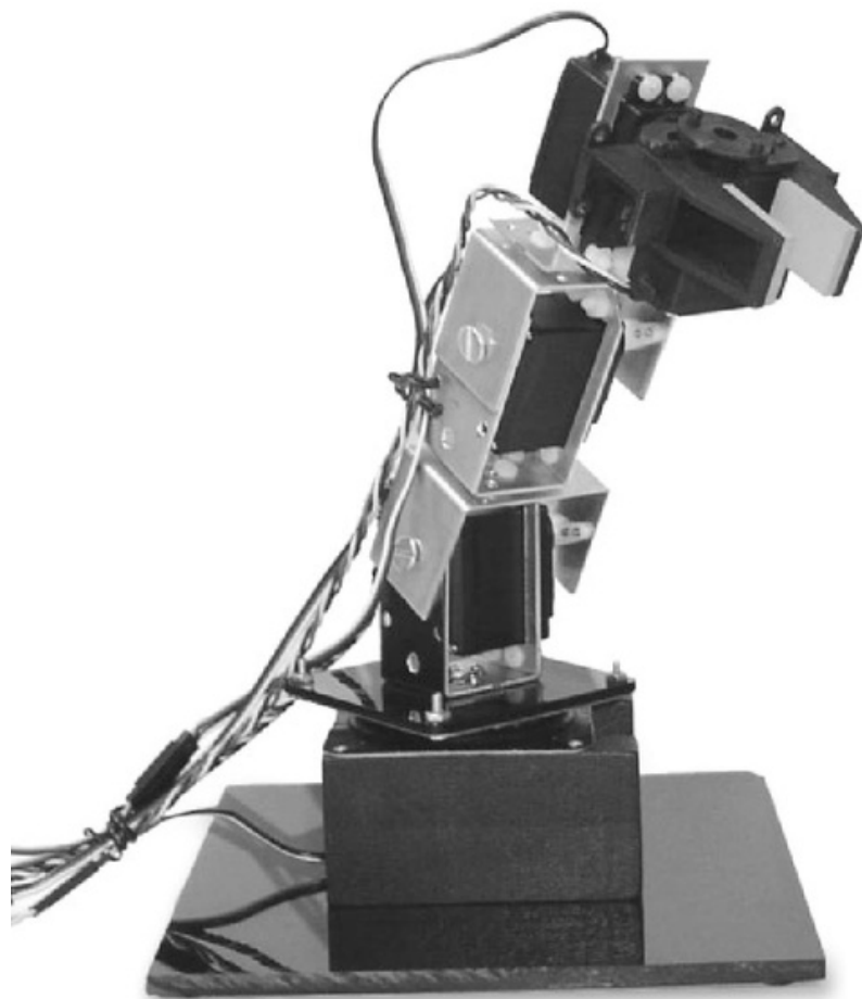
Figura 5. Kit de brazo robótico RA-01 con 5 servos.
