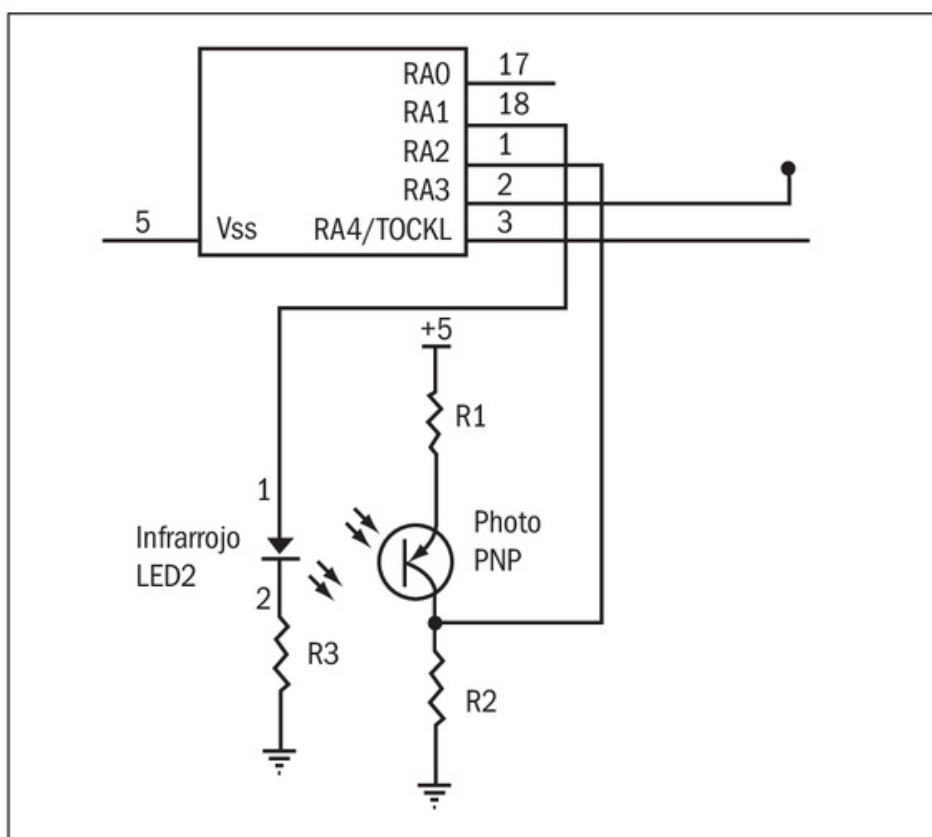
Figura 10. Circuito básico de conexión del infrarrojo a nuestro controlador.
