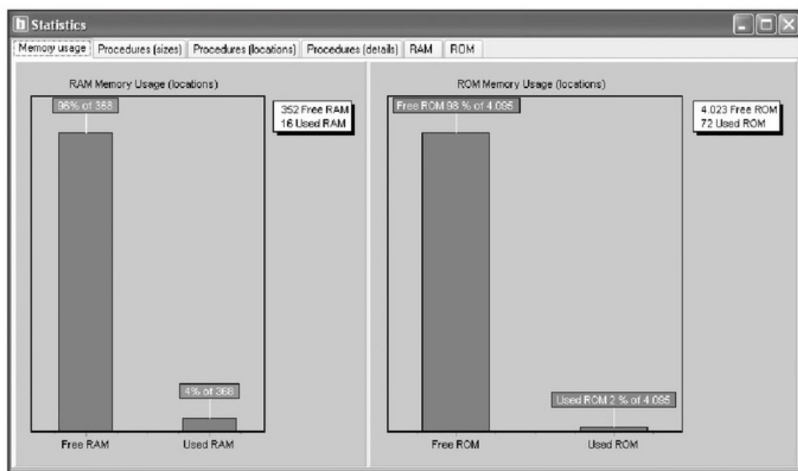
Figura 16. MikroBasic nos brinda magníficos gráficos estadísticos sobre el código de máquina que genera nuestro fuente.
