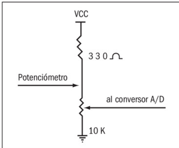
Figura 15. Conexión del potenciómetro a nuestro controlador.
