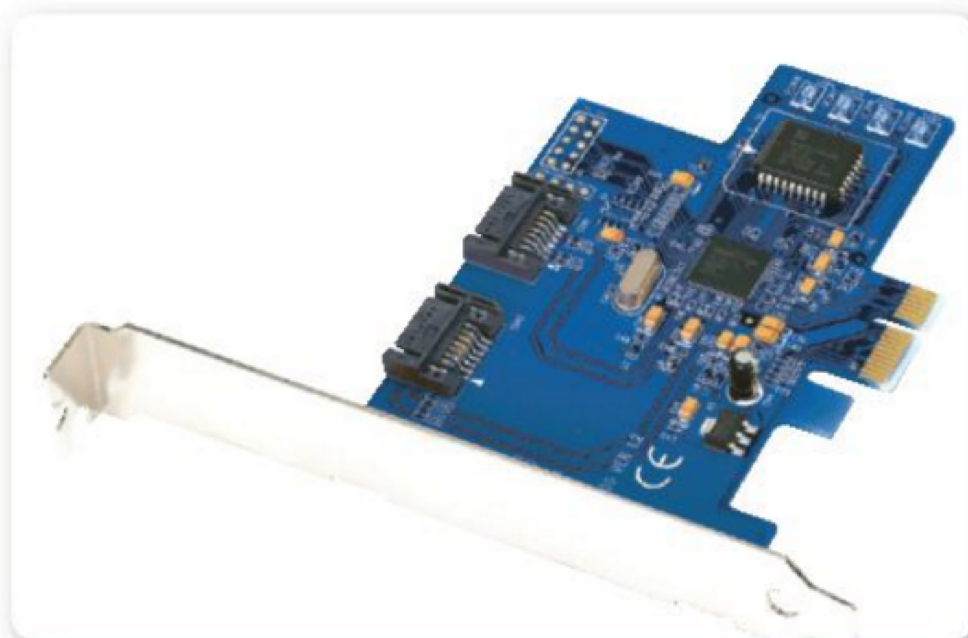
Figura 1. Controladora S-ATA. Si la interfaz de discos incorporada en el motherboard se daña, es posible reemplazarla por una placa.
