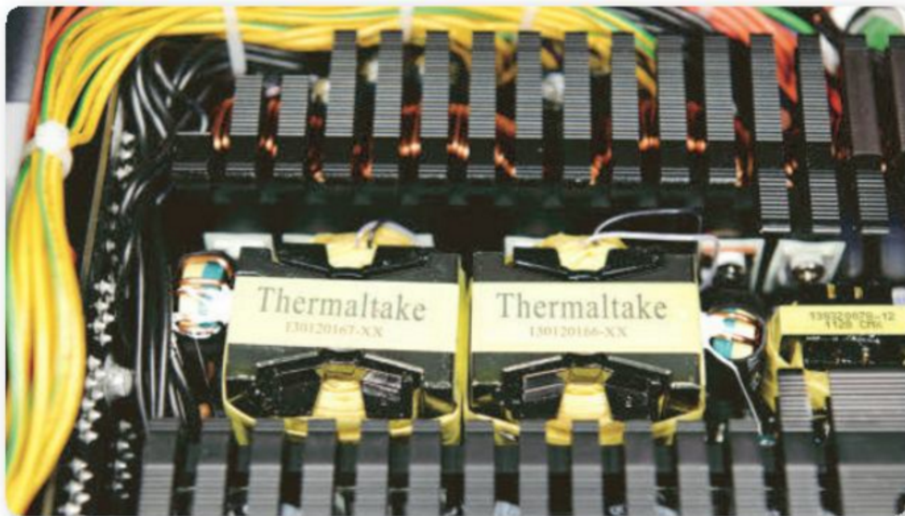
Figura 2. Los transformadores son los encargados de llevar la tensión de la red a los distintos valores de tensión necesarios.
