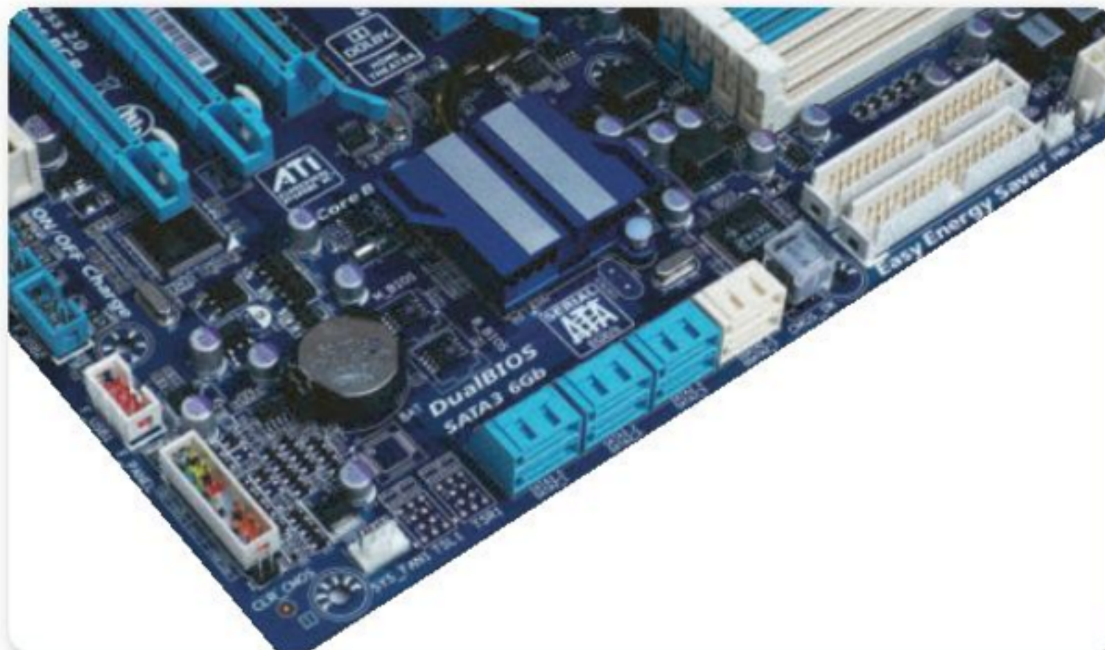
Figura 14. Algunos modelos de mothers instalan un segundo chip del BIOS por seguridad.
