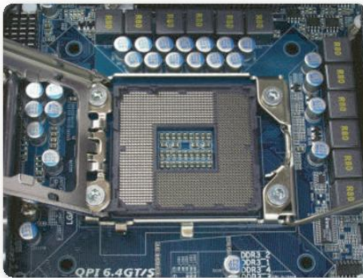
Figura 8. Este zócalo debe su nombre a que cuenta con 1366 superficies conductoras LGA que están incorporadas en el socket.
