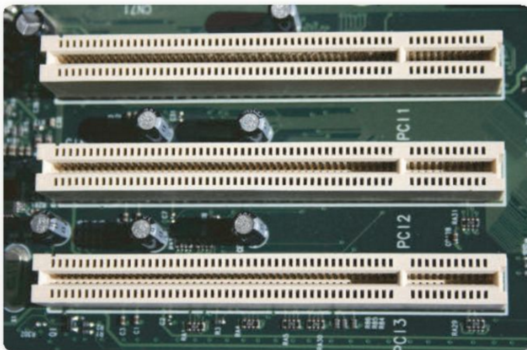
Figura 13. El zócalo PCI es considerado una ranura de cuarta generación, hoy remplazado por el PCI Express.
