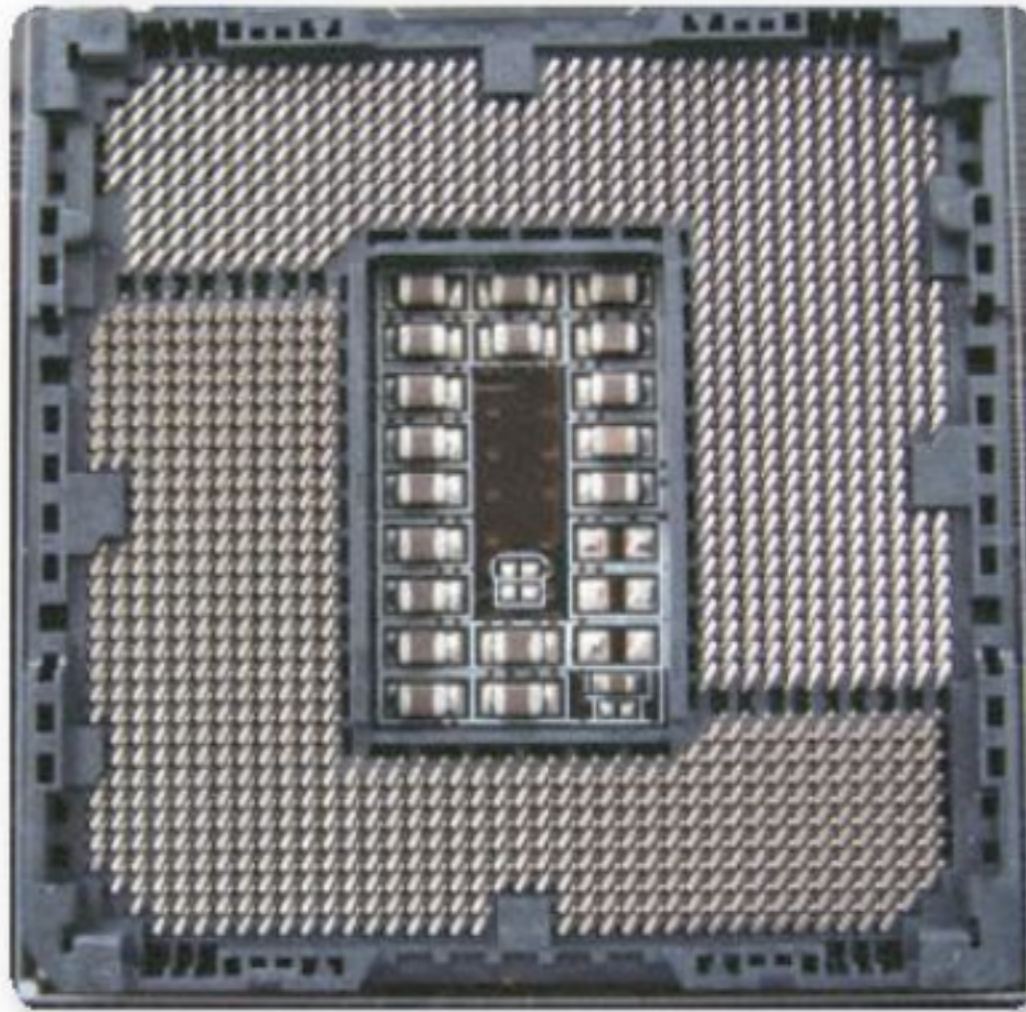
Figura 9. El zócalo LGA 1155 fue diseñado como un reemplazo al zócalo LGA 1156.
