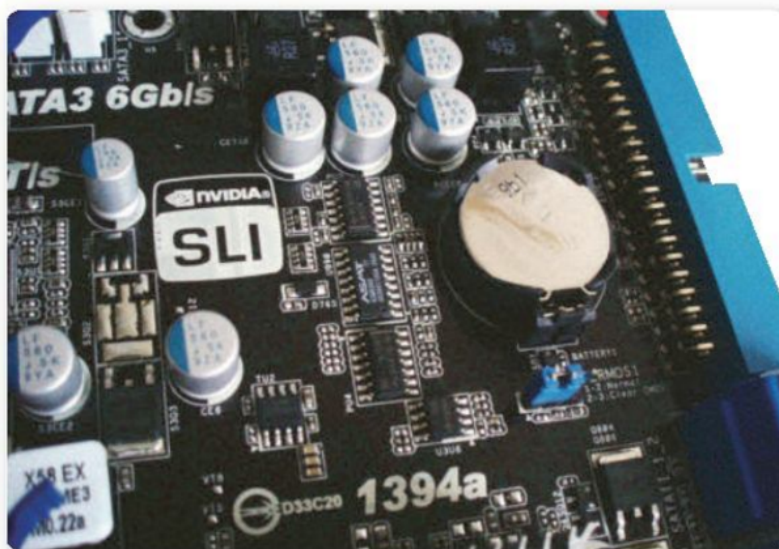
Figura 17. Mediante el jumpeo adecuado, podemos volver a valores de fábrica.
