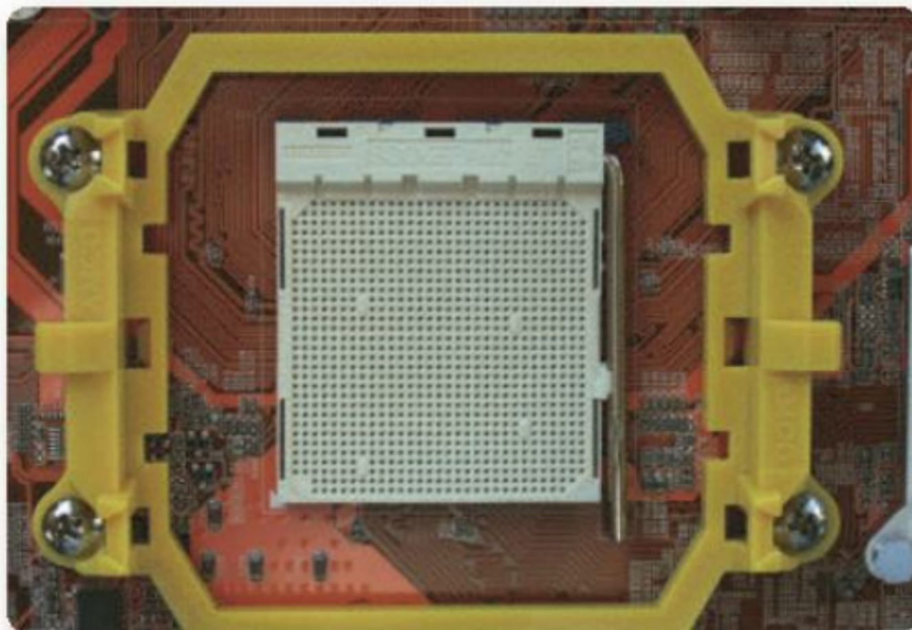
Figura 10. El AM2 es un zócalo de CPU diseñado para procesadores AMD.
