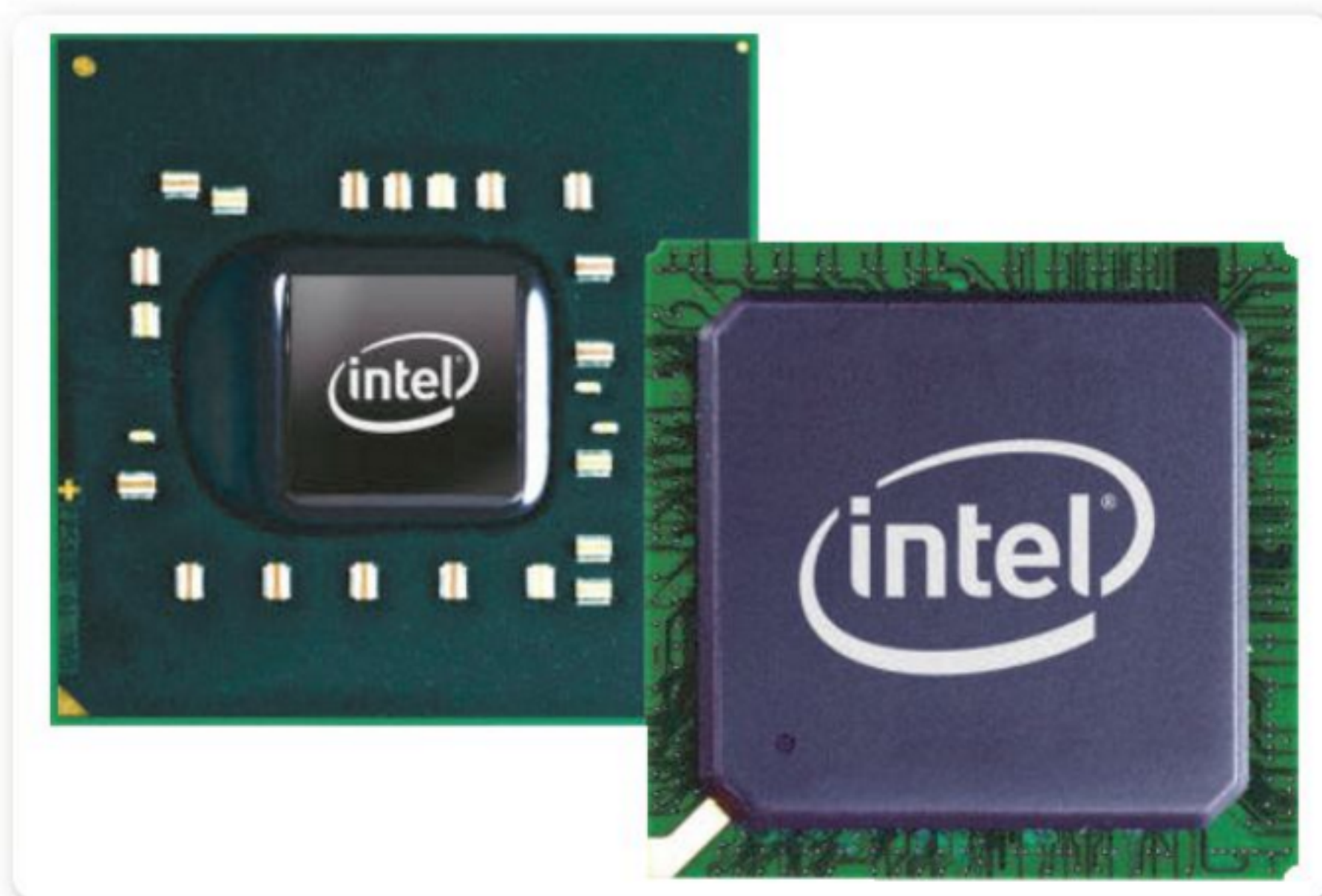
Figura 5. Típico chipset de Intel sin disipador de calor. El de arriba es el northbridge, y el de abajo, el southbridge.
