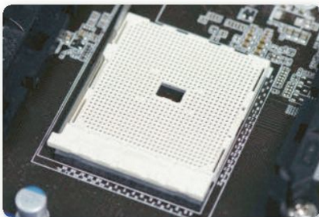
Figura 12. El zócalo FM2 fue lanzado en 2012 y es uno de los más usados por AMD.
