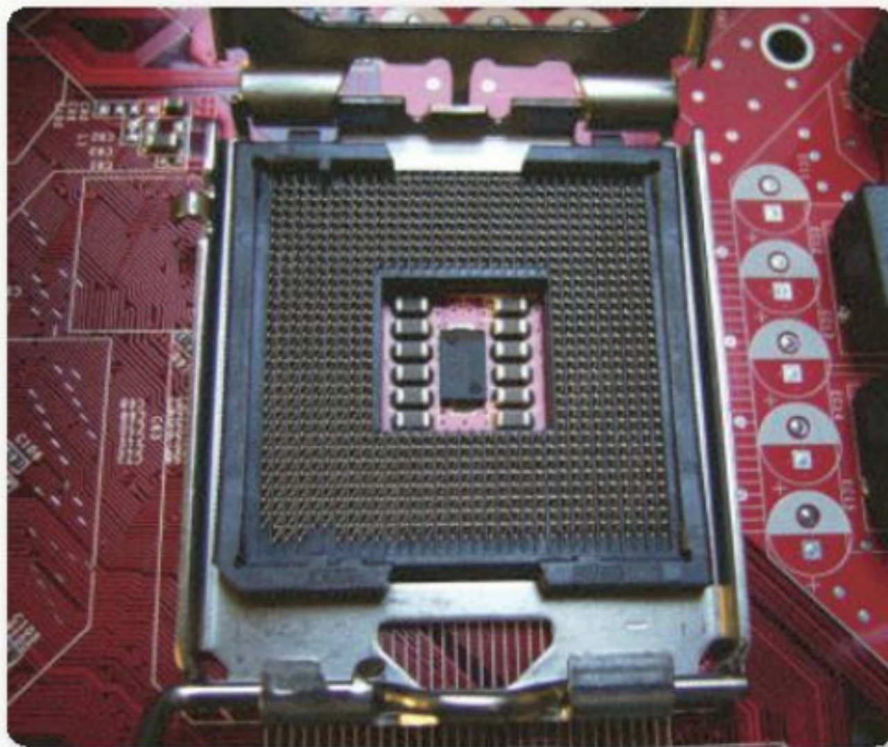
Figura 3. En los zócalos LGA, los contactos no están en la CPU, sino en el motherboard, para que no se doblen al manipular el chip.
