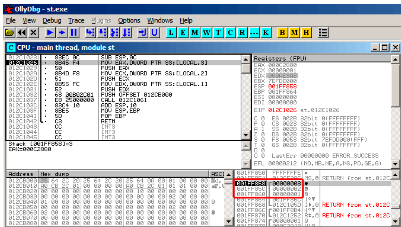
Figure 1.7: OllyDbg: f2()
