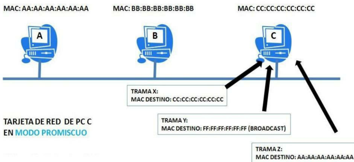
Figura 143 – NIC operando en modo promiscuo
