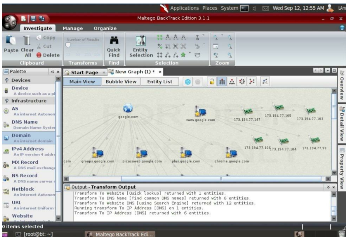
Figura 17 - Obtenemos las IP's asociadas a google.com
