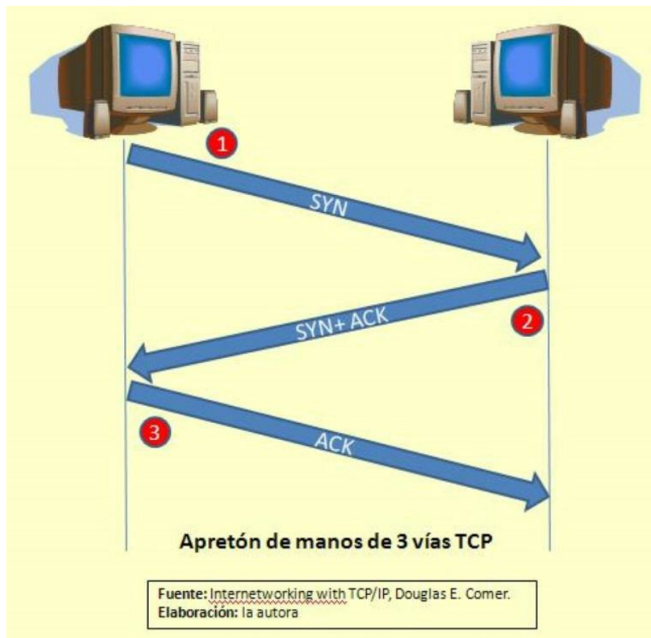
Figura 38 - Apretón de manos de 3 vías TCP
