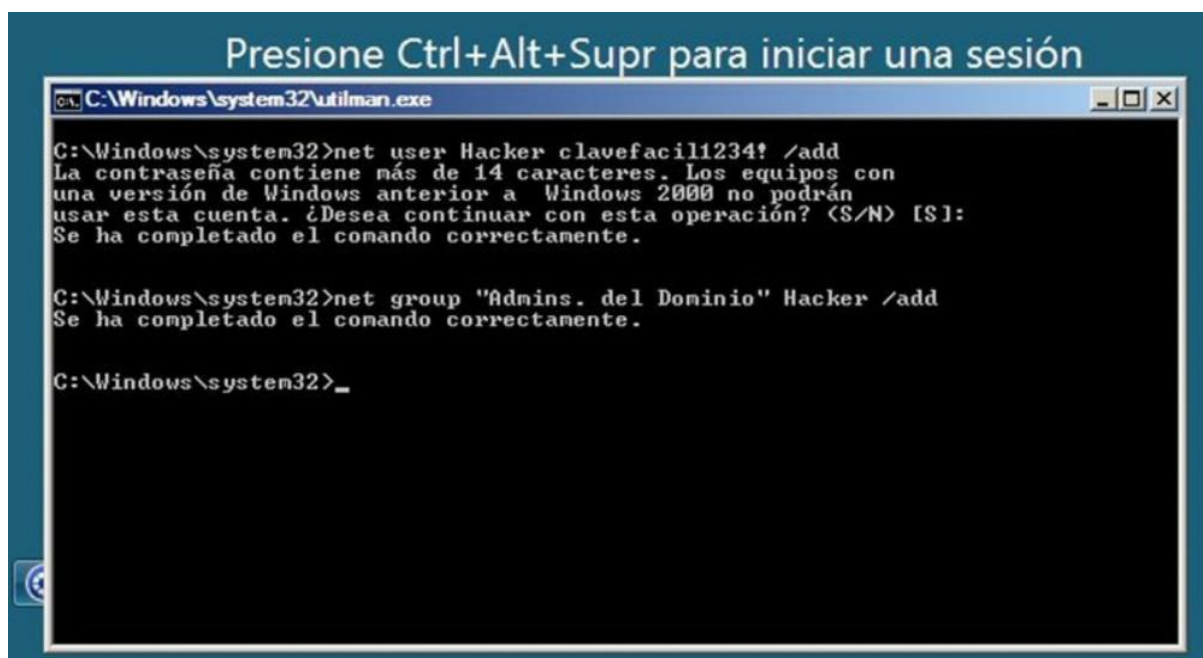
Figura 156 - Agregamos un usuario con privilegios administrativos
