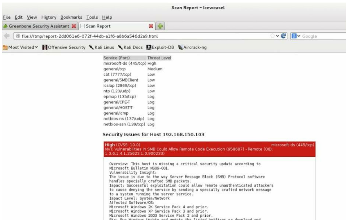
Figura 63 - GSA reporte en HTML
