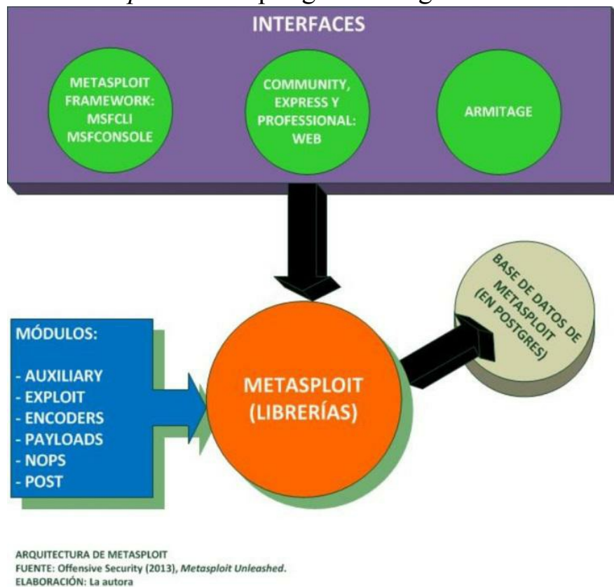
Figura 82 - Arquitectura de Metasploit
