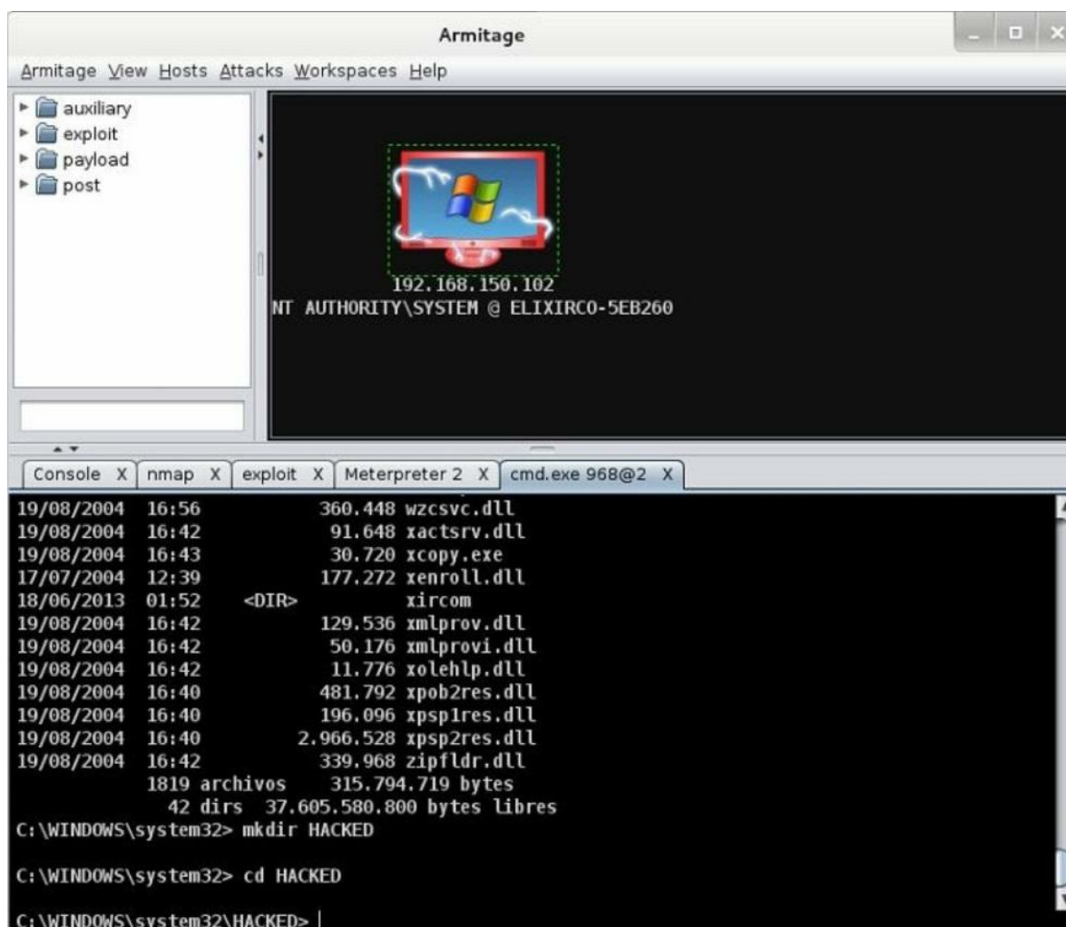
Figura 138 - Ejecución de shell DOS en host remoto
