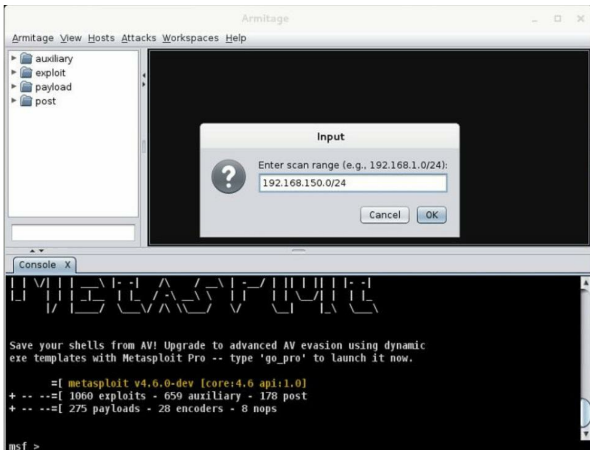
Figura 185 - Escaneo de la subred objetivo
