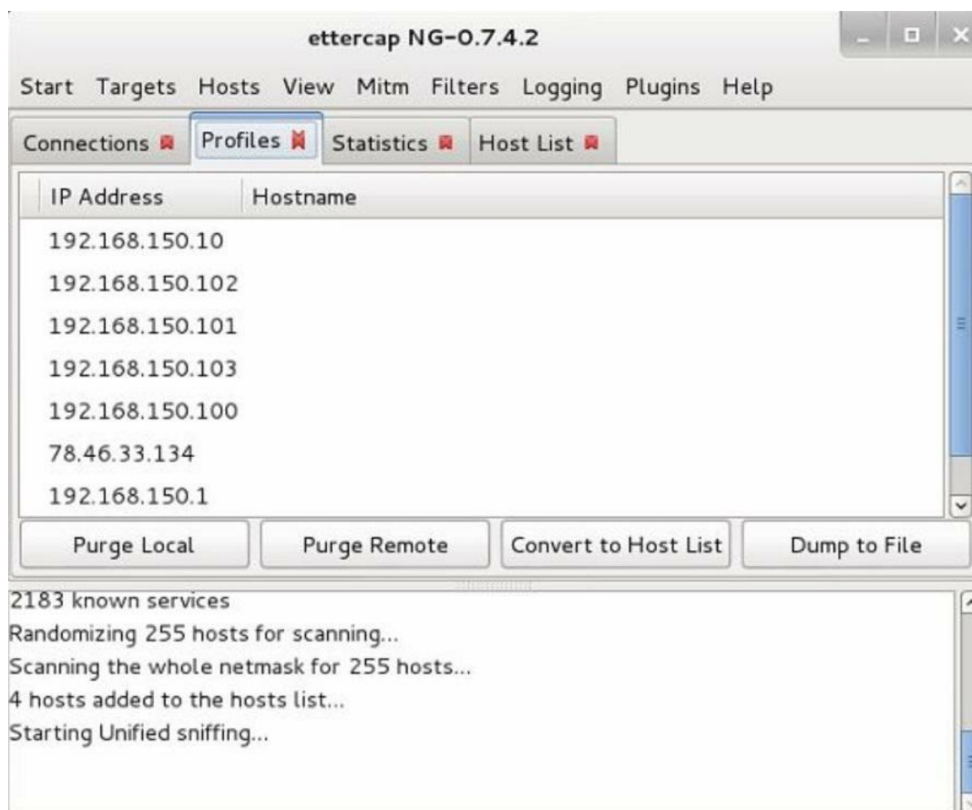
Figura 166 - Perfiles recolectados con ettercap
