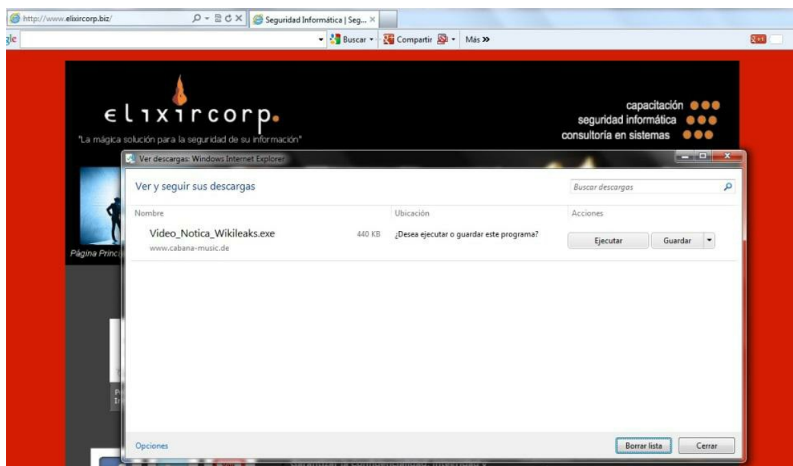
Figura 34 - Al hacer click sobre el enlace, se descarga un archivo malicioso en nuestro PC
