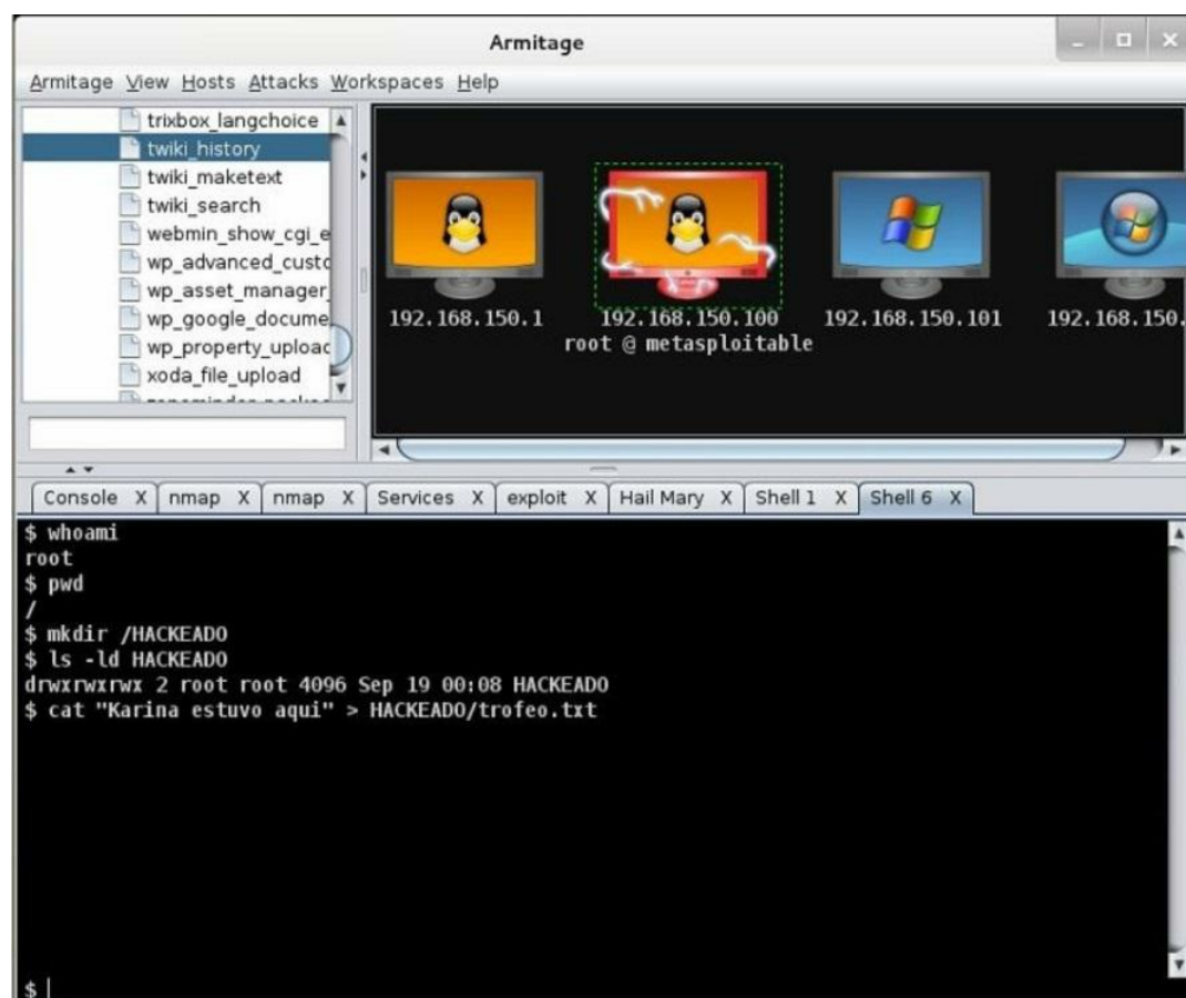
Figura 192 - Dejamos un trofeo en el host víctima
