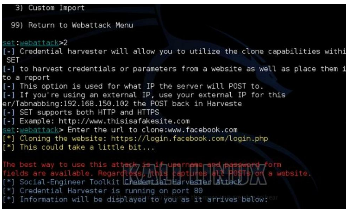
Figura 170 - Sitio web réplica operativo y a la espera de capturar credenciales
