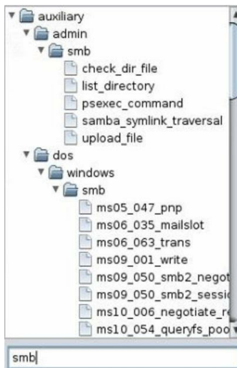
Figura 140 – Módulos que contienen el término "smb"
