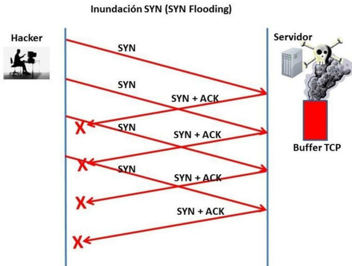
Figura 150 - DoS mediante inundación SYN
