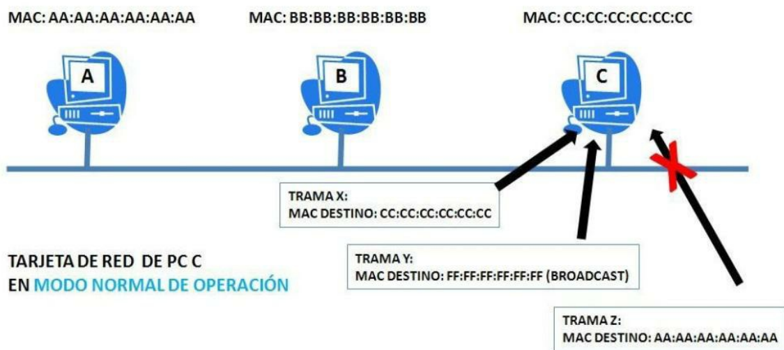
Figura 142 - Modo normal de operación de una tarjeta de red (NIC)
