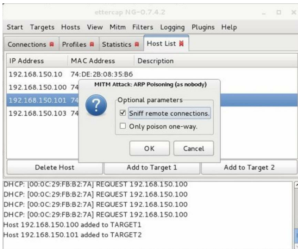
Figura 167 - ARP poisoning con ettercap
