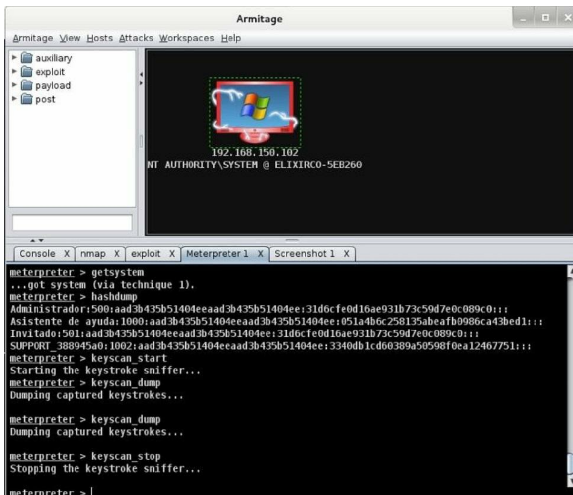
Figura 137 - Elevación de privilegios, dump de la SAM y keylogger
