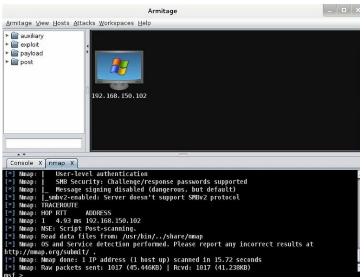
Figura 131 - Host agregado al workspace default
