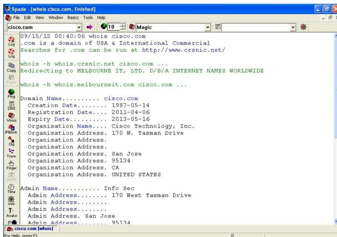
Figura 28 - Consulta sobre dominio en Sam Spade
