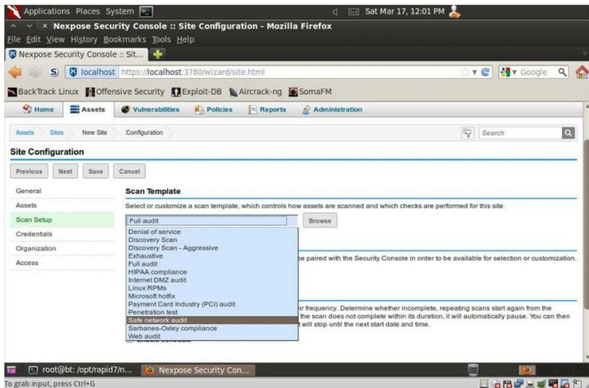
Figura 50 - Seleccionando la plantilla de escaneo
