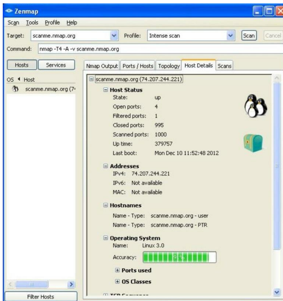
Figura 41 - Detección de sistema operativo
