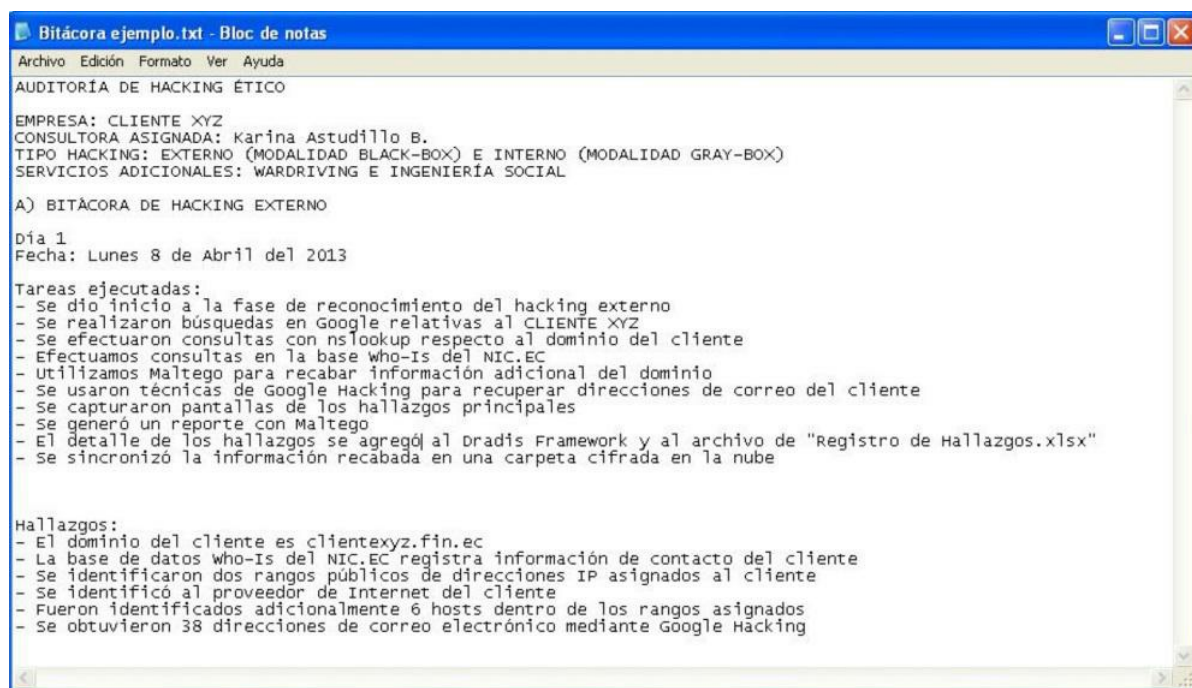
Figura 194 - Bitácora ejemplo
