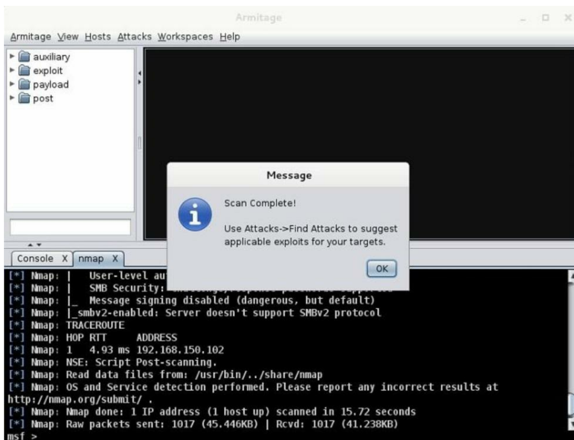
Figura 130 - Escaneo finalizado
