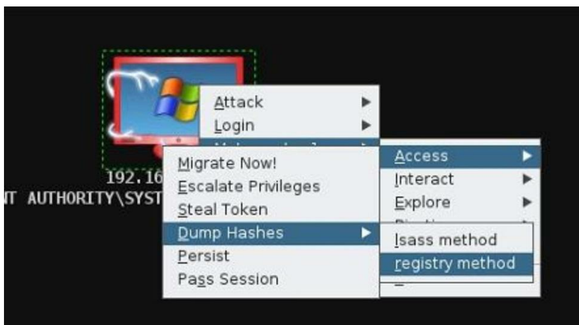
Figura 141 - Obtención de hashes vía meterpreter usando el menú contextual
