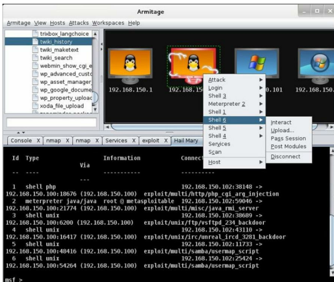
Figura 191 - Host Linux comprometido y sesiones remotas abiertas
