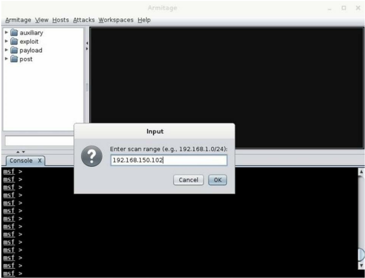
Figura 129 - Escaneo con Nmap desde Armitage
