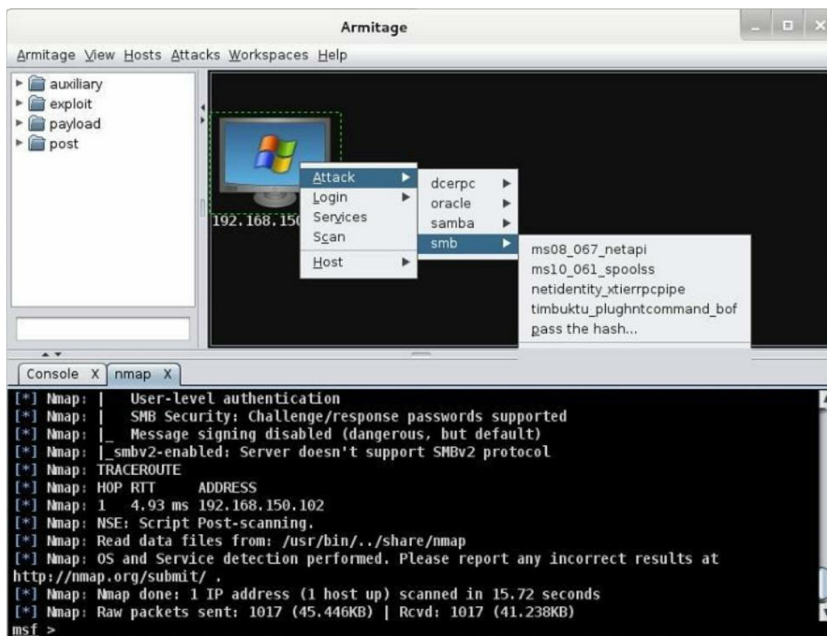
Figura 132 - Menú contextual Attack agregado para el host víctima
