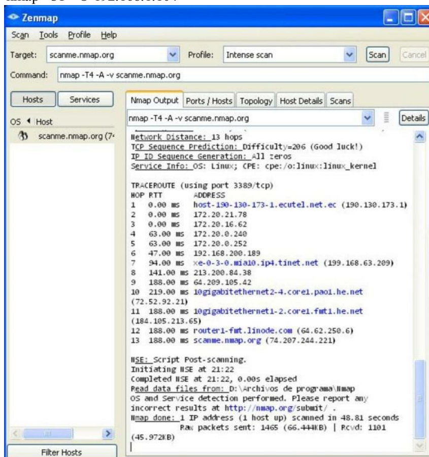
Figura 39 - Interfaz gráfica Zenmap, escaneo intensivo a scanme.nmap.org
