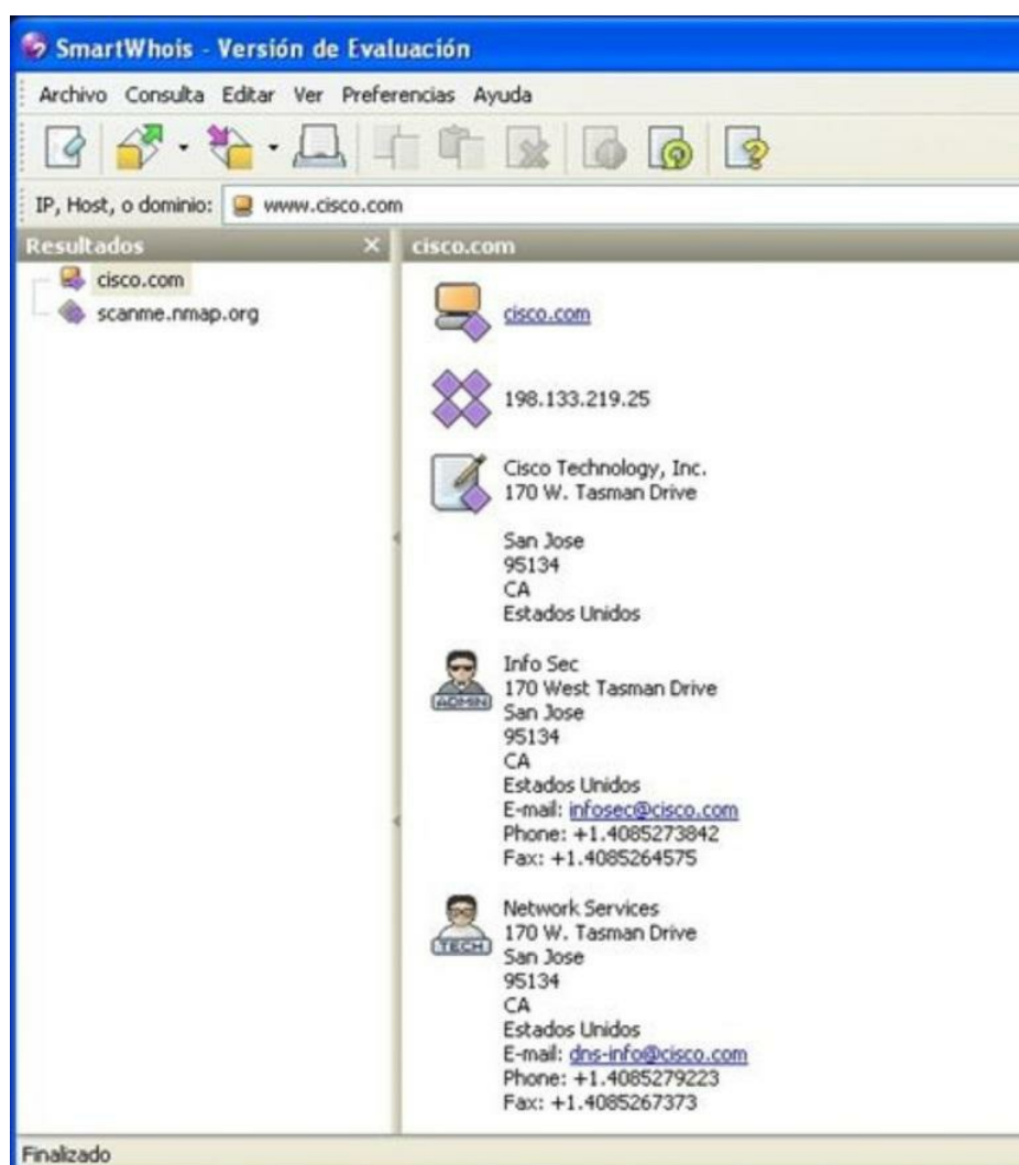
Figura 26 - Resultados de consultar el dominio cisco.com
