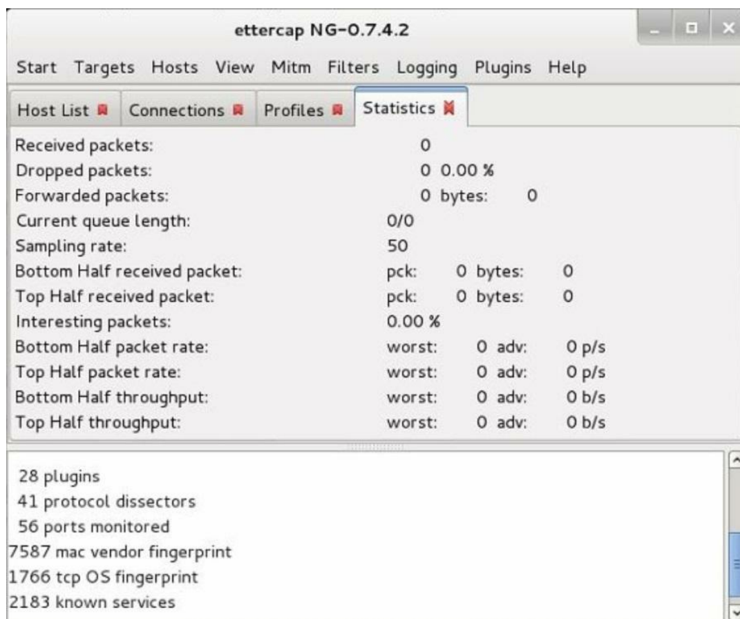
Figura 165 - Viñetas adicionales en ettercap
