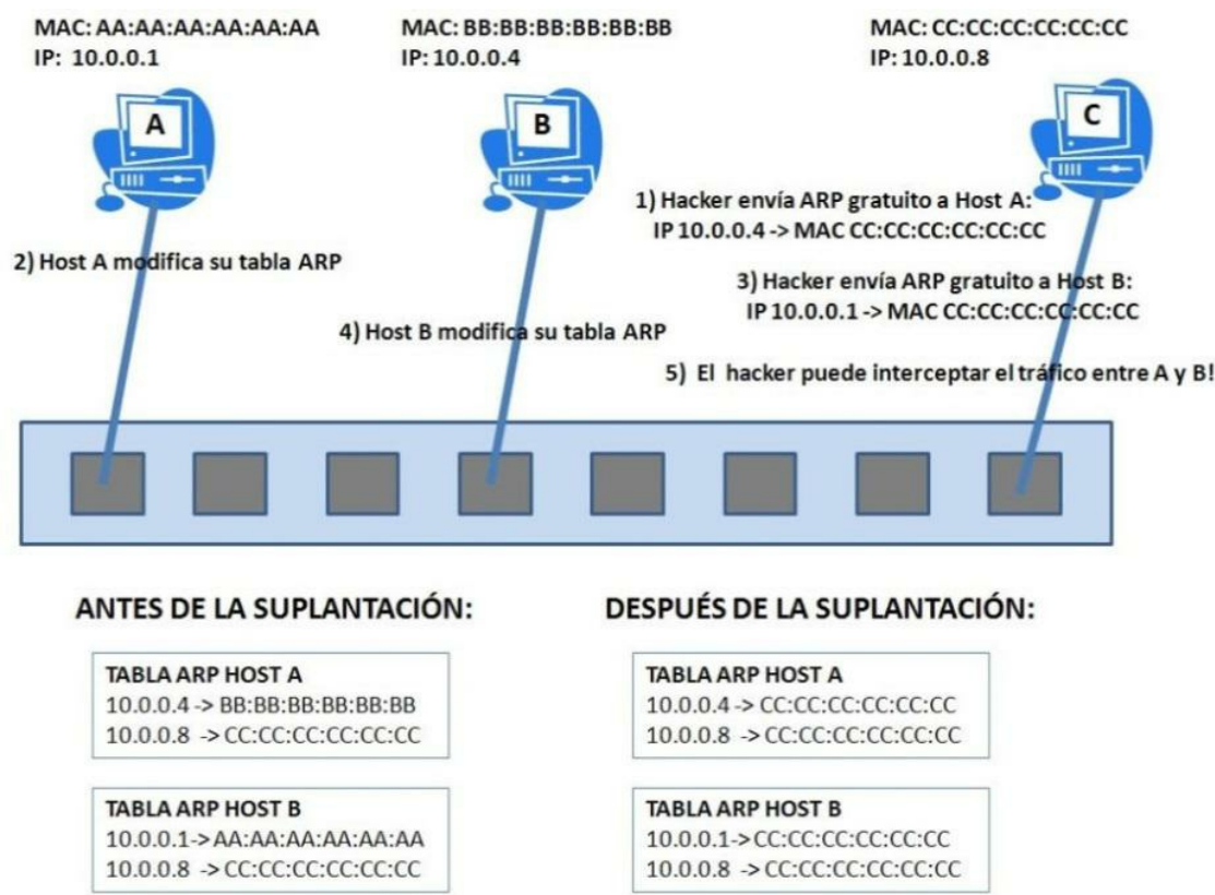
Figura 146 - Ataque MITM a través de suplantación ARP (spoofing)
