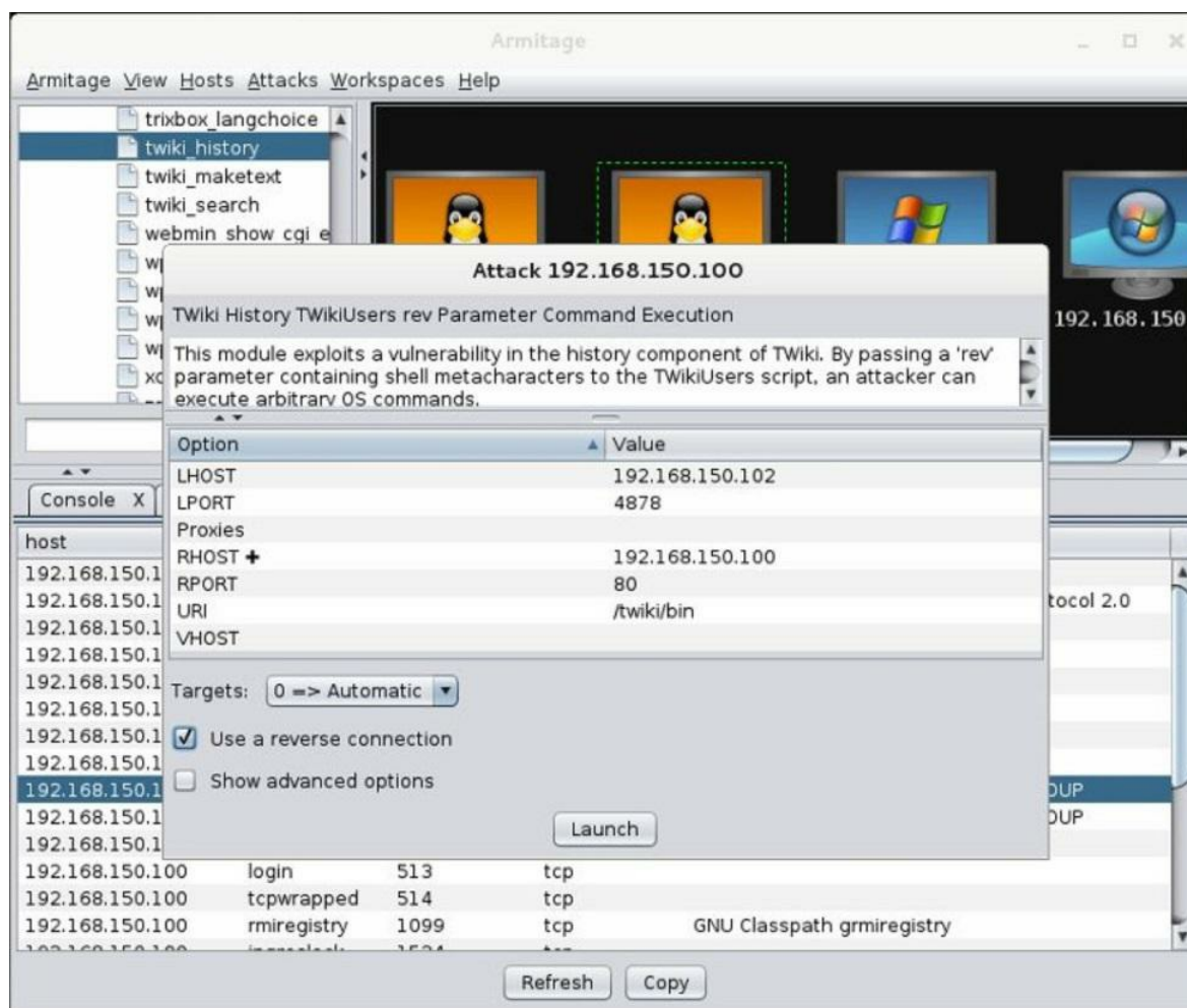
Figura 189 - Ejecución de exploit manualmente
