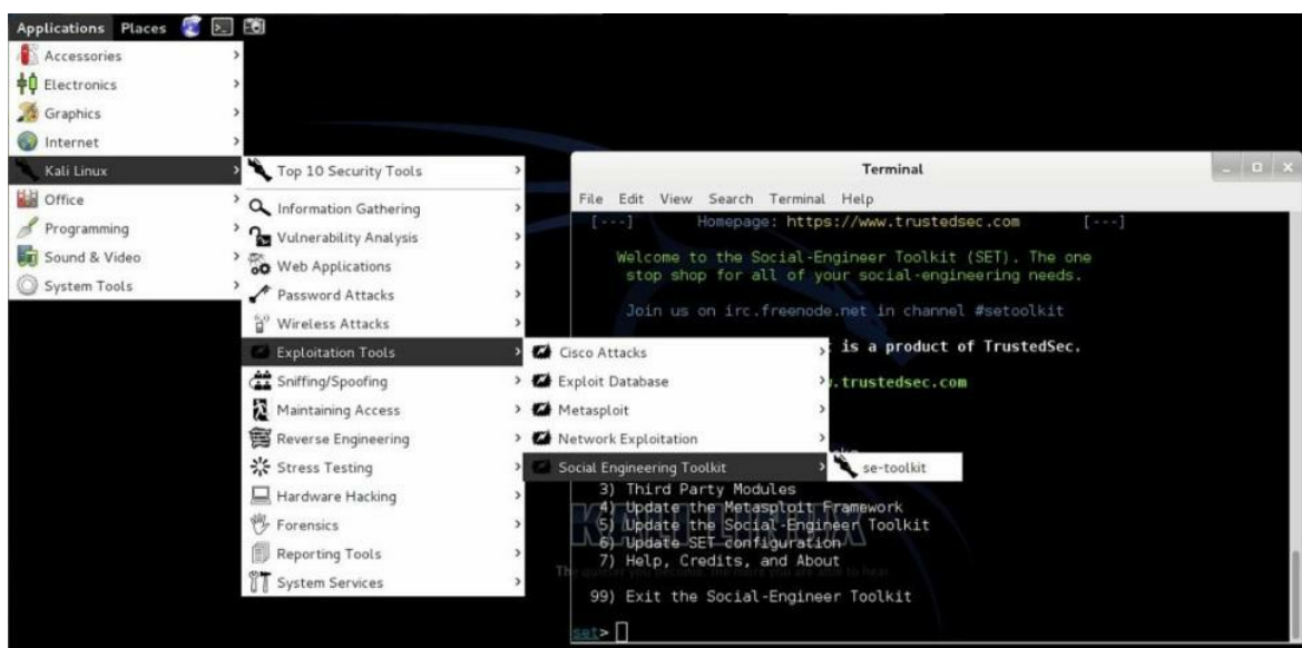
Figura 169 - Ejecutamos SET
