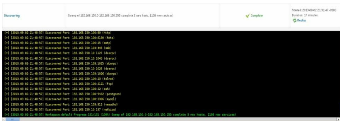
Figura 121 - Escaneo completado
