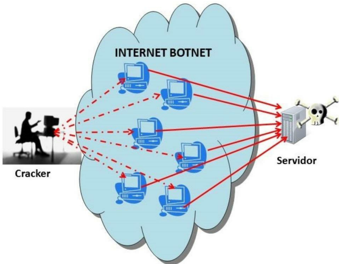
Figura 149 - Ataque DDoS
