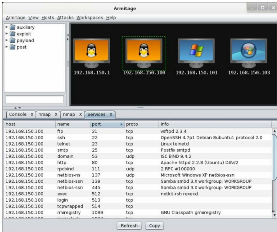
Figura 186 - Servicios activos en el host Linux víctima
