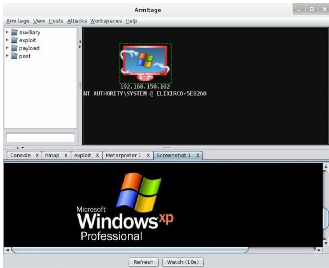
Figura 136 - Captura de pantalla con el comando screenshot de meterpreter
