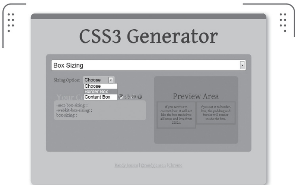
► Figura 28. La propiedad box-sizing puede manejarse con gran facilidad mediante la aplicación online CSS3 Generator.
