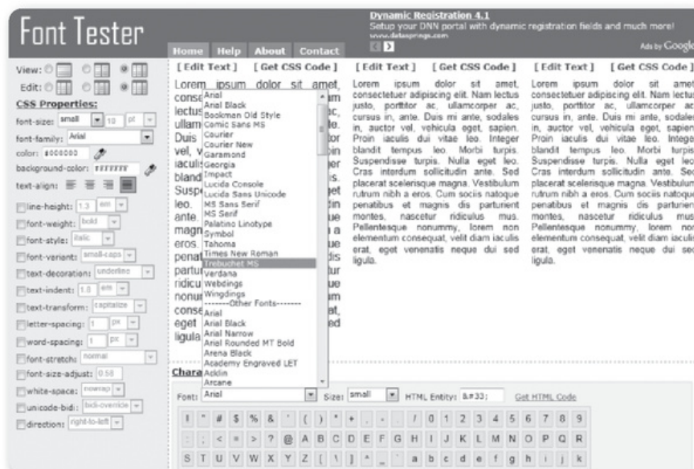
► Figura 6. Font Tester (www.fonttester.com) es una herramienta online muy completa para probar estilos de fuentes y nos ofrece la posibilidad de obtener el código CSS de los estilos que creamos.
