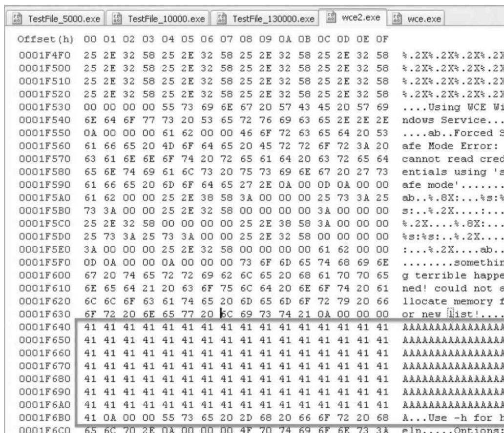
Figure 130 - Modifying the Signature to Evade AV
