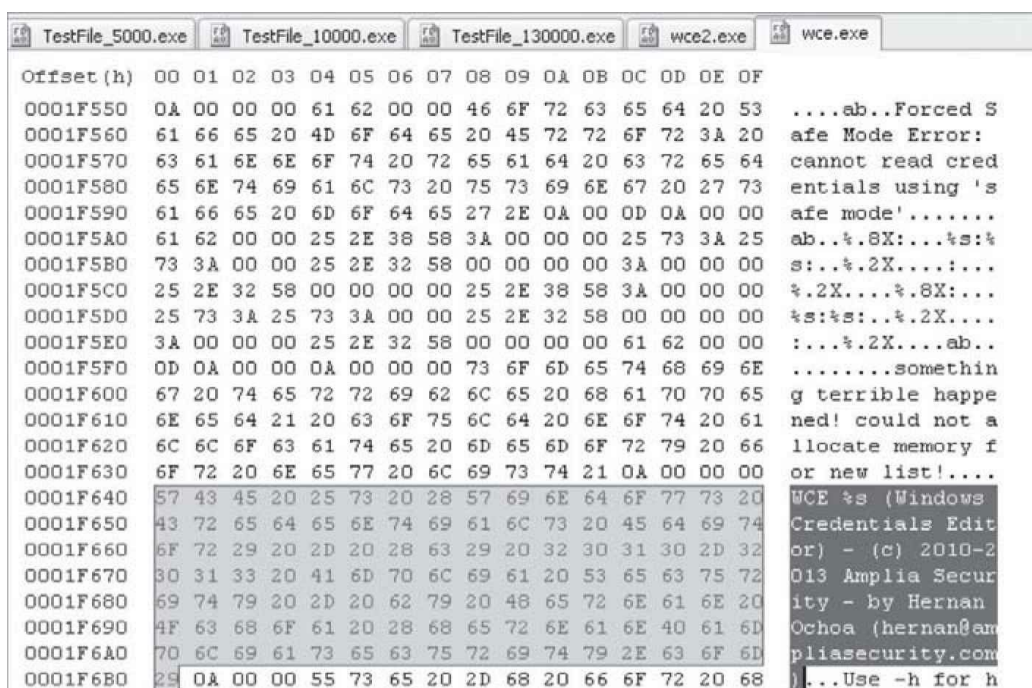
Figure 129 - Identifying the String that Triggers AV
