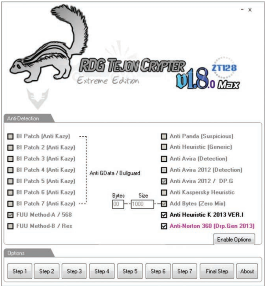
FIGURE 9.9 Tejon Crypter
